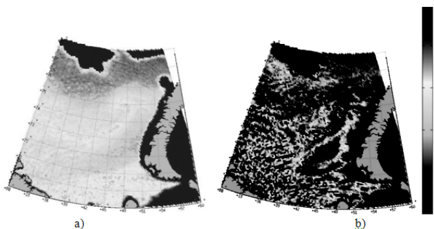
Рис. 4 Поле водяного пара, \text{кг/м}^2 – а) и жидко-капельной влаги, \text{кг/м}^2 – б) полярного циклона над восточной частью Баренцево моря 18 января 2007 года 08:31-09:22 UTC по данным спутника Aqua прибора AMSR-E
