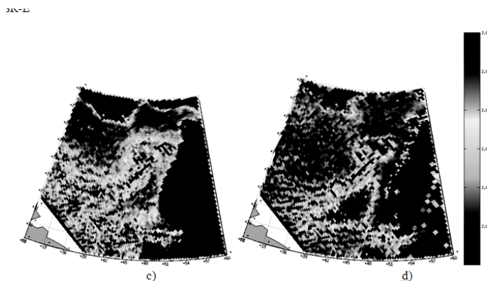
Рис. 5 Поле водяного пара, \text{кг}/\text{м}^2 – с) и жидко-капельная влага, \text{кг}/\text{м}^2 – d) полярного циклона над восточной частью Баренцево моря 18 января 2007 года по данным метеорологического спутника серии DMSP f-13 прибора SSM/I
