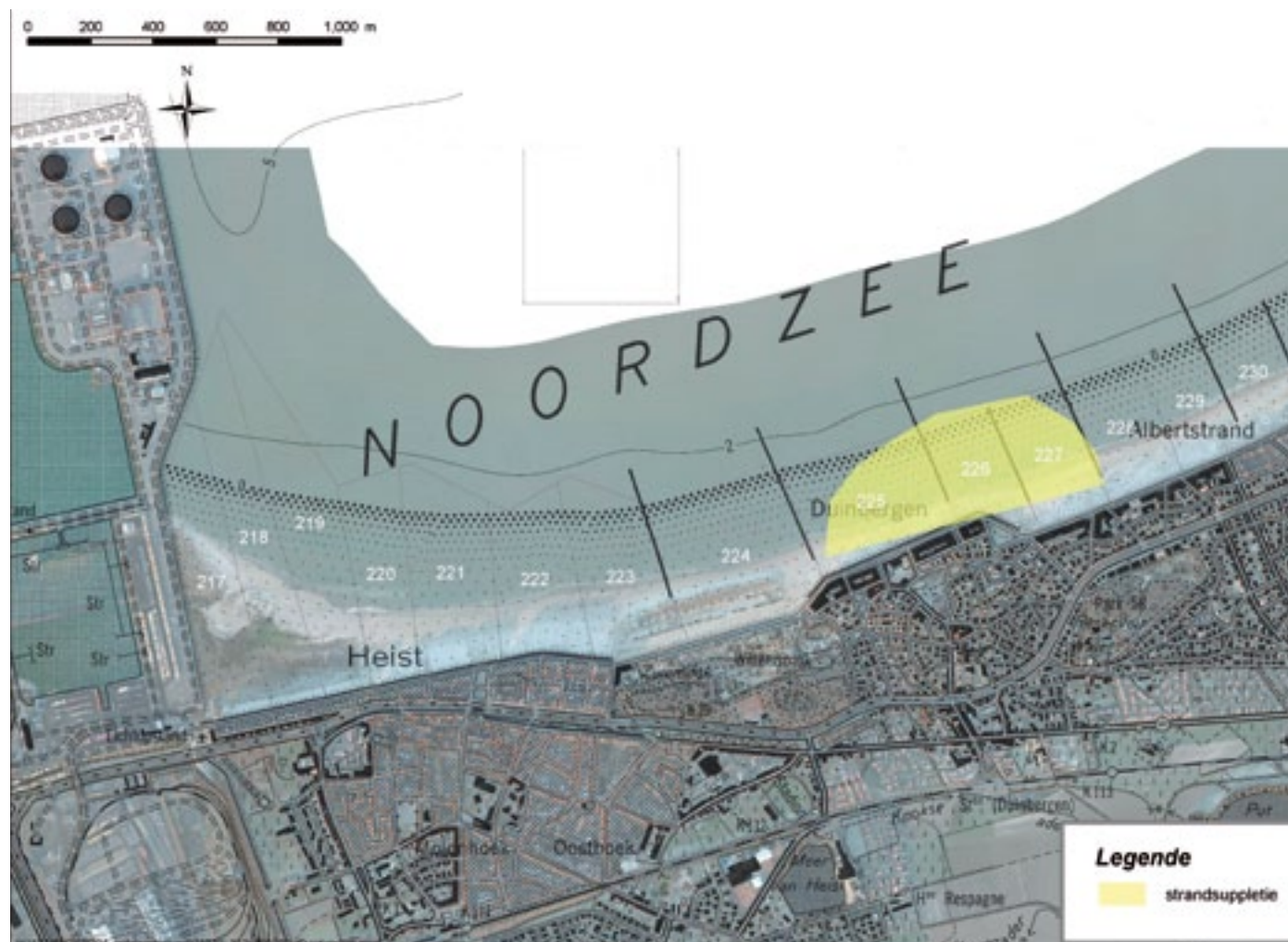
De locatie van de gekozen maatregelen in Knokke-Heist
