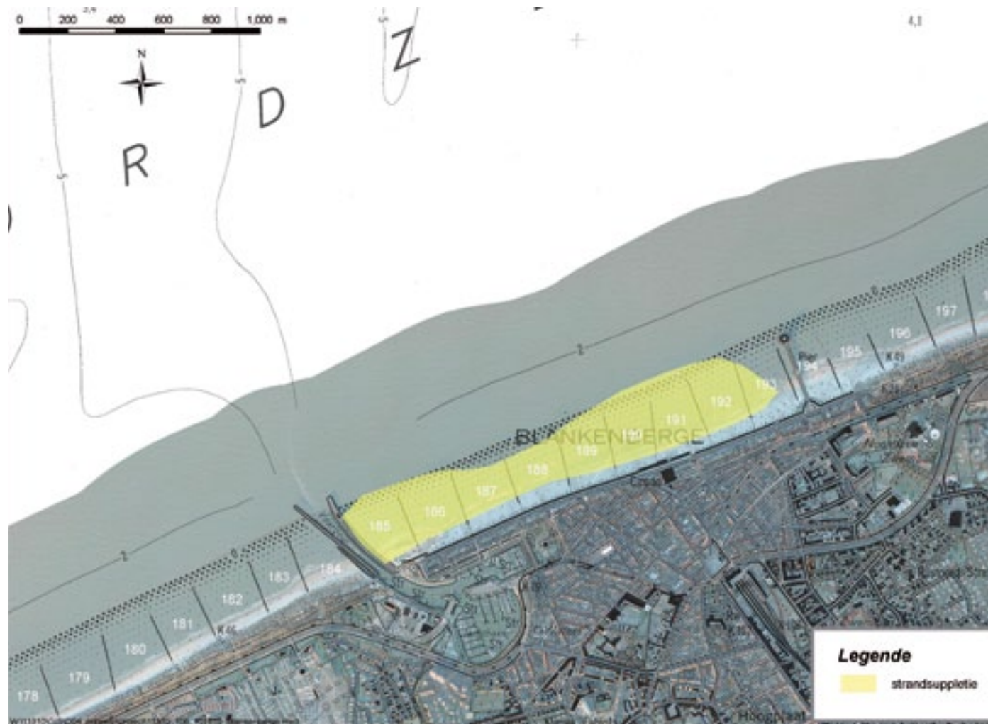
De locatie van de gekozen maatregelen in Blankenberge (sectie 185 tot 195)
