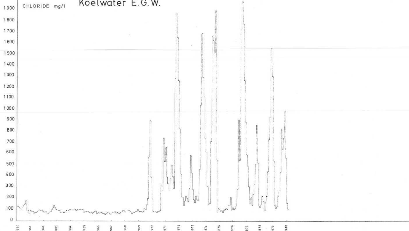
FIG. 7. — Evolutie van het chloridegehalte van het koelwater dat door de Elektriciteitscentrale van de stad Gent in het Handelsdok wordt opgepompt.
