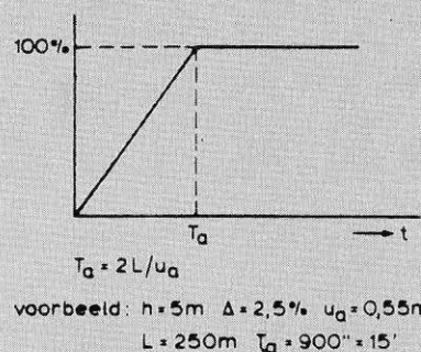
FIG. 15. — Het uitgewisselde volume met de tijd.
