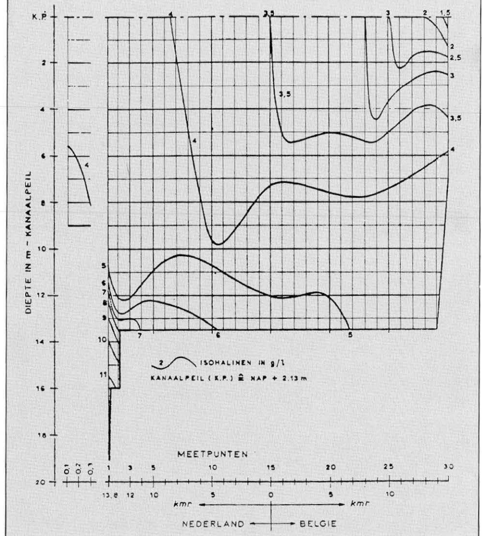
FIG. 9. — Isohalinen in g/l van het kanaal Gent-Terneuzen. Toestand op 29-12-1976.
