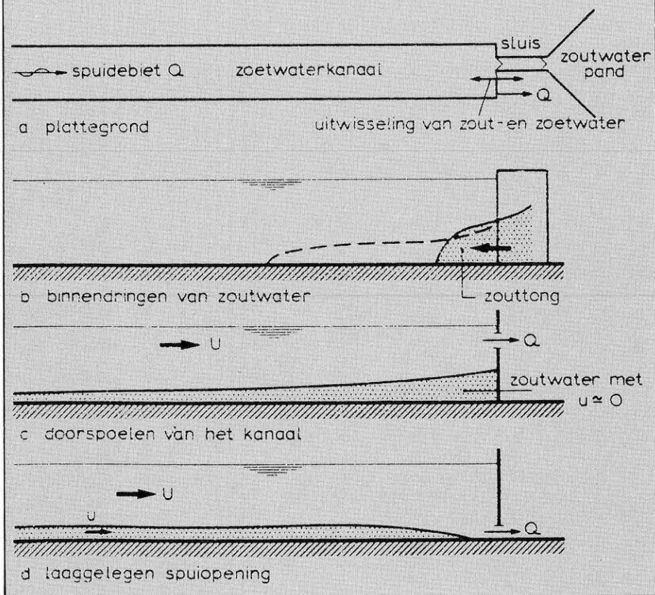
FIG. 13 — Situatie met normale zoutpenetratie.
