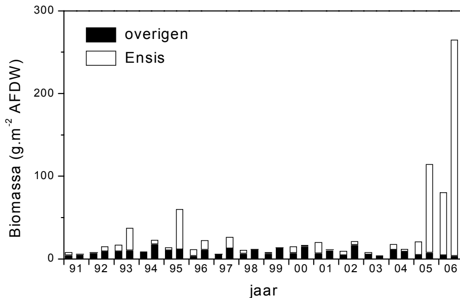
Figuur 2. Verloop van de biomassa van het macrozoöbenthos, en afzonderlijk dat van Ensis americanus , op raai J op het Balgzand tijdens de winter- en zomerbemonsteringen.
