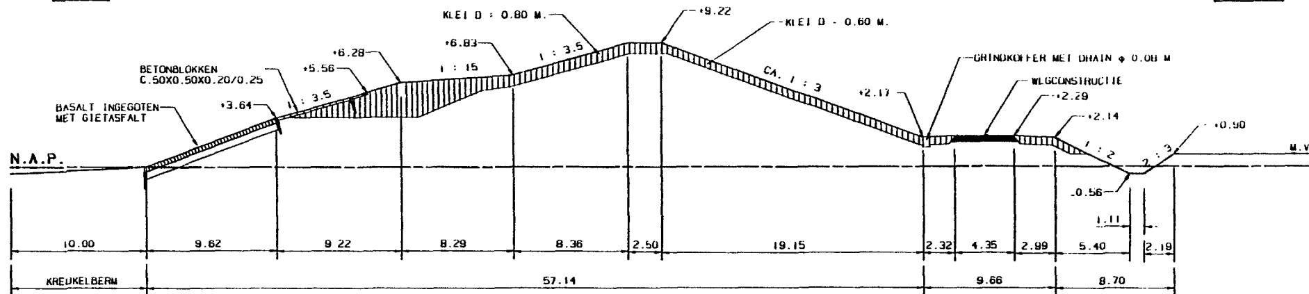
DWARSPROFIEL 2
