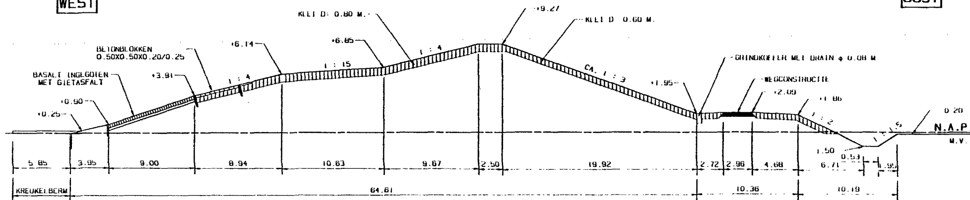
DWARSPROFIEL 1
