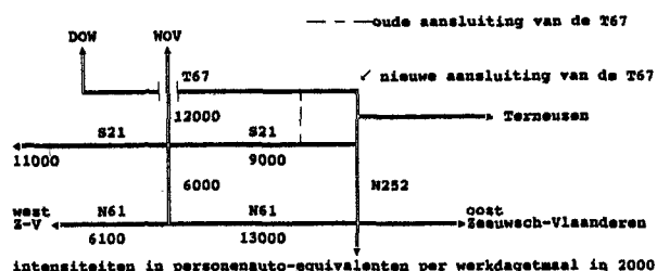
Figuur g. Schematische situatie aansluiting WOV in Zeeuwsch-Vlaanderen nabij DOW
