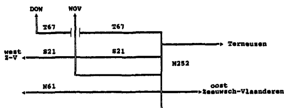
Figuur e. Schematische situatie aansluiting WOV in Zeeuwsch-Vlaanderen volgens variant D.
