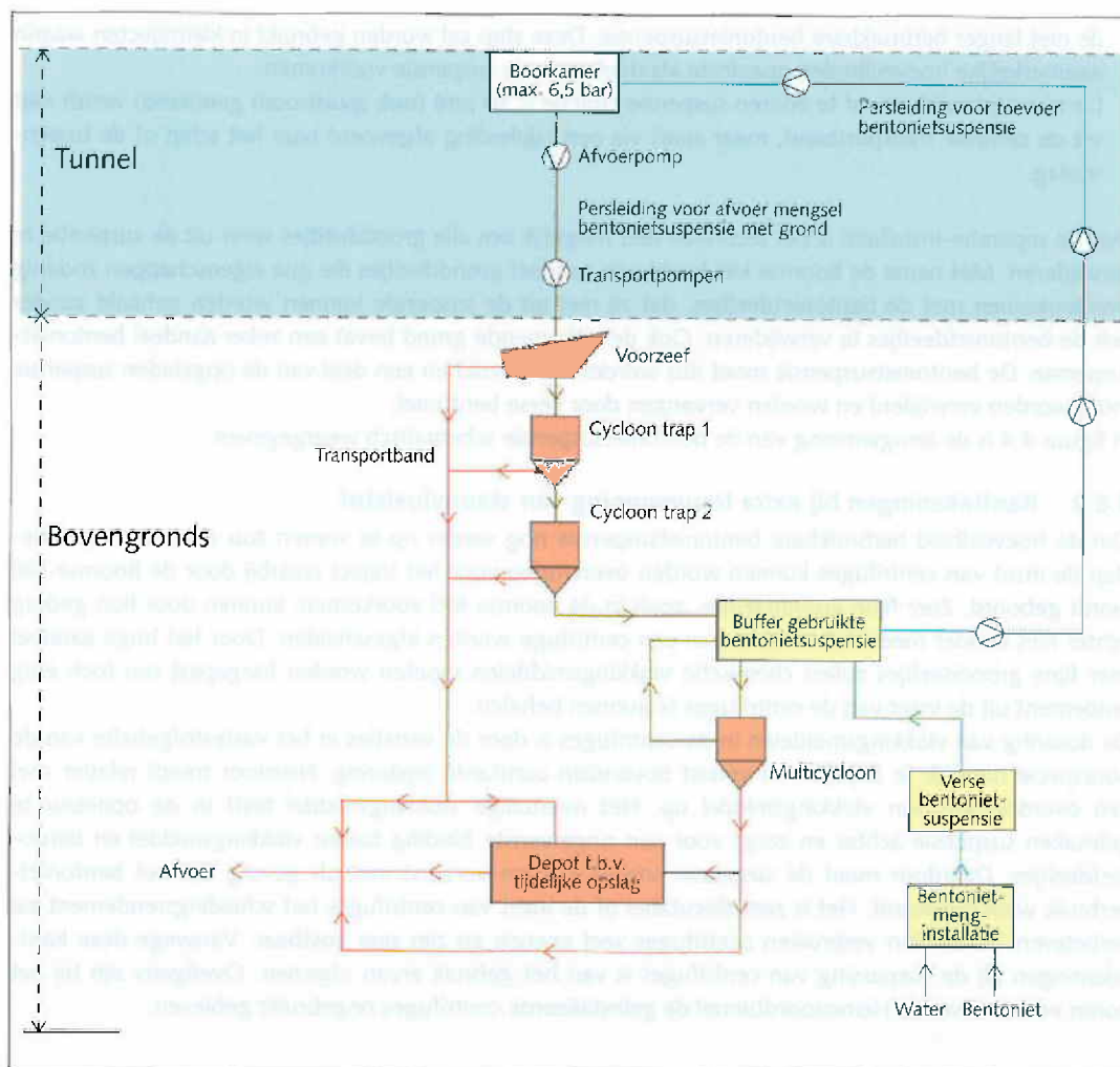
Figuur 4.4 Schematische weergave van de separatie installatie.
