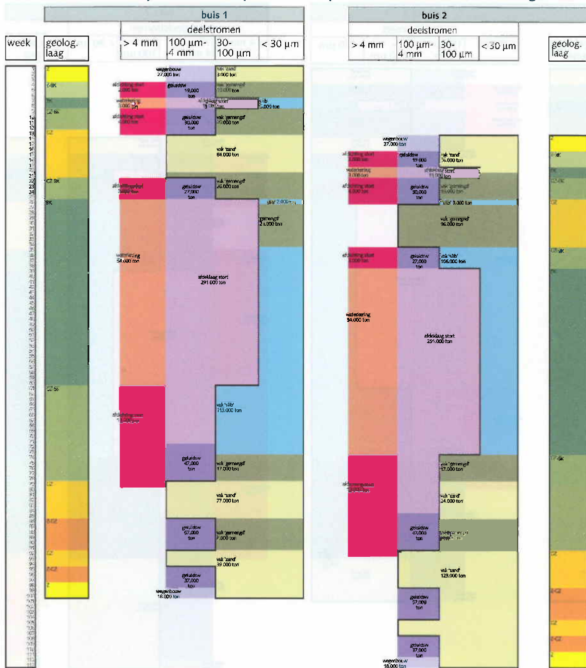
Afvoer van de vrijkomende boorspecie uit de separatie-installaties (in tonnen droge stof)
