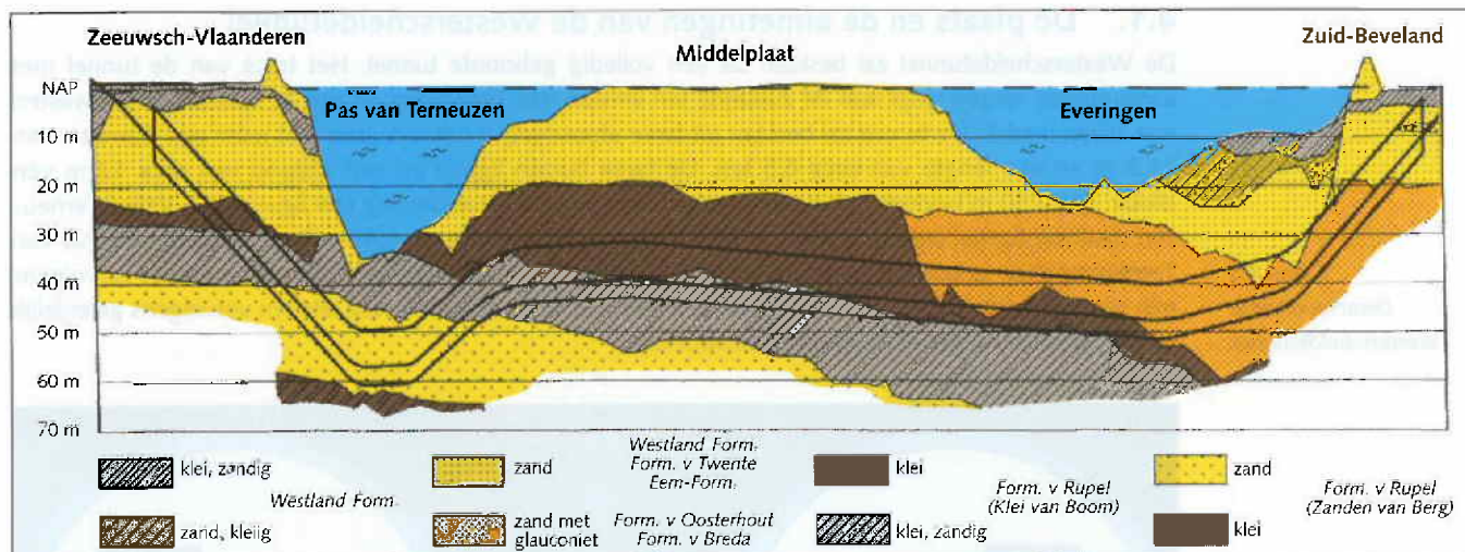
Figuur 4.2 Geologisch bodemprofiel ter plaatse van de Westerscheldetunnel.
