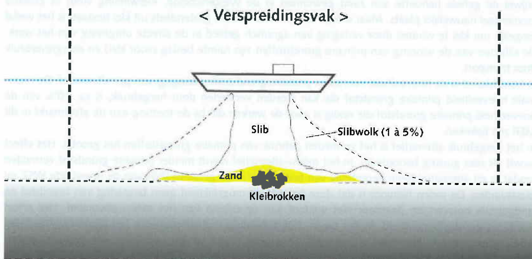
Figuur 9.1 Het verspreiden van specie met een onderlosser.
