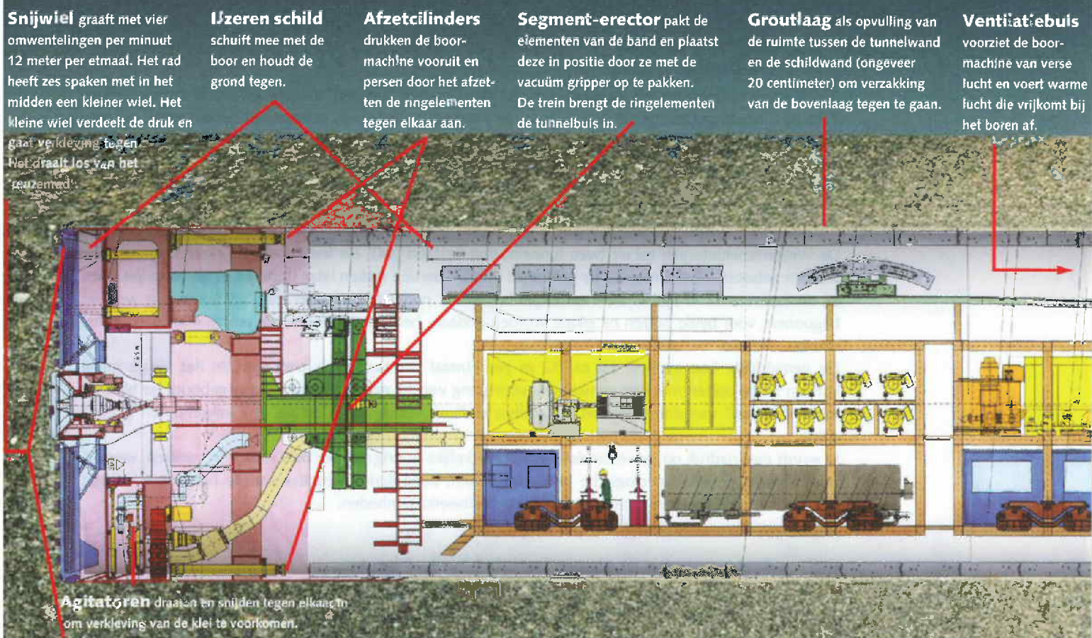
Figuur 4.3 De boormachine voor de Westerscheldetunnel zal een tunnel met een doorsnede van 11,3 meter boren.
