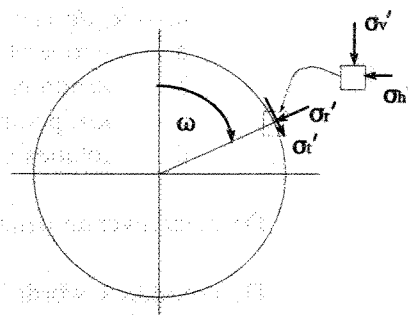
figuur 4.43 Toelichting poolcoördinaten
