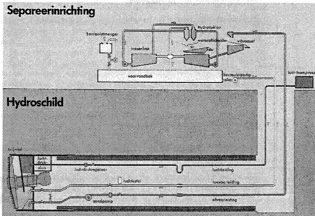
figuur 4.3 Grondscheidingsinstallatie
