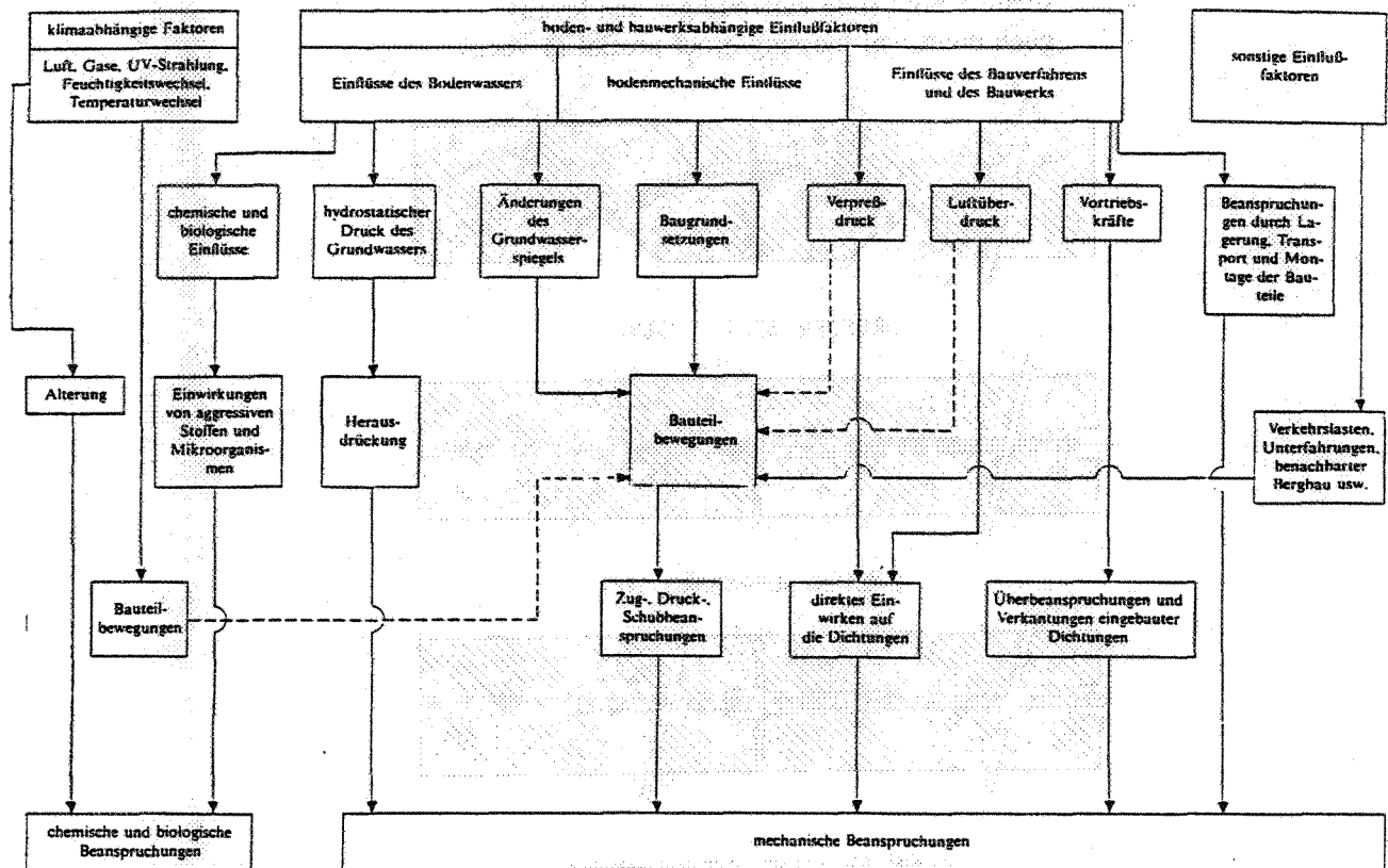
figuur 4.37 Invloedsfactoren op keuze afdichting
