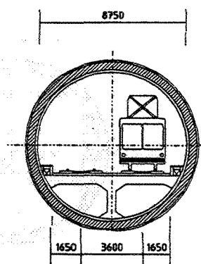
6. SNELTRAM, DUBBEL SPOOR
