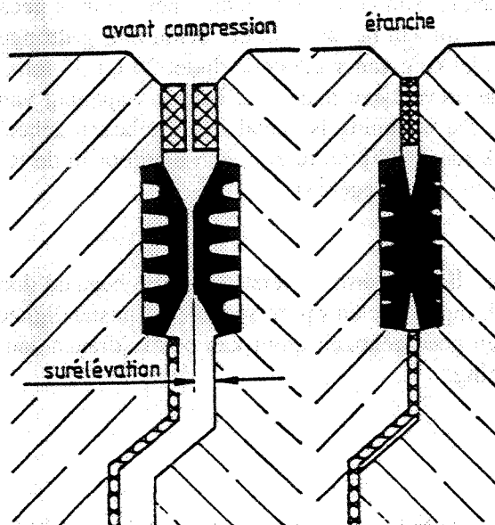
figuur 4.38 Indrukking neopreen profiel
