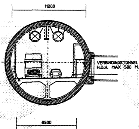
11. STAD/AUTOHIELWEG CAT. A II, 2 RIJSTROOKEN 1 RICHTING (5,55m)
