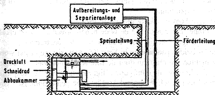
figuur 4.19 Sturing steundruk Duits vloeistofschild
