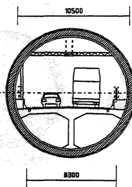
9. MET-AUTOHIELWEG CAT. B IV 1 RIJSTROOK / 2 RICHTINGEN (5,10m)
