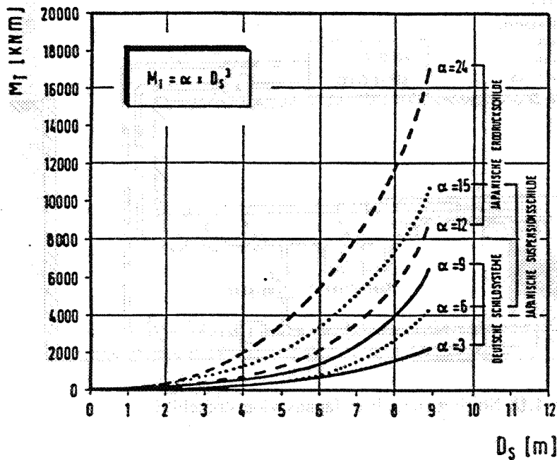
figuur 4.17 Aandrijfmomenten
