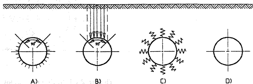
figuur 4.39 Modellering lining-grond systeem
