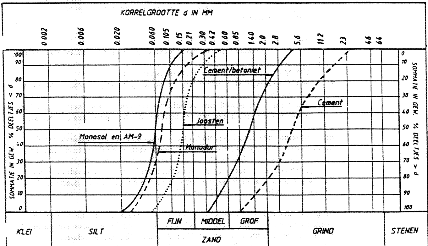
figuur 7.2 Korrelverdelingsdiagram
