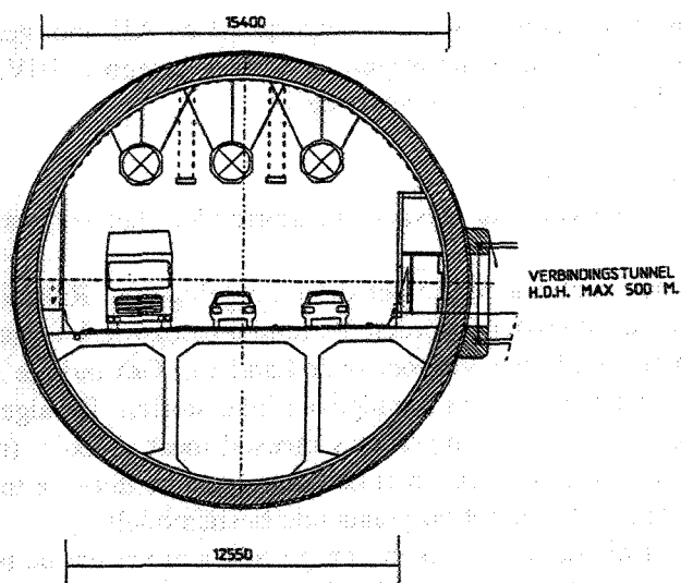
15. AUTOSNELWEG CAT. A1, 3 RIJSTROKEN 1 RICHTING (3.50m)
