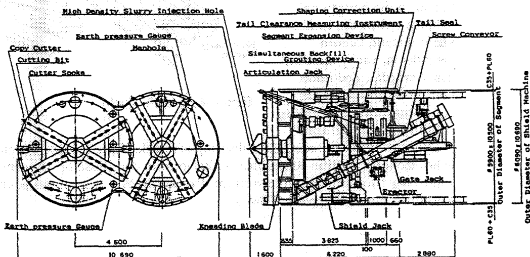
figuur 4.20 DOT Shield voor de Risho Shield Tunnel in Hiroshima
