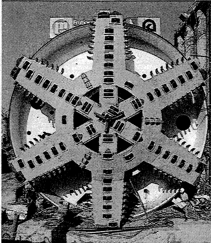
figuur 4.9 Vooraanzicht graafspakenwiel Mixschild
