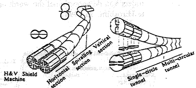
figuur 4.21 H&V shield
