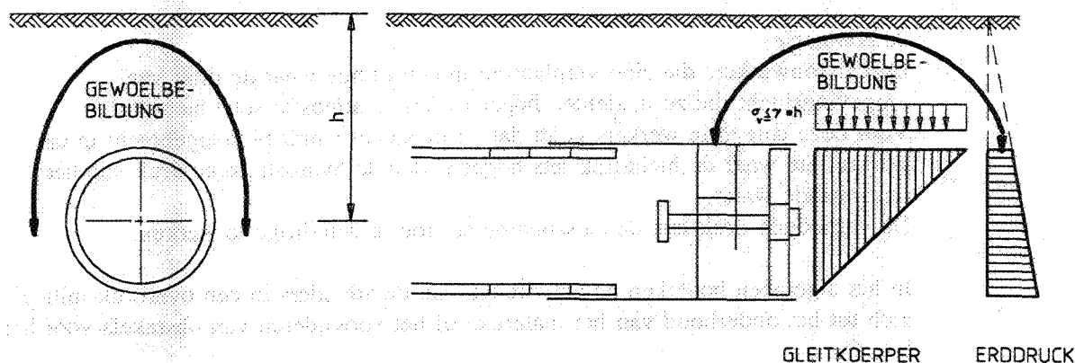
figuur 4.46 Gewelfwerking
