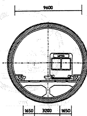
7. METRO, DUBBEL SPOOR
