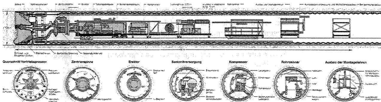
figuur 4.6 "Systeem Thixschild"
