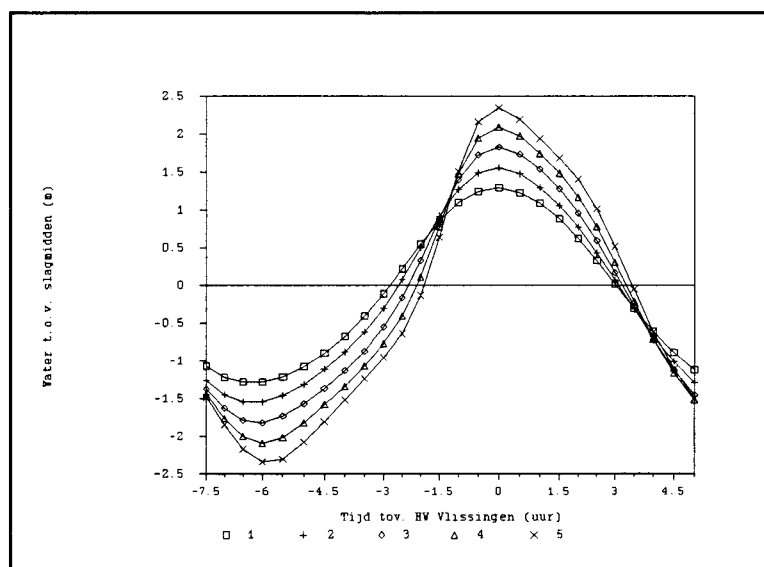
Figuur 6 Astronomische getijde bij Vliessingen, per astro-klasse
