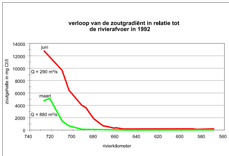
Figuur 11 Verloop van de zoutgradiënt in het Elbe-estuarium in relatie tot de rivierafvoer. Q = gemiddelde maandafvoer (data ARGE-ELBE).
