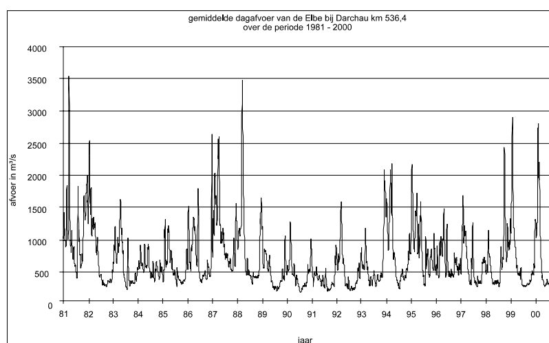
Figuur 3 Gemiddelde dagelijkse afvoer van de Elbe bij Darchau over de periode 1981-2000 (naar data van ARGE ELBE).
