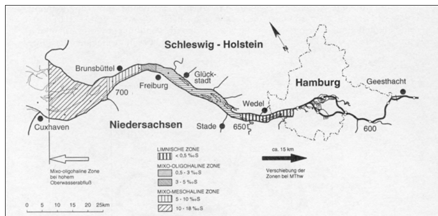
Figuur 12 Ligging van de saliniteitszones bij een lage rivierafvoer een uur voor laagwater (uit Riedel-Lorjé & Ehrhorn, 1998).
