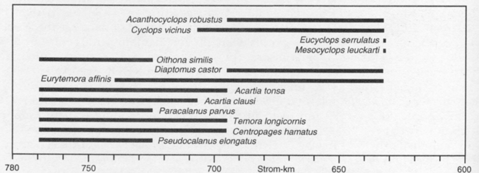
Abb. 25.2 Verbreitung der Ruderfußkreb-Arten > 55 µm im Längsschnitt des Elbe-Aestuars in den Jahren 1986 - 1989 (Daten: PEITSCH 1992)
