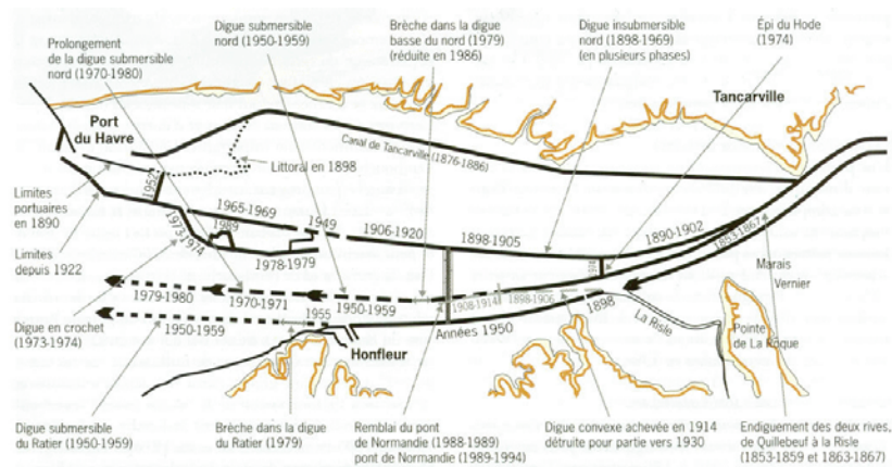
Figuur 39 Bedijkingen ten behoeve van de haven van le Havre en het Kanaal van Rouen (uit Lesueur, 1999).
