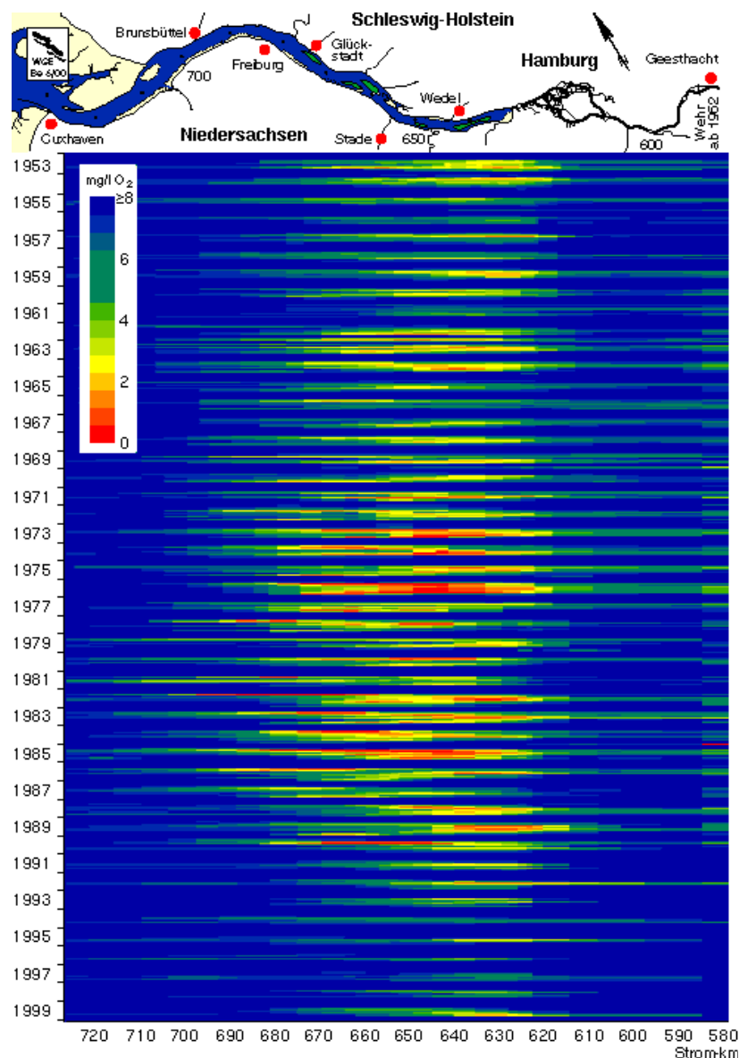
Figuur 24 Het zuurstofgehalte in het Elbe-estuarium van 1953-1999. (ARGE-ELBE, 2000).
