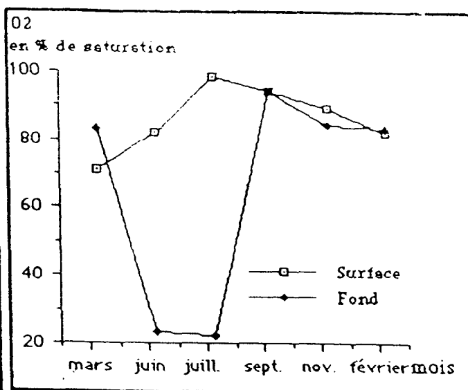
Fig. 10 : Variations saisonnières de l'oxygène dissous à Diam (amont)
