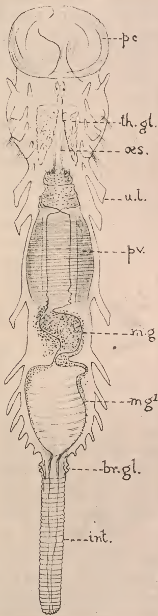
FIG. 139.—Sketch of the alimentary system of a young Sabellaria alveolata . pc., cephalic plate; th.gl., thoracic glands; æs., oesophagus; ul., uncini-gerous lamellæ; pv., proventriculus; mg., anterior stomach; mg', posterior stomach; br.gl., brown glands; int., intestine (after Arnold Watson).
