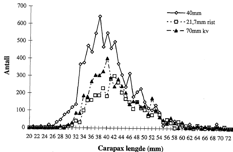
Figur 21. Lengdefordeling av sjøkreps fanget i trippeltrål under forsøkene på Egersundbanken i 1996, rigget med 40 mm vanlige masker, 21,7 mm rist og 70 mm kvadratiske masker [Length distribution of Norway lobster caught in triple trawl during the experiments in 1996, rigged with 40 mm diamond meshes, 21,7 mm grid and 70 mm square meshes].
