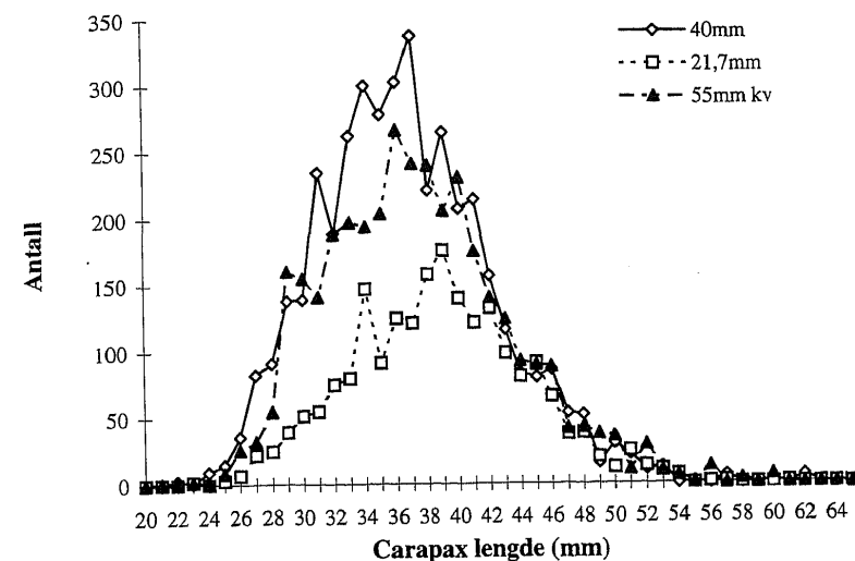
Figur 19. Lengdefordeling av sjøkreps fanget i trippeltrål under forsøkene i Skagerrak i 1995, rigget med 40 mm vanlige masker, 21,7 mm rist og 55 mm kvadratiske masker [Length distribution of Norway lobster caught in triple trawl during the experiments in 1995, rigged with 40 mm diamond meshes, 21,7 mm grid and 55 mm square meshes].
