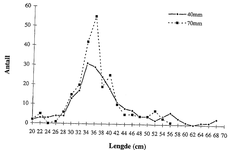
Figur 17. Lengdefordeling av torsk fanget i 40 og 70 mm vanlige masker under forsøkene på Egersundbanken i 1996 [Length distribution of cod caught in 40 and 70 mm diamond meshes during the experiments in 1996].
