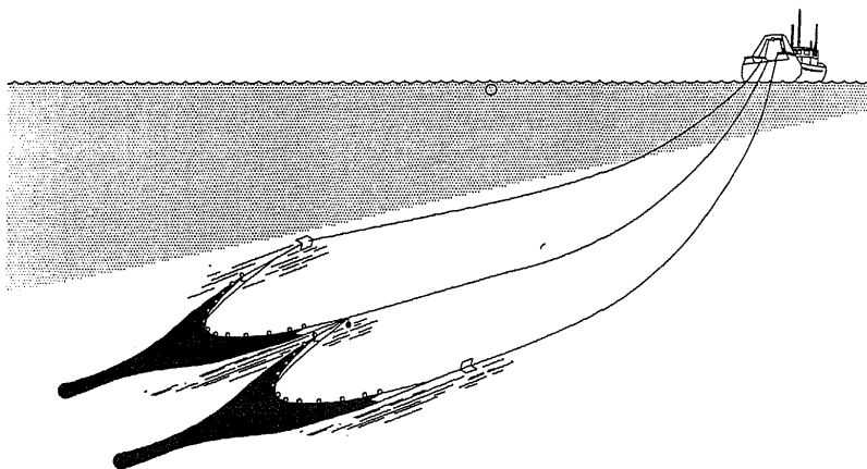
Figur 1a. Tvillingtrål rigget med tre trålwirer [Twin trawl rigged with three towing warps].
