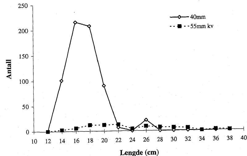
Figur 22. Lengdefordeling av hyse fanget i 40 mm vanlige masker og 55 mm kvadratiske masker under forsøkene på Egersundbanken i 1995 [Length distribution of haddock caught in 40 mm diamond and 55 mm square meshed codends during the experiments in 1995].
