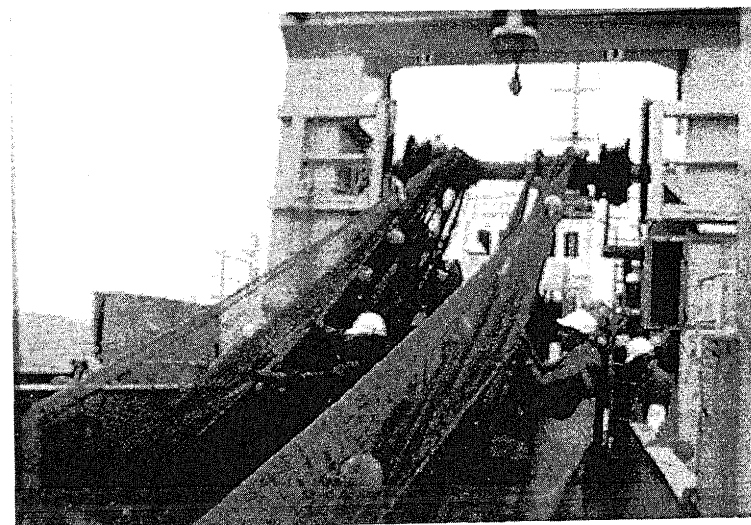
Figur 8. Innhiving av trippeltrål å øverste tråltrommel ombord i "Michael Sars" [Hauling of the triple trawl on board "Michael Sars"].
