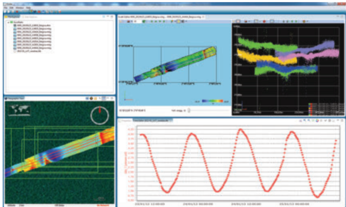
Fig. 1 - GLOBE software.
