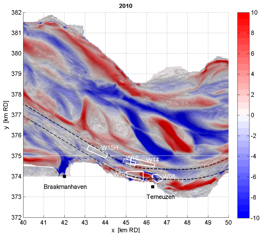
Figuur 2.8 Sedimentatie (rood) en erosie (blauw) tussen 2010 en 1955. De witte polygonen geven de positie van de verschillende stortvakken. De vaargeul is aangegeven met de gestippelde lijnen.
