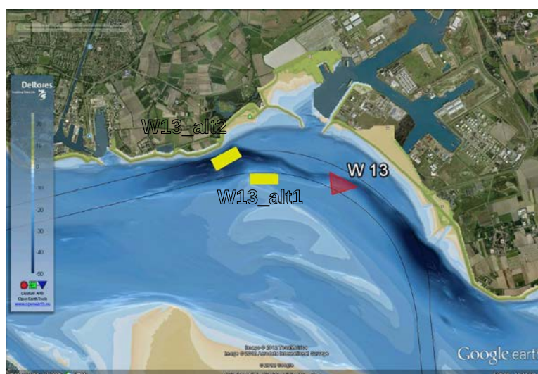
Figuur 2.48 Huidige locatie stortvak W13 (in rode kleur) en mogelijke nieuwe locaties (in gele kleur). De zwarte lijn geeft de ligging van de vaargeul.
