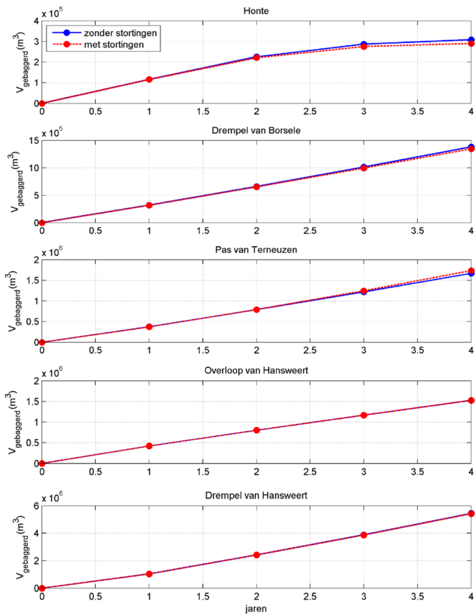
Cumulatief vaargeulonderhoud in vijf deelgebieden volgens modelsimulaties zonder stortingen en met stortingen op alternatieve locaties (alternatief 2).
