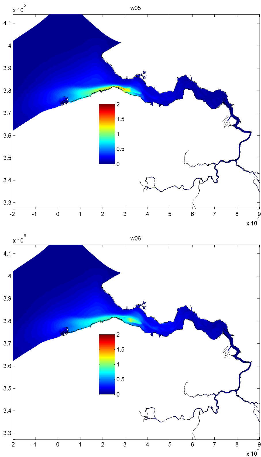
Figuur B.2 Verhoging van slibconcentratie (mg/L) t.g.v. de continue verspreiding van 100 kton/jaar slib vanaf vak W05 (boven) en W06 (onder)
