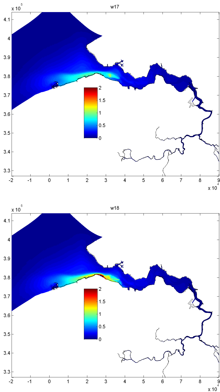
Figuur B.3 Verhoging van slibconcentratie (mg/L) t.g.v. de continue verspreiding van 100 kton/jaar slib vanaf vak W17 (boven) en W18 (onder)
