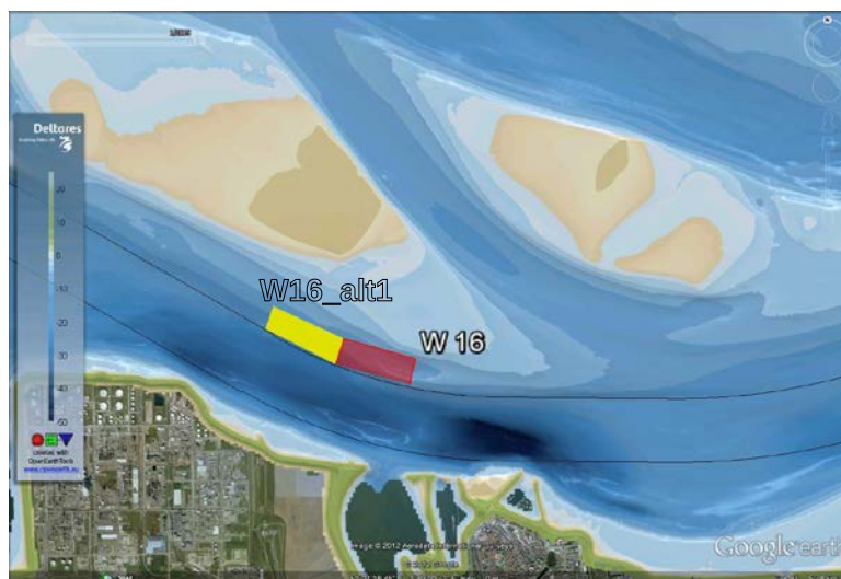
Figuur 2.51 Huidige locatie stortvak W16 (schaduwkleur) en mogelijke nieuwe locatie (in gele kleur). De zwarte lijn geeft de ligging van de vaargeul.
