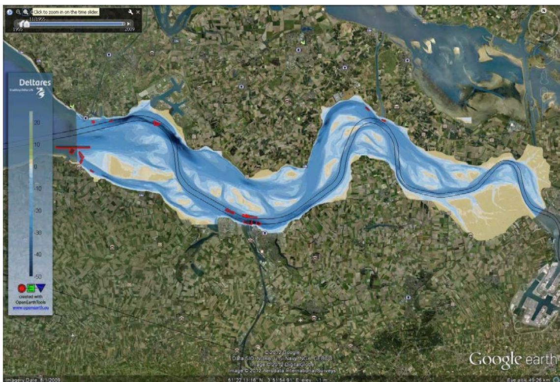
Figuur 2.1 Vaklodingen van het jaar 1955. De locaties van de stortvakken geanalyseerd in deze studie zijn zichtbaar in rode schaduwkleur. De vaargeul is aangegeven met zwarte lijnen.
