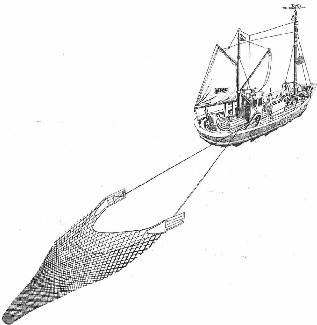
Un chalut à panneaux en action.
