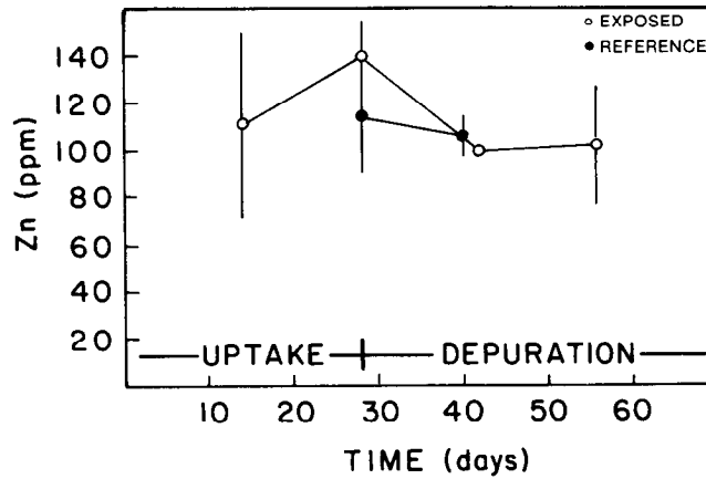
b. Zn
