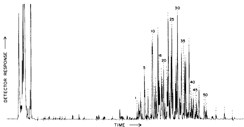
b. Day 14
