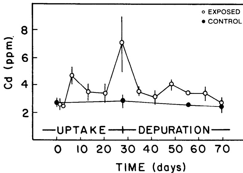
b. Cd
