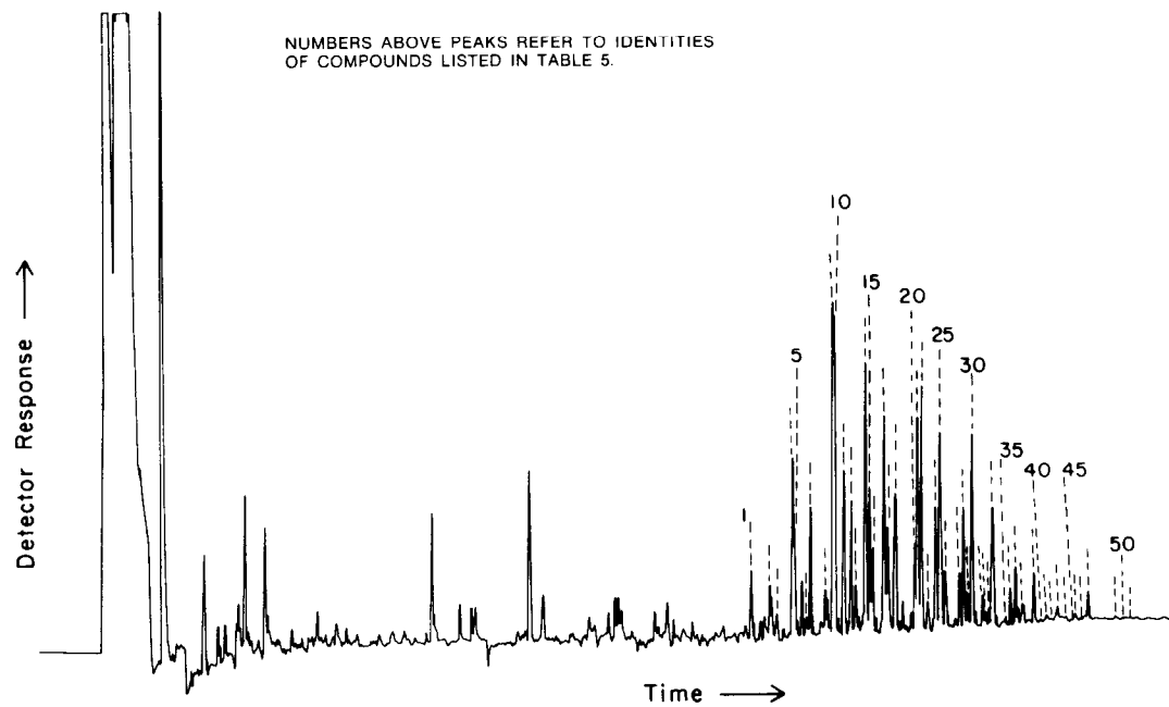
a. Filtrate
