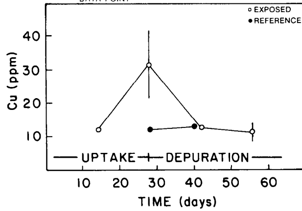
a. Cu
