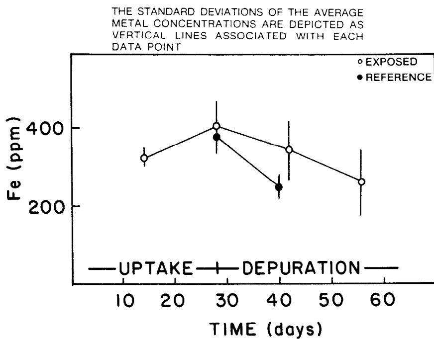
a. Fe
