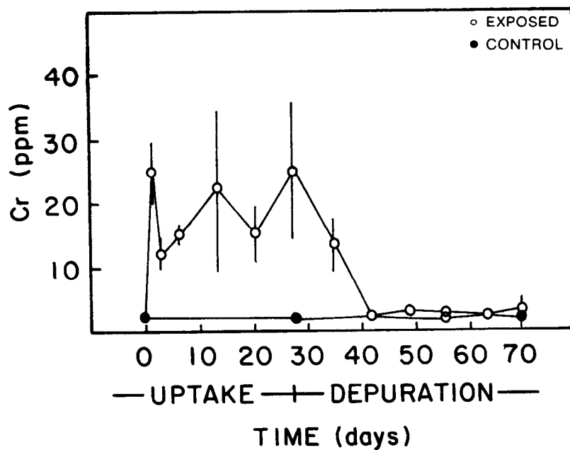
b. Cr
