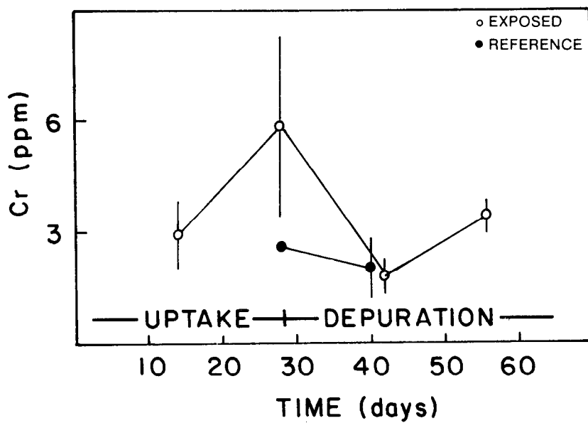
b. Cr
