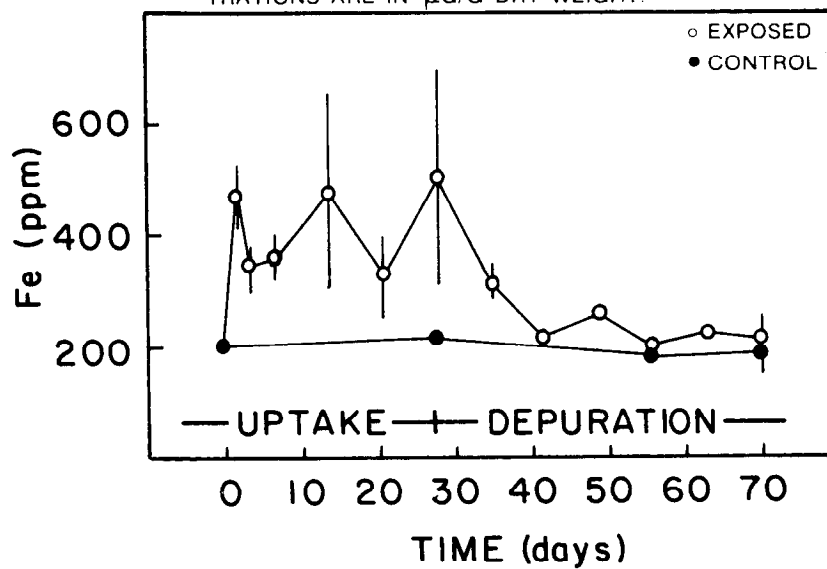
a. Fe
