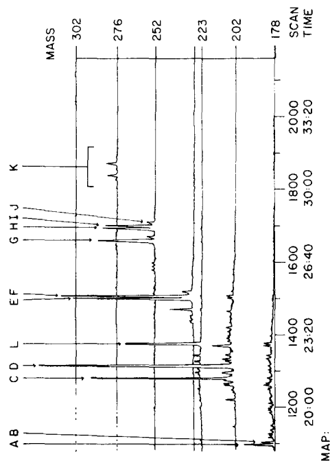
d. Day 28
