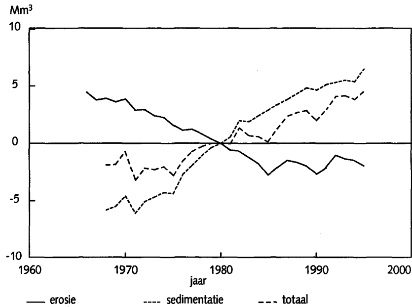
Figuur 3.26 Schouwen; inhoudsveranderingen gehele Noordzeekust, 1965-1995; km 0.84-17.42.
