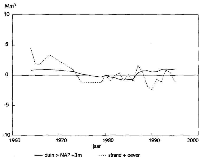
Figuur 3.19 Noord-Holland; inhoudsveranderingen rekenstroken, 1965-1995.
