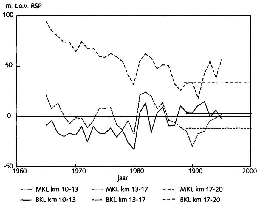
Figuur 3.6 b Ameland; kustlijnverplaatsingen, 1965-1995. b. segmenten
