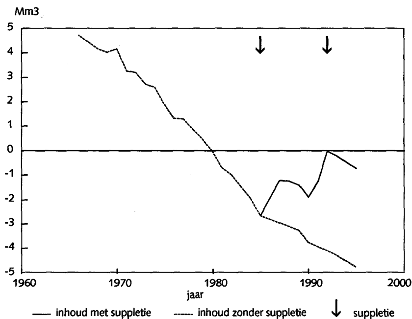
Figuur 3.23 Schouwen; inhoudsveranderingen en suppleties, 1966-1995; km 10.84- 16.97.
