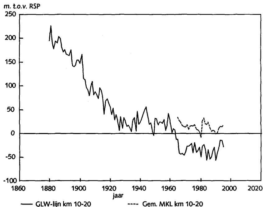
Figuur 3.7 Ameland; lange termijn ontwikkeling laagwaterlijn, 1880-1995.
