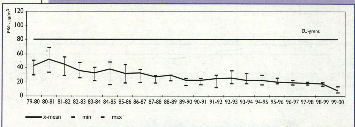
Figuur 3.10.a: \text{SO}_2 -mediaanwaarde, steden x-mean, hoogste en laagste in Vlaanderen
