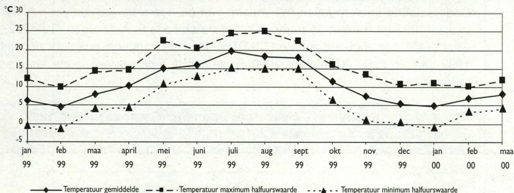
Figuur 14.3: Temperatuur T4M705 Roeselare in de periode januari 1999 tot en met maart 2000
