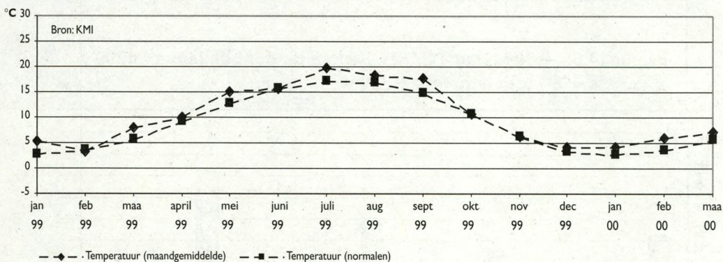
Figuur 14.4: Temperatuur Ukkel in de periode januari 1999 tot en met maart 2000
