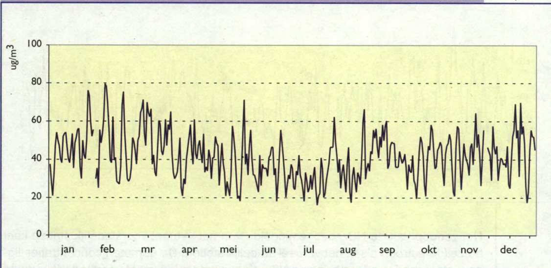
Figuur 4.4: Daggemiddeld \text{NO}_2 -verloop in het stedelijk x-mean station in het kalenderjaar 1999
