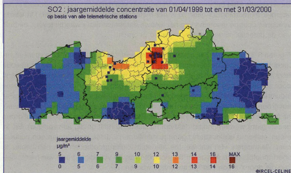
Figuur. 3.1: SO 2 -jaargemiddelde concentratie in het meteorologisch jaar 1999-2000
