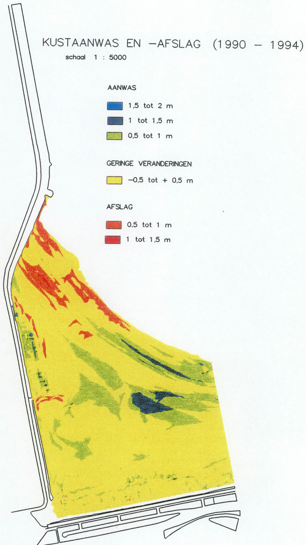
Figuur 7: Strandvlakte Heist-West: kustaanwas en -afslag tussen 1990 en 1994
