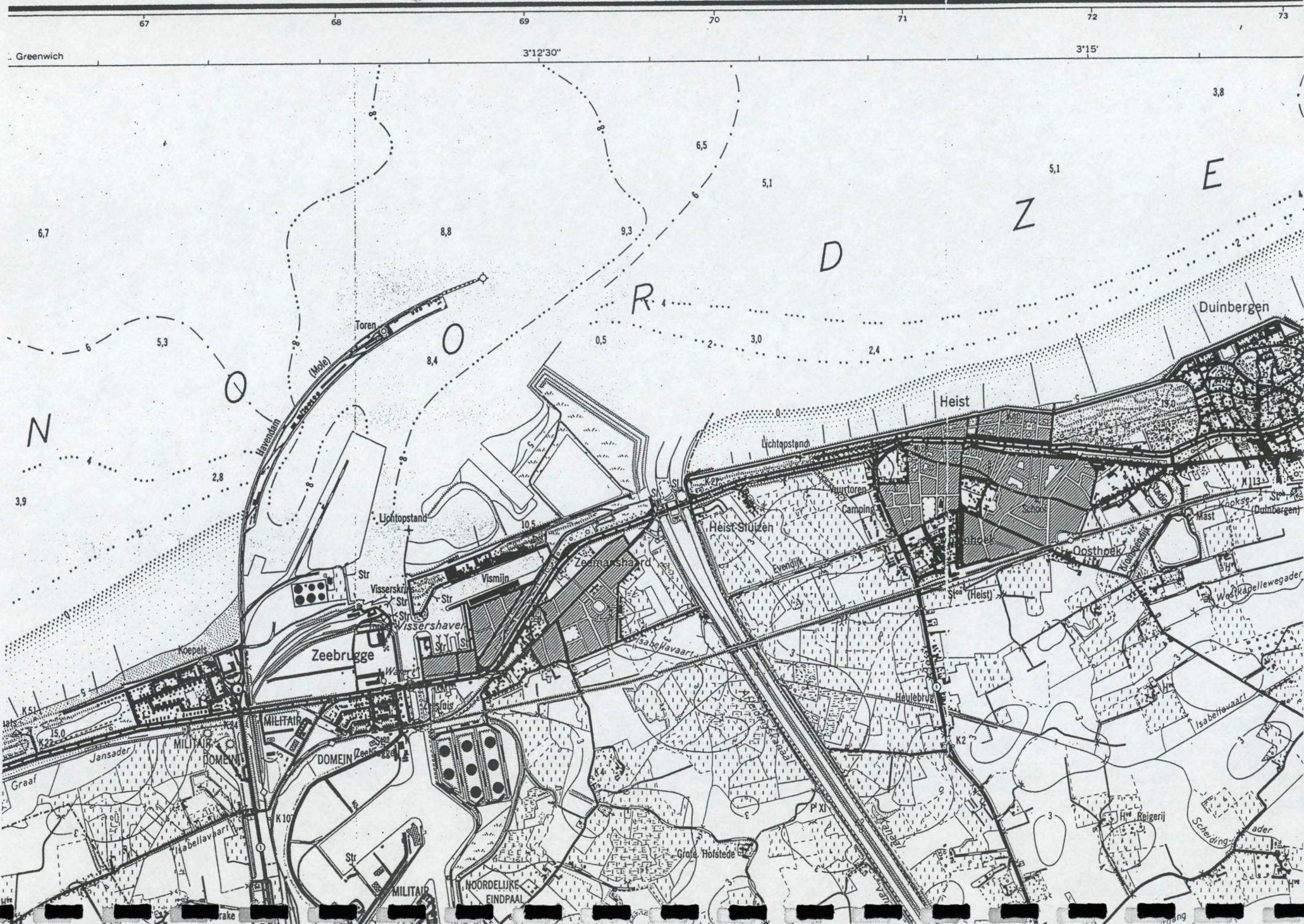
Figuur 1: De haven van Zeebrugge en het strand van Heist-West in 1971 (topografische kaart van het Militair Geografisch Instituut, schaal 1/25 000, kaartblad 5/5-6 Heist-Westkapelle)
