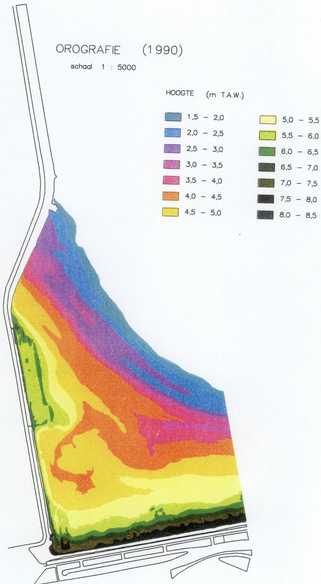
Figuur 4: Orografie van de strandvlakte van Heist-West in 1990
