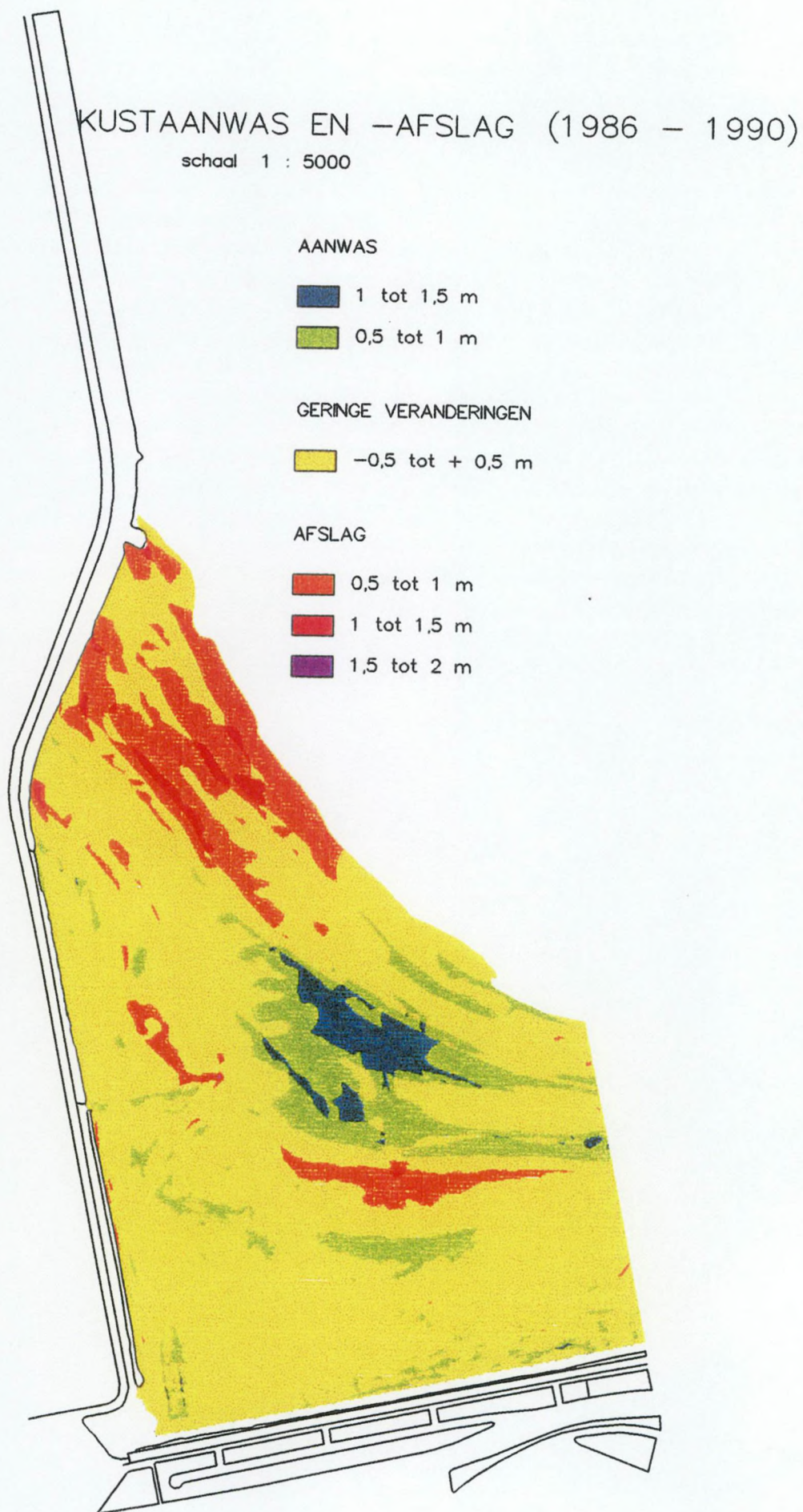
Figuur 6: Strandvlakte Heist-West: kustaanwas en -afslag tussen 1986 en 1990
