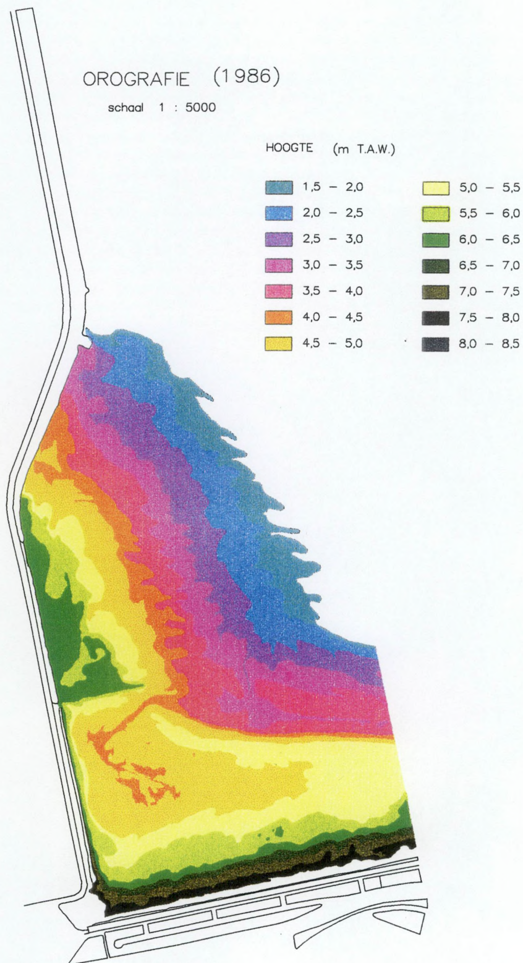
Figuur 3: Orografie van de strandvlakte van Heist-West in 1986
