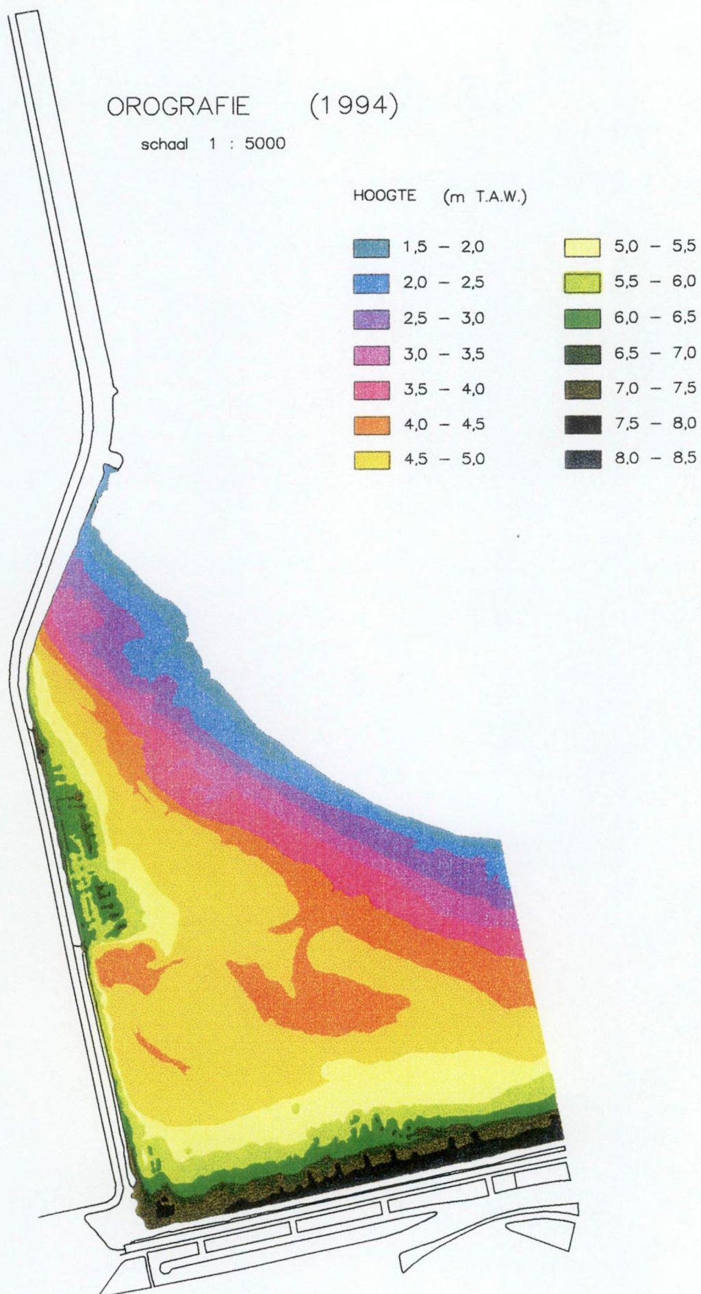
Figuur 5: Orografie van de strandvlakte van Heist-West in 1994
