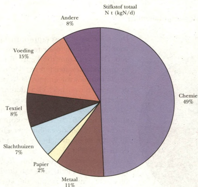
Fig 3.12 Aandeel per sector: totaal stikstof N t
