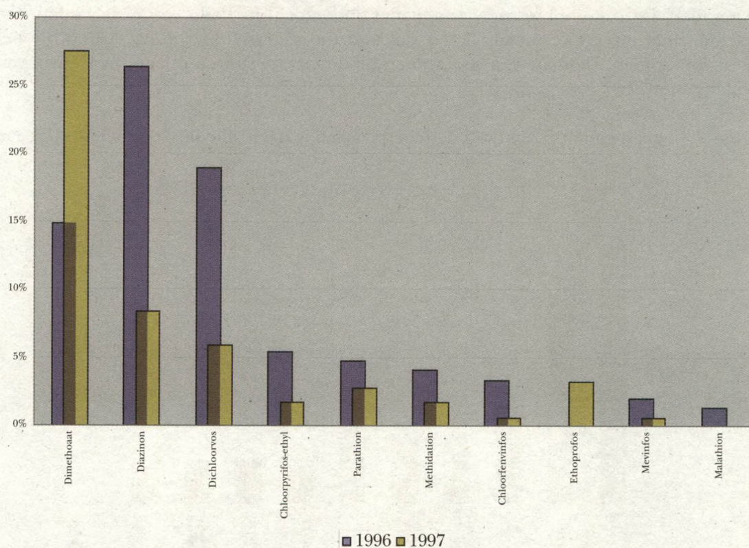
Figuur 2.17 : Organofosforpesticiden
