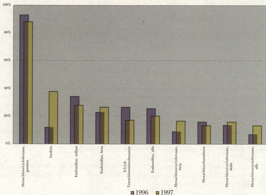
Figuur 2.12 : Organochloorpesticiden
