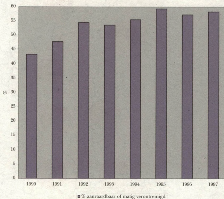
Figuur 2.2 : Percentage van de meetplaatsen met een aanvaardbare of matig verontreinigde waterkwaliteit voor de periode 1990-1997
