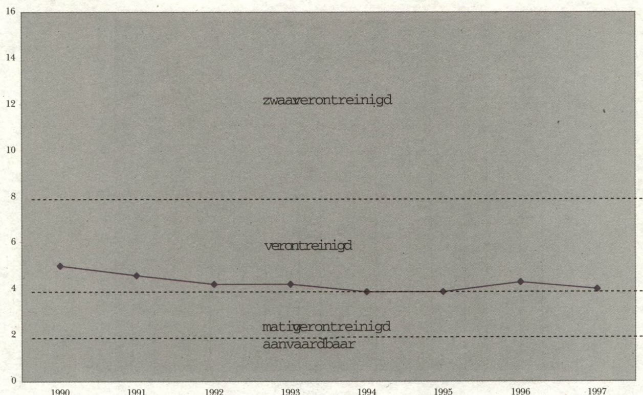
Figuur 2.3 : Evolutie van de gemiddelde PIO-waarde voor de periode 1990-1997
