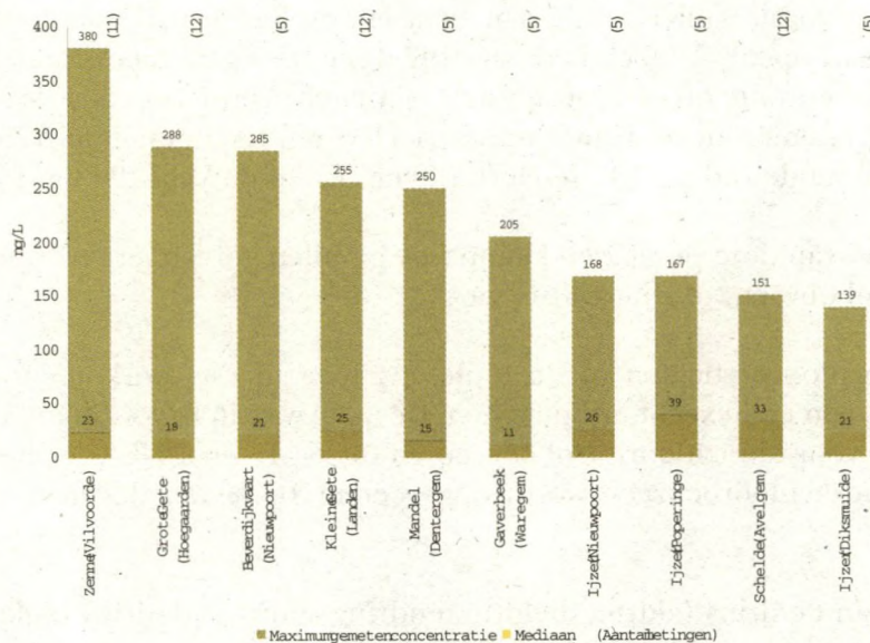
Figuur 2.13: Maximaal gemeten concentratie, mediaan en aantal metingen van Hexachloorcyclohexaan, gamma voor de jaren 1996-1997
