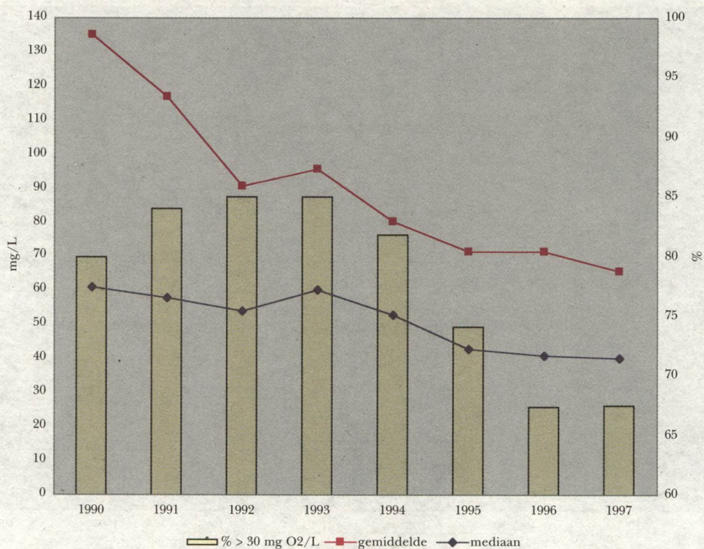
Figuur 2,4 : Chemisch Zuurstofverbruik
