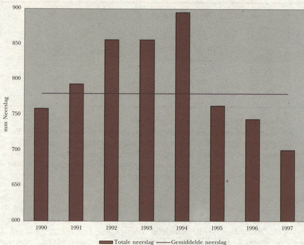
Figuur 2.1 : Totale Neerslag 1990-1997
