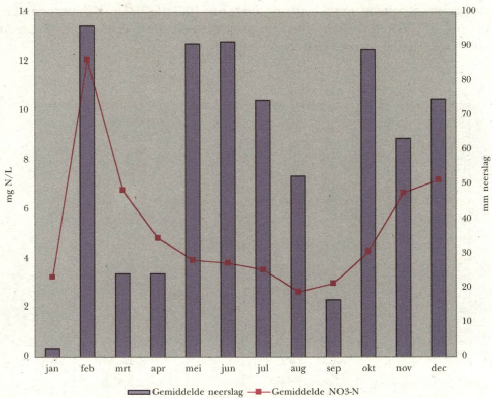
Figuur 2.9 : maandgemiddelde nitraat en neerslag
