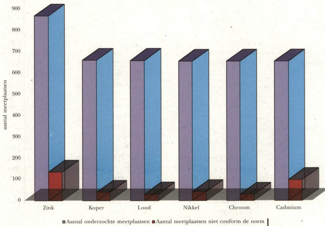
Figuur 2.11 : Zware metalen : toetsing aan de basiskwaliteitsnorm
