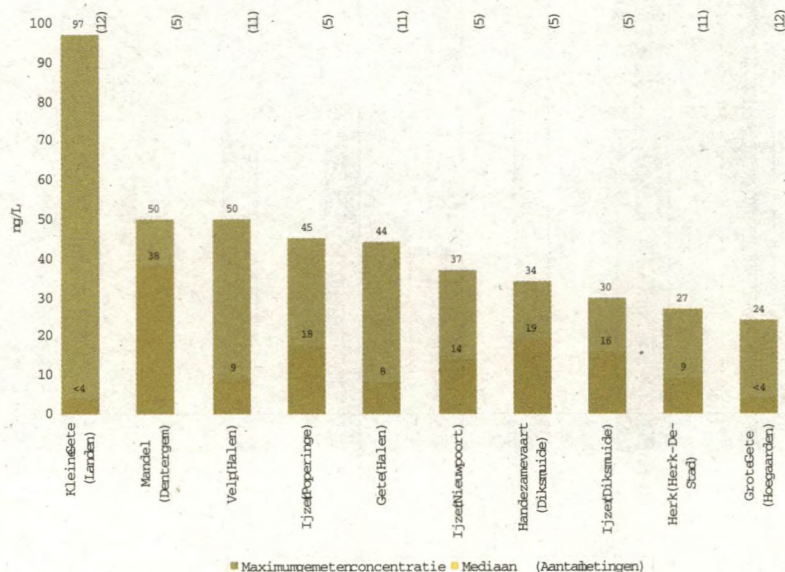
Figuur 2.14: Maximaal gemeten concentratie, mediaan en aantal metingen van Endosulfan, sulfaat voor de jaren 1996-1997
