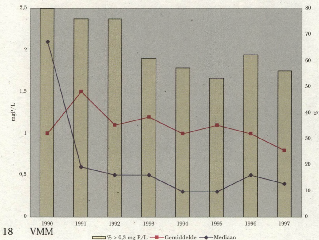
Figuur 2.10 : Totaal ortho-fosfaat
