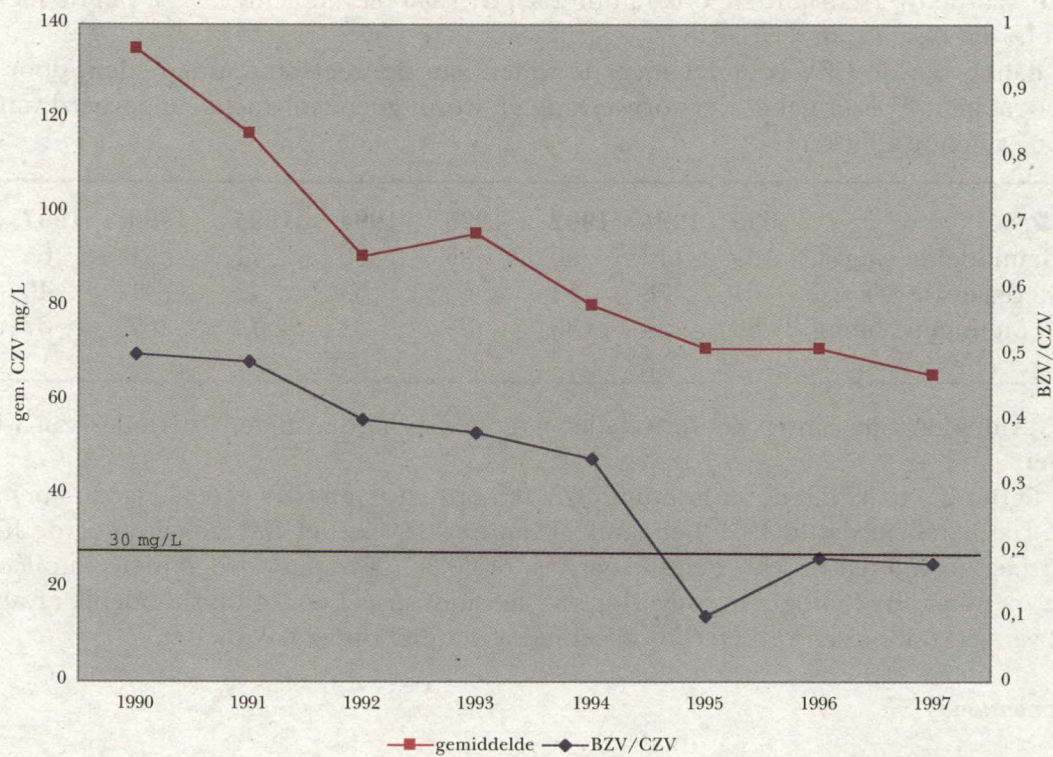
Figuur 2.5 : Gemiddeld CZV en verhouding BZV/CZV
