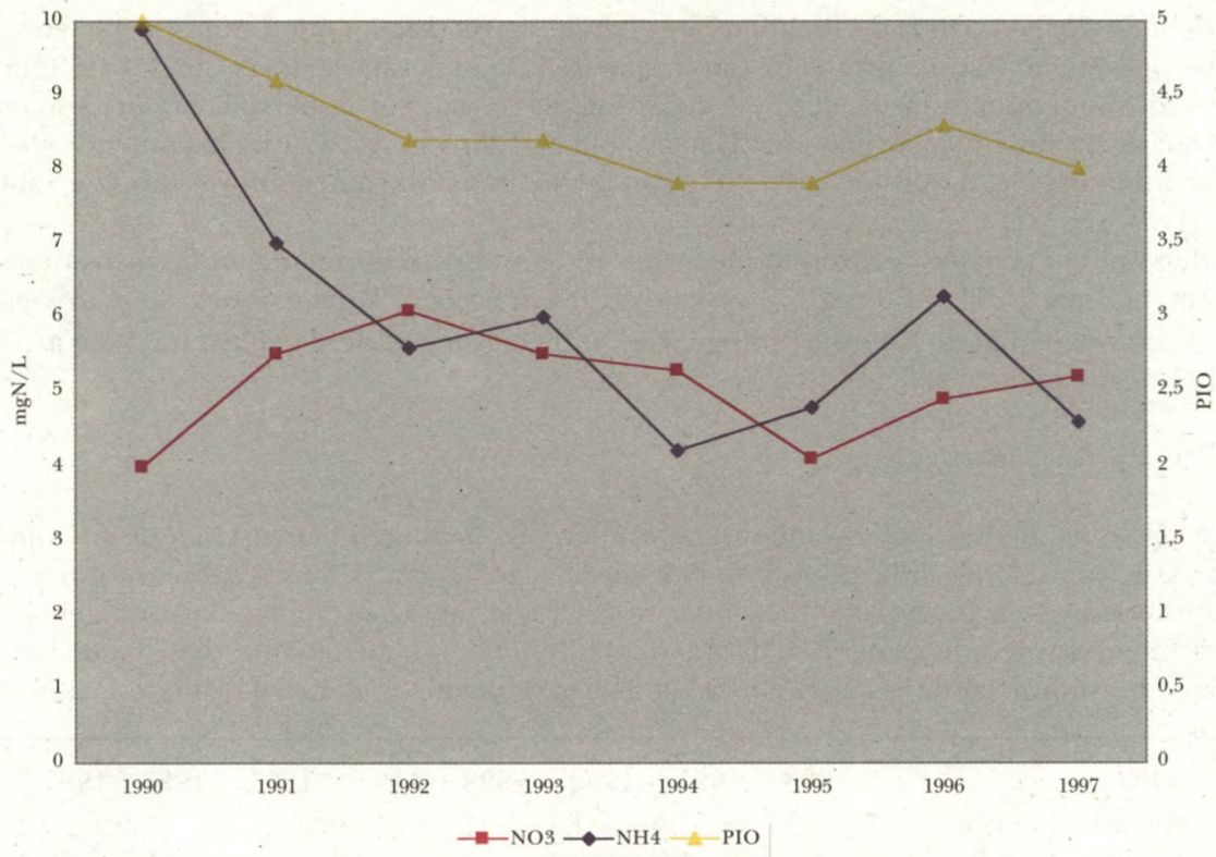
Figuur 2.8 : Evolutie van het nitraatgehalte, het ammoniumgehalte en de PIO in de periode 1990-1997
