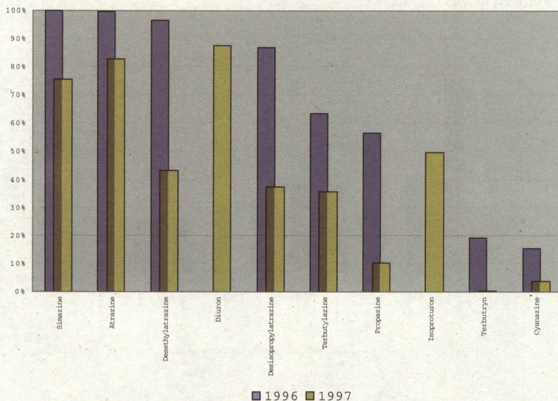
Figuur 2.15: Organostikstofpesticiden
