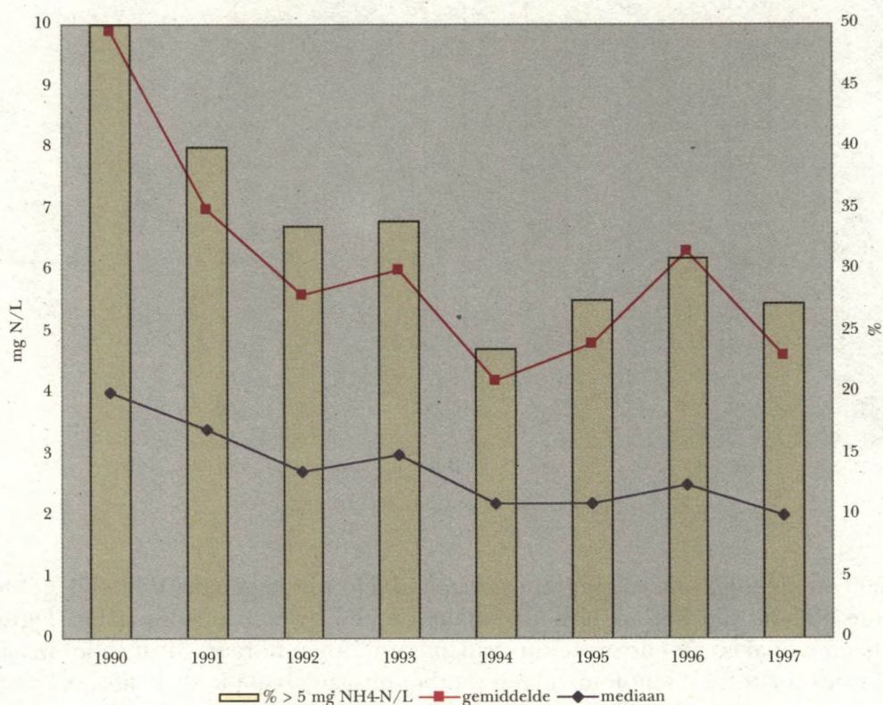
Figuur 2.6 : Ammoniakale stikstof
