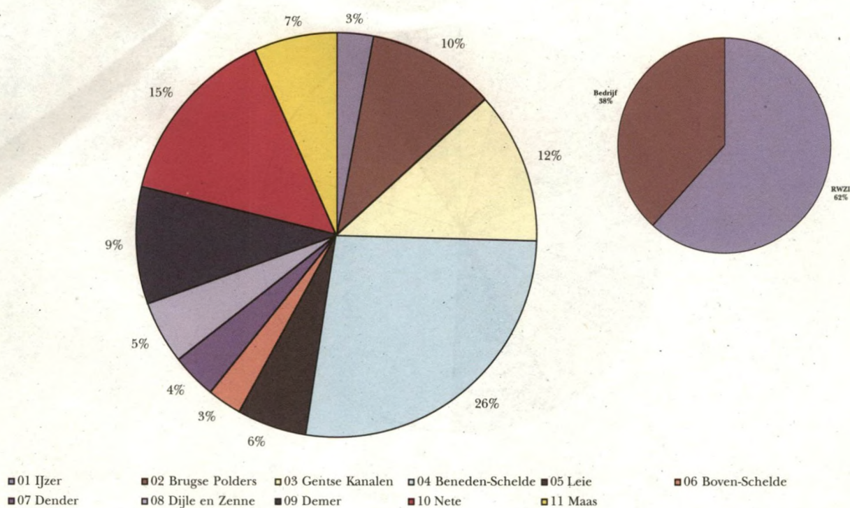
Fig. 3.2 Overzicht geloosde vracht biochemisch zuurstofverbruik BZV
