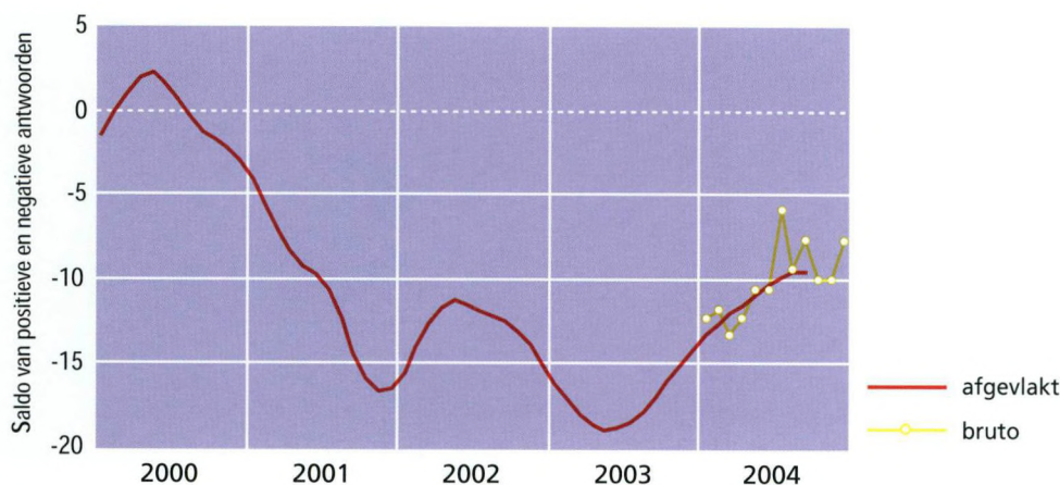
Figuur: Synthetische conjunctuurcurve voor West-Vlaanderen, 2000-2004 | Bron: NBB, Verwerking: GOM - West-Vlaanderen.
