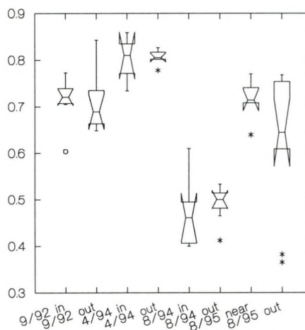
Fig. 3.7.7d. Evenness E (Pielou)
