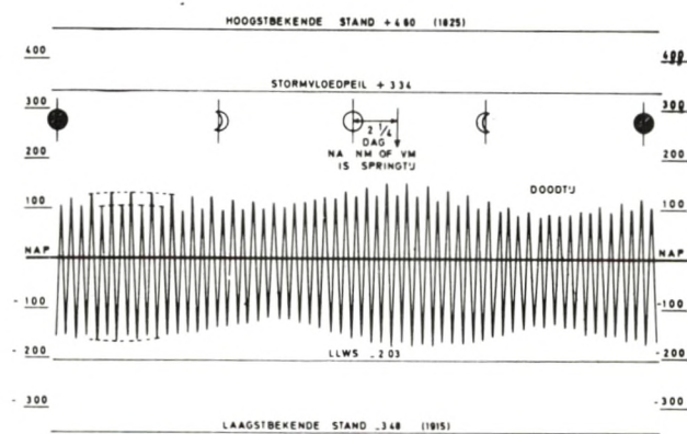
Fig.12 c . Voorbeeld van het verloop der getijbeweging te Delfzijl van nieuwe maan tot nieuwe maan
