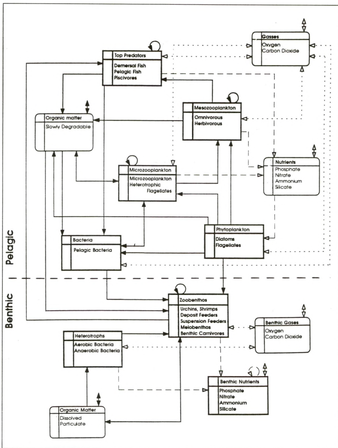
Fig. 2.1. Vereenvoudigd schema van het ecosysteem in de Nederlandse kustzone. Vogels en zeezoogdieren zijn buiten beschouwing gelaten (Naar BLACKFORD & RADFORD, 1994, in press).
