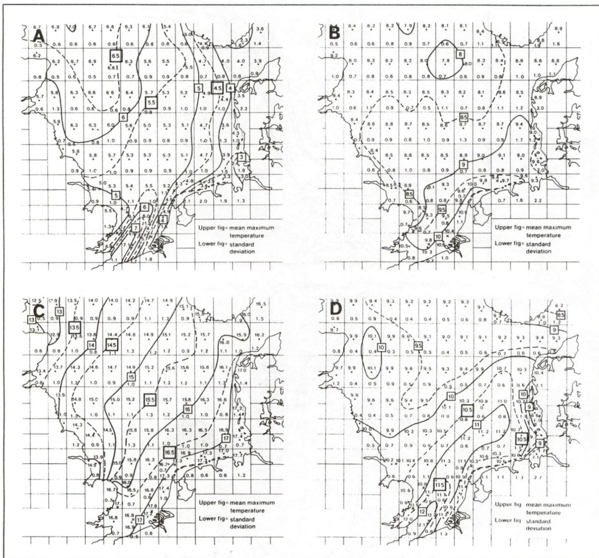
Fig. 3.4. Gemiddelde oppervlakte temperatuur in de Noordzee (1961-1980) voor de maanden februari (A), mei (B), augustus (C) en november (D) (KOREVAAR, 1990).
