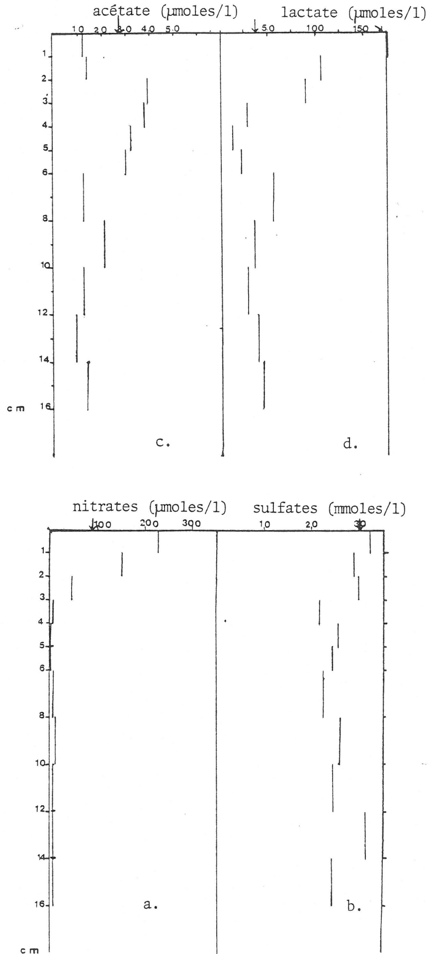
Figure 1. Concentration en Nitrate (a), Sulfate (b), acetate (c) et lactate (d) dans l'eau interstitielle d'une carotte vaseuse du Bassin de Chasse d'Ostende (B 6/2/79).
