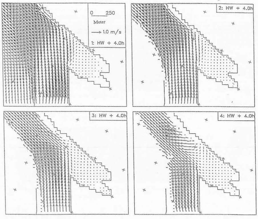
Fig. 10 : Springtij hoge saliniteit. Strooming in de toegangsgeul 4 uur na HW.
