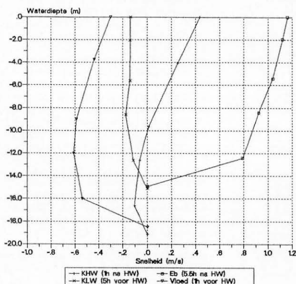
Fig. 5: Springtij 04/10/90 - Hoge Saliniteit Snelheidsverticalen Meetpunt 1 (3D Model)
