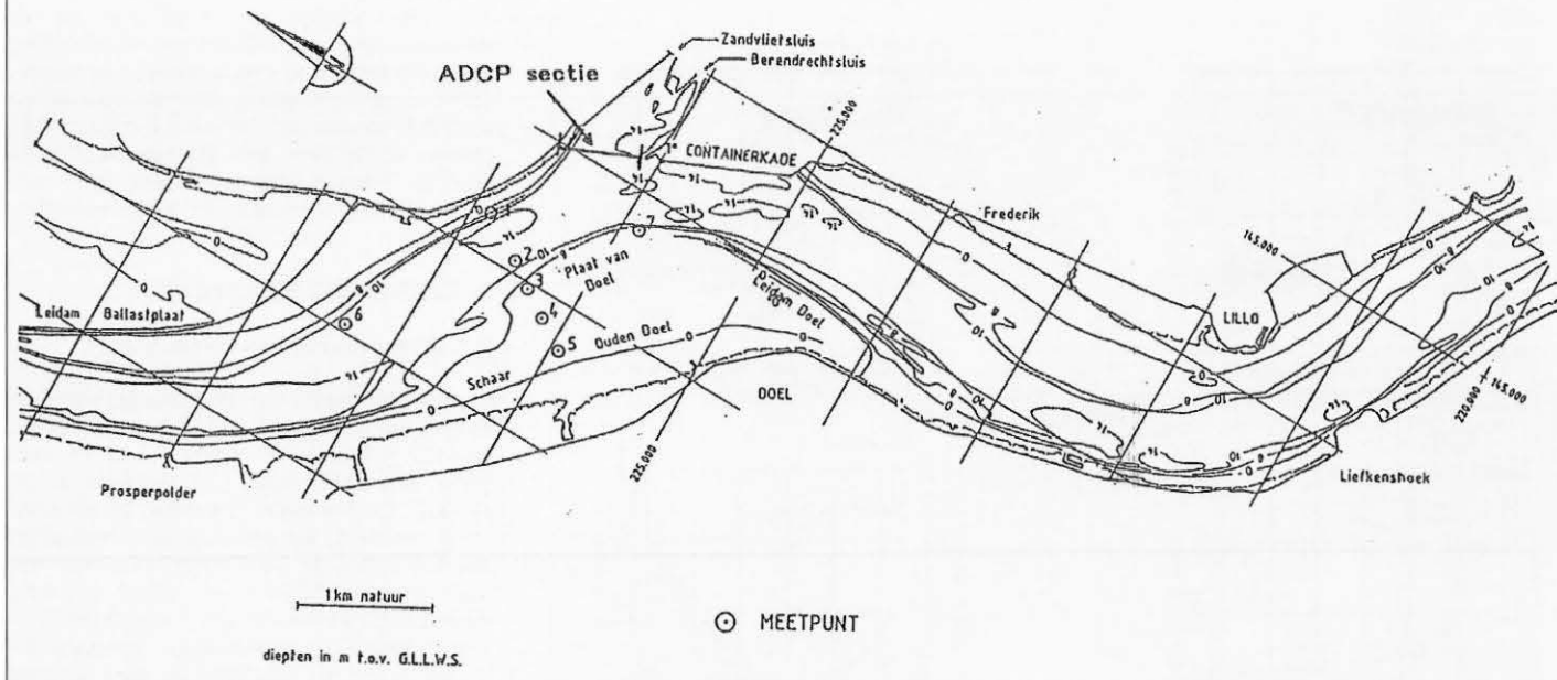
Fig. 2: Ligging van de meetpunten voor de springtijmeting van 4/10/90 en de doortijmeting van 27/9/90 en de vaarroute van de ADCP metingen op 19 en 29/4/93.
