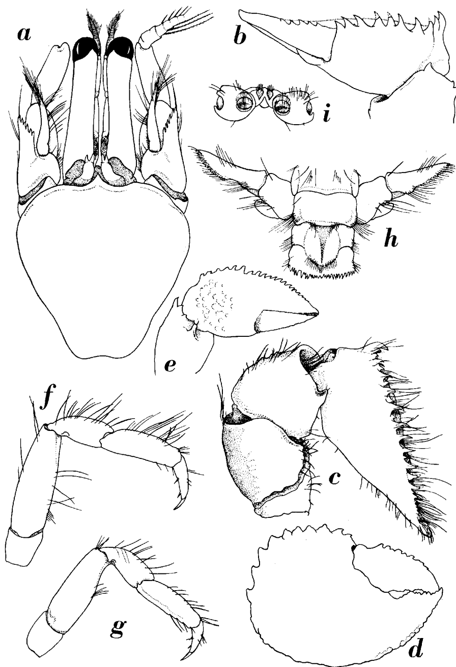
Fig. 2. Paguritta corallicola n. sp. a, Holotypus; b-i, Paratypus. a, Vorderkörper; b, rechte Schere (Innenseite); c, rechter Scherenfuss (Aussenseite); d, rechte Schere, von oben gesehen; e, linker Scherenfuss, schräg von oben gesehen; f, 2. Pereiopod; g, 3. Pereiopod; h, Telson; i, Geschlechtsöffnungen (Männchen). a-h, \times 14 ; i, \times 28 .
