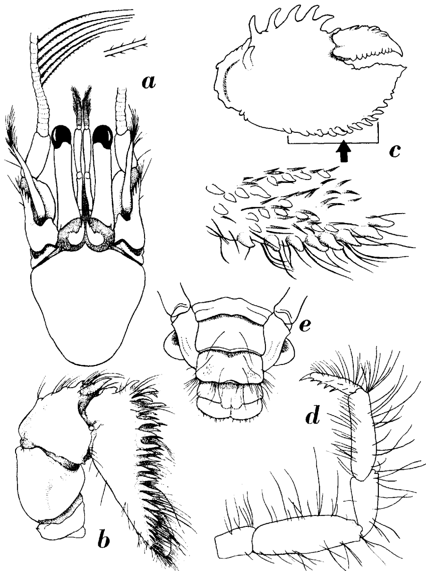
Fig. 1. Paguritta harmsi (Gordon). a-c, Holotypus; d-e, Paratypus. a, Vorderkörper; b, rechter Scherenfuss (Aussenseite); c, rechte Schere, von oben gesehen; d, 2. oder 3. Pereiopod; e, Telson. a-e, \times 14 .
