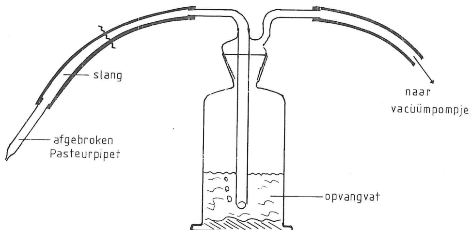
Fig. 2. De afzuigopstelling.
