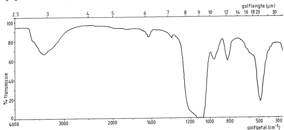
Fig. 6. Voorbeeld van een infraroodspectrum van diatomeeën (methode a).
