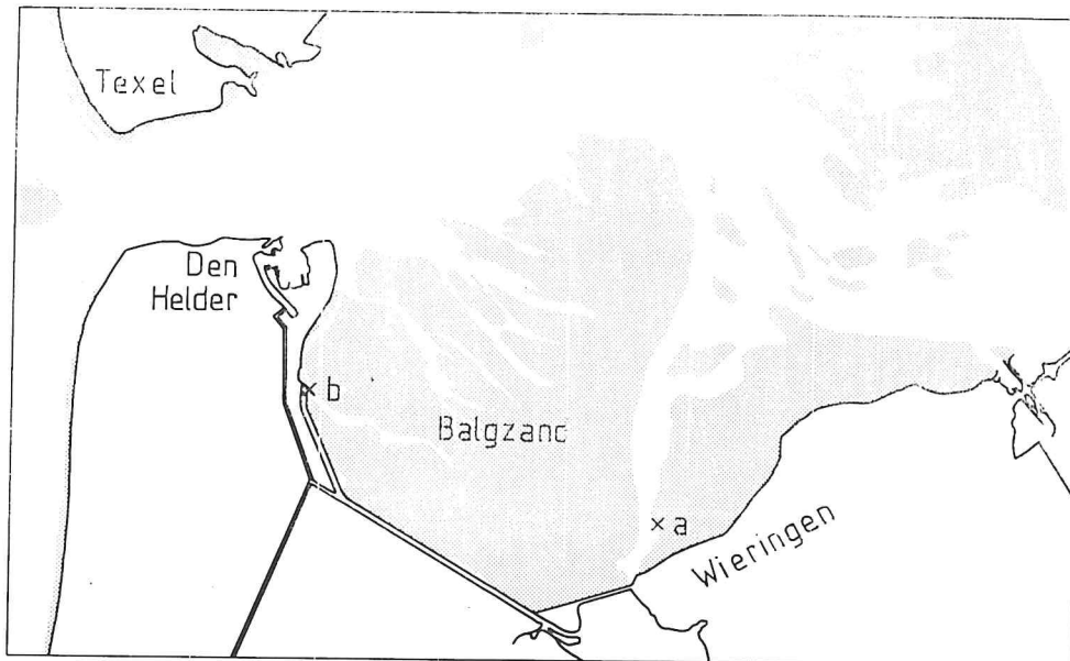
Fig. 1. De monsterplaatsen. a. Slib 28-7-77. b. Overige monsters. geëgaliseerd. De bak wordt in daglicht opgesteld. Na \frac{1}{2} dag wordt de oppervlaktelaag, waar de diatomeeën ingekropen zijn, afgezogen met een vacuumpompje: zie Fig. 2.
