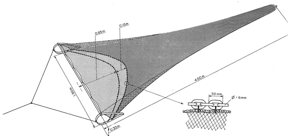
Fig. 3. De 2-meter boomkor (naar KUIPERS, 1975).
