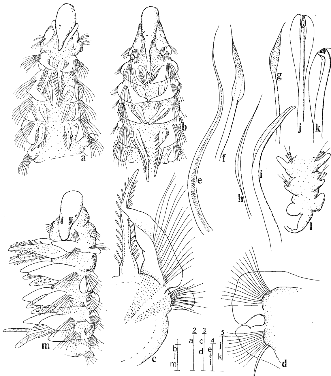
Figure 20— Prionospio steenstrupi Malmgren—a, anterior end, dorsal view— Prionospio australiensis nov. sp.—b, anterior end, dorsal view; c, left setiger 4, anterior view; d, right setiger 13, anterior view; e, capillary notoseta, setiger 4 from posterior tier; f, capillary notoseta, setiger 4 from anterior tier; g, sheathed neuroseta, setiger 4; h, capillary neuroseta, setiger 13; i, sabre seta; j-k, multidentate hooded hooks; l, posterior end, dorsal view— Prionospio ehlersi Fauvel—m, anterior end, dorsolateral view. [Scale 1 = 200 \mu m; 2 = 200 \mu m; 3 = 50 \mu m; 4 = 20 \mu m]
