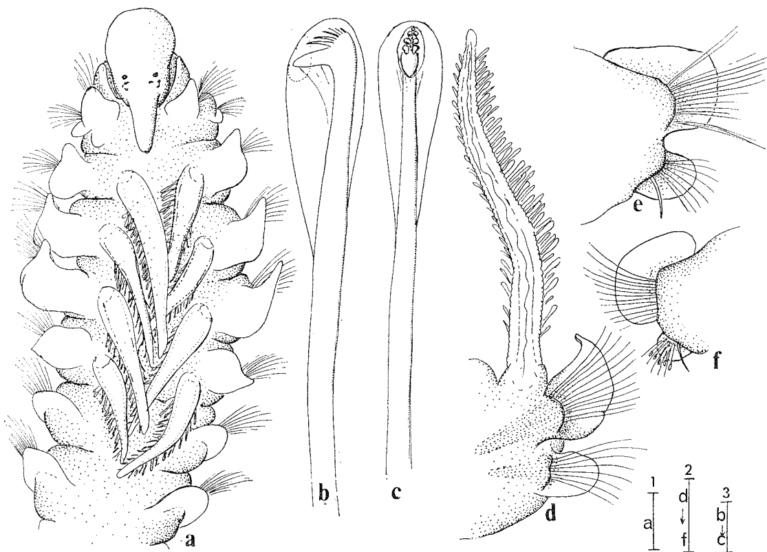
Figure 24— Prionospio multipinnulata sp. nov.—a, anterior end, dorsal view; b-c, hooded hooks; d, left setiger 4, anterior view; e, left setiger 10, anterior view; f, right setiger 20, anterior view. [Scale 1 = 200 \mu m; 2 = 200 \mu m; 3 = 20 \mu m]
