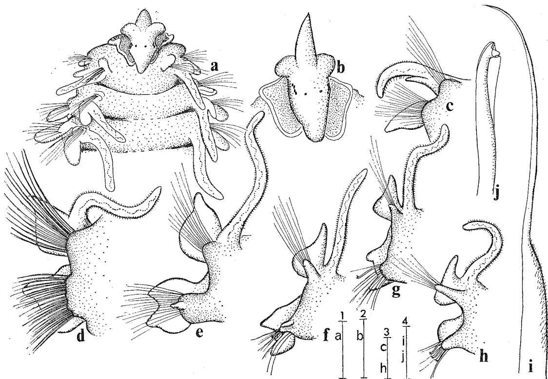
Figure 11— Australospio trífida gen et sp. nov.—a, anterior end, dorsal view; b, prostomium, dorsal view; c, right setiger 1, anterior view; d, right setiger 7, anterior view; e, right setiger 15, anterior view; f, right setiger 22, anterior view; g, right setiger 40, anterior view; h, right setiger 50, anterior view; i, neuroseta from setiger 7; j, bidentate hooded hook. [Scale 1 = 100 \mu m; 2 = 50 \mu m; 3 = 200 \mu m; 4 = 30 \mu m]
