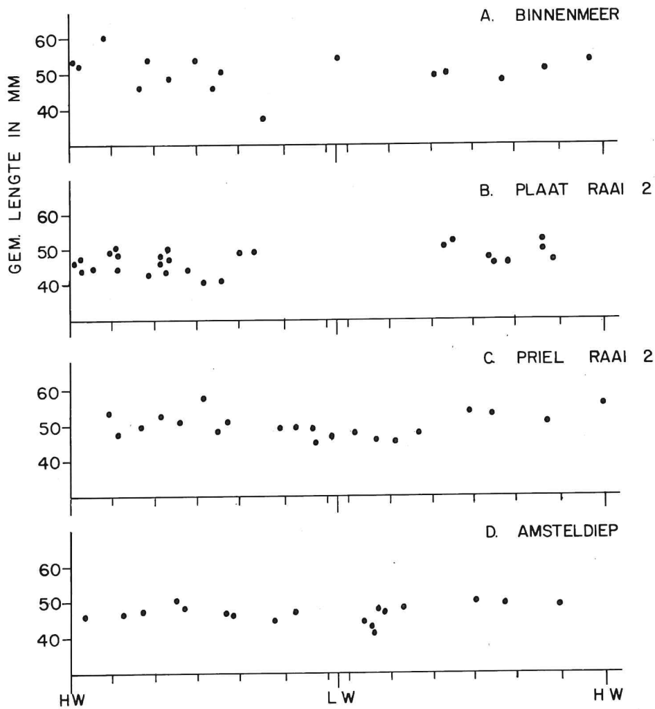
Fig. 18. Gemiddelde lengte van 0-groep schol gedurende het getij in de week van 21/6-25/6 1976.
