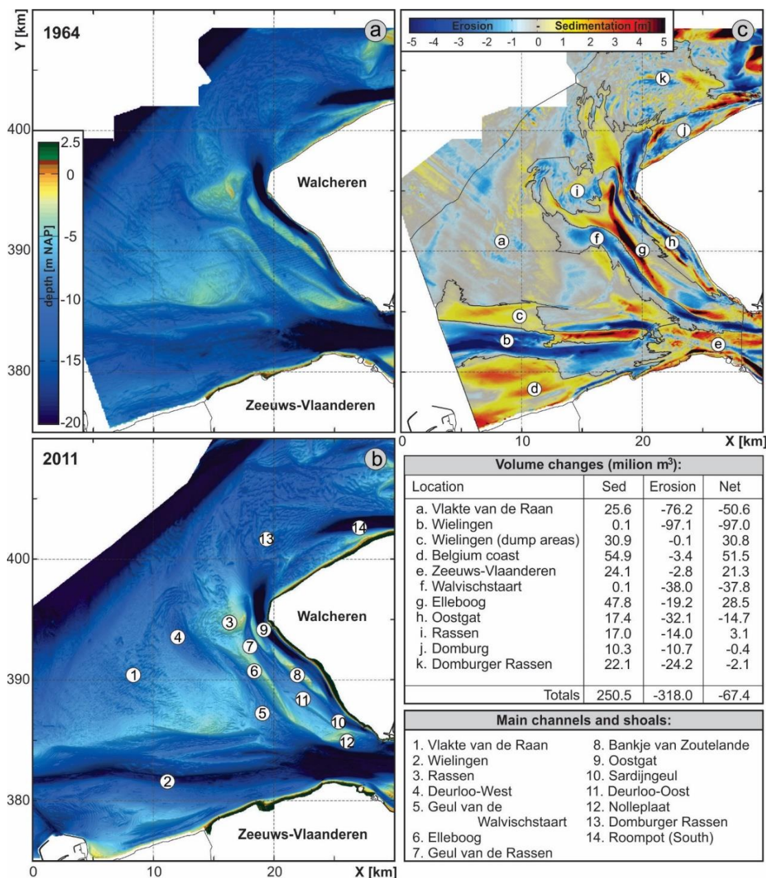
Figuur 2.7 Details van de bodem van de Westerscheldemonding in 1964 (a) en 2011 (b) en overzicht van de totale volumeverandering in geselecteerde polygonen over de periode 1964- 2011 (c). (figuur afkomstig uit Elias et al., 2016)
