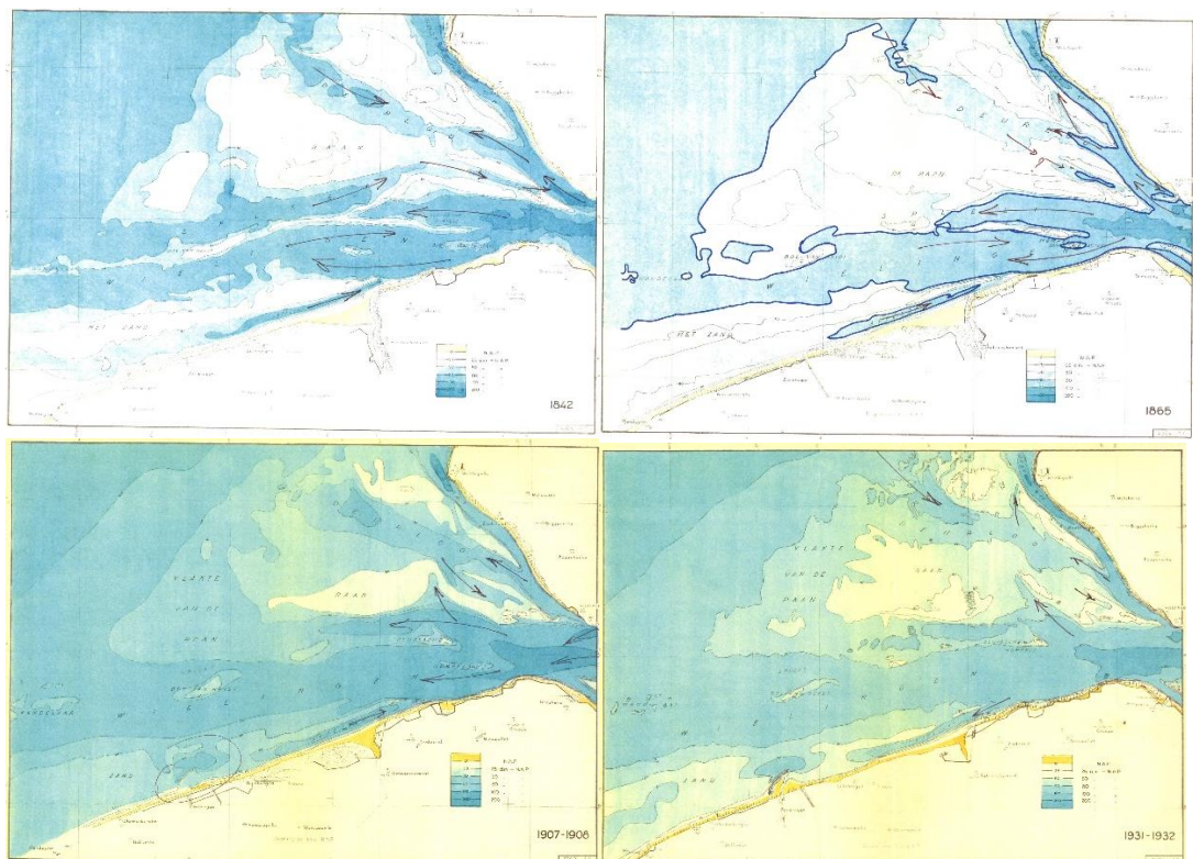
Figuur 2.5 De ontwikkeling van geulen en platen in de Westerscheldemonding tussen 1842 en 1931-1932. De afgebeelde kaarten zijn van 1842, 1865, 1907-1908 en 1931-1932. Zie tekst voor beschrijving van de veranderingen (bron: Rijkswaterstaat, zonder jaar).
