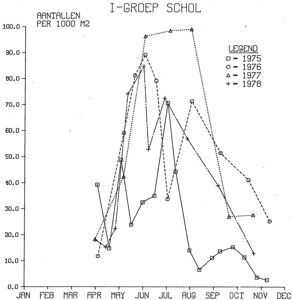
Fig. 3. Gemiddelde dichtheid van I-groep schol op het Balgzand rond HW. Aantallen per 1000 m 2 zijn gemiddelden uit 40 trekken, gecorrigeerd voor net-efficiency.
