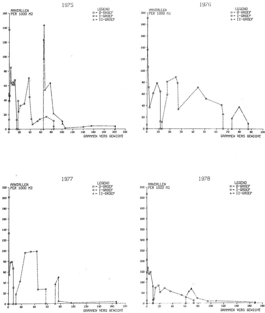
Fig. 7. Allen-curves van de drie leeftijdsgroepen schol op het Balgzand.
