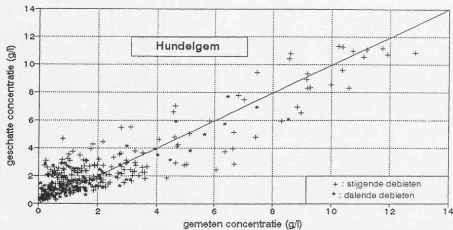
Figuur 2: Vergelijking van gemeten en geschatte concentraties in het meetpunt te Hundelgem.
