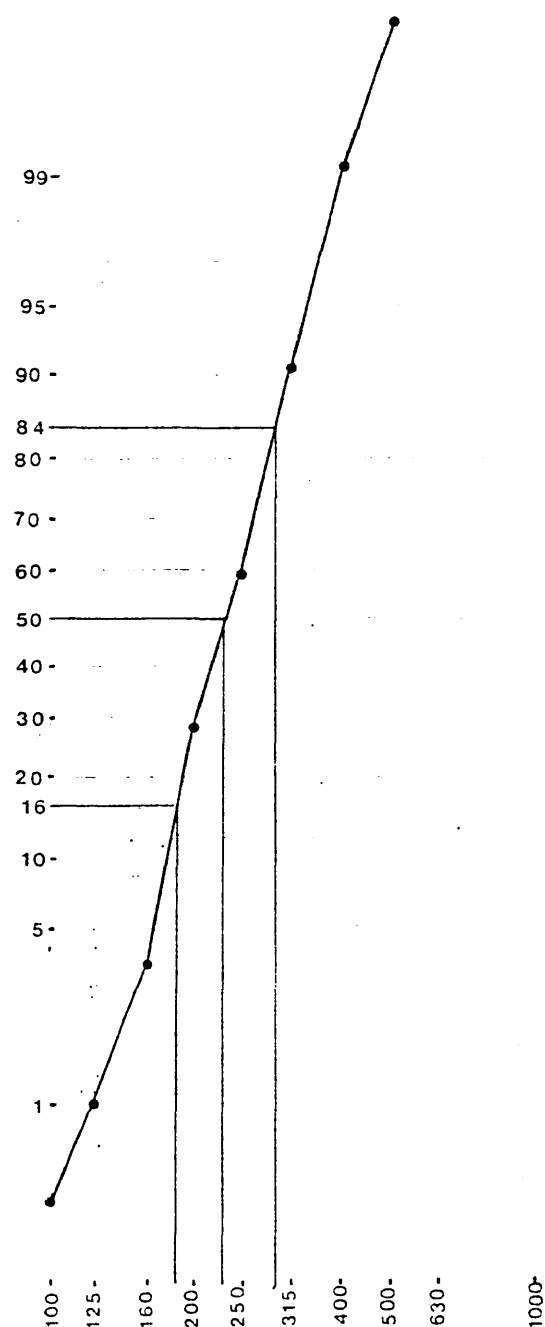
Figuur 4: Voorbeeld van een grafiek, zoals die gebruikt werd bij de bepaling van de mediane korrelgrootte en de sorteringfactor. Horizontaal de korrelgrootte ( \mu ) op een logaritmische schaal. Verticaal procenten van het totaalgewicht, cumulatief uitgezet. Snijpunt van de lijn met het 50%-niveau levert de mediane korrelgrootte op ( 230\mu ). De helft van het verschil tussen de korrelgroottes behorend bij 16 en 84%, uitgedrukt in \phi -notatie levert de sorteringfactor op.
