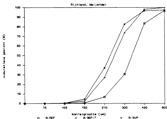
Figuur 7. Korrelgrootte-verdeling van zand van Rijnland, Meijendel:
