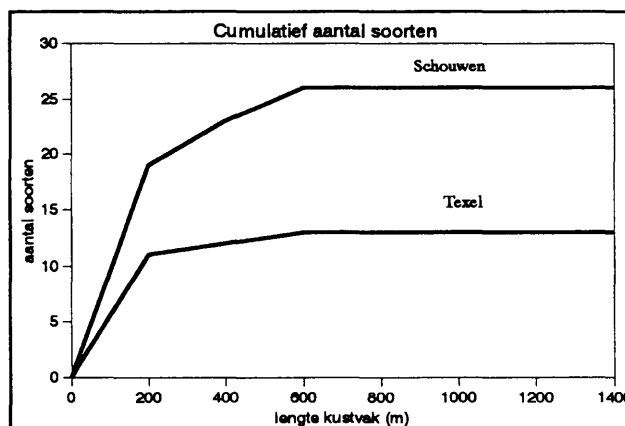
Figuur 23. Cumulatief aantal gevonden soorten in de zeereep per lengte van het opgenomen kustvak op de locaties Schouwen en Texel.
