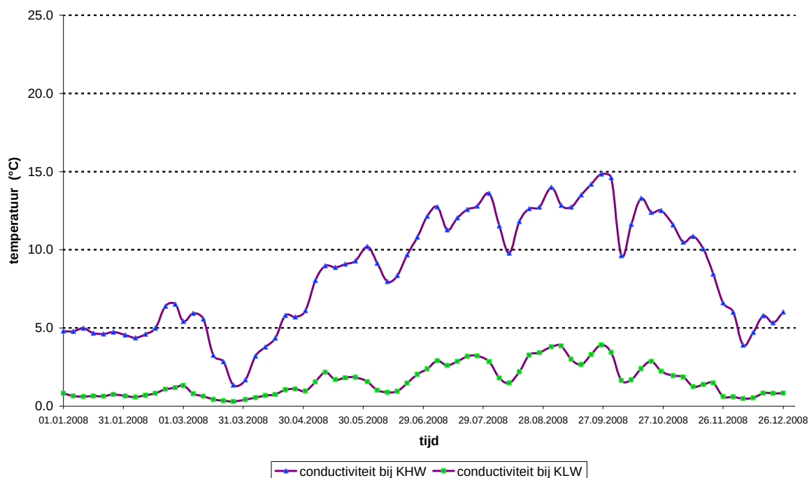
Figuur 68 - Beneden-Zeeschelde te Oosterweel: jaarverloop 2008 van de conductiviteit per vijfdaagse periode, met onderscheid naar de conductiviteit bij KHW en bij KLW
