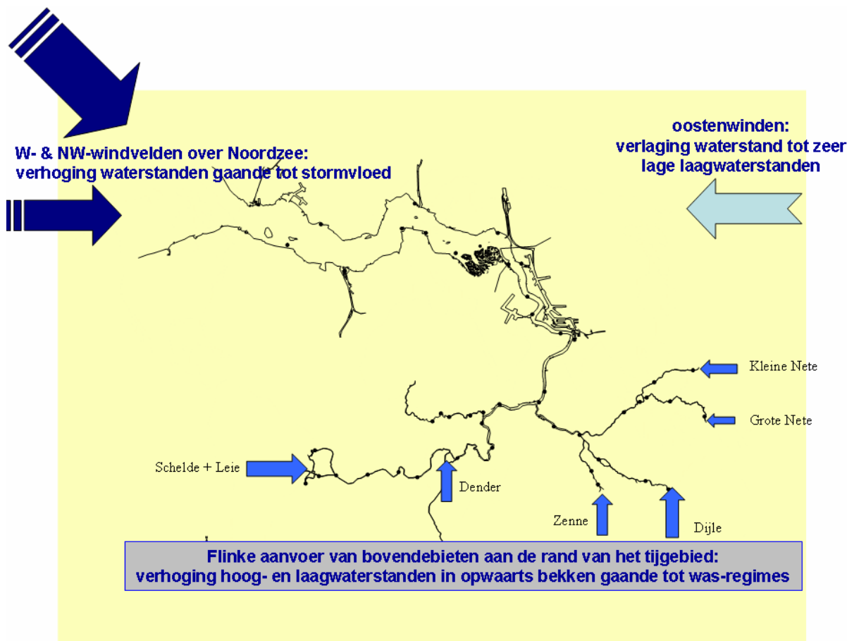
Figuur 1 - Zeescheldebekken: algemeen ligingsplan met schetsmatige aanduiding van de grootste tij-beïnvloedende componenten
