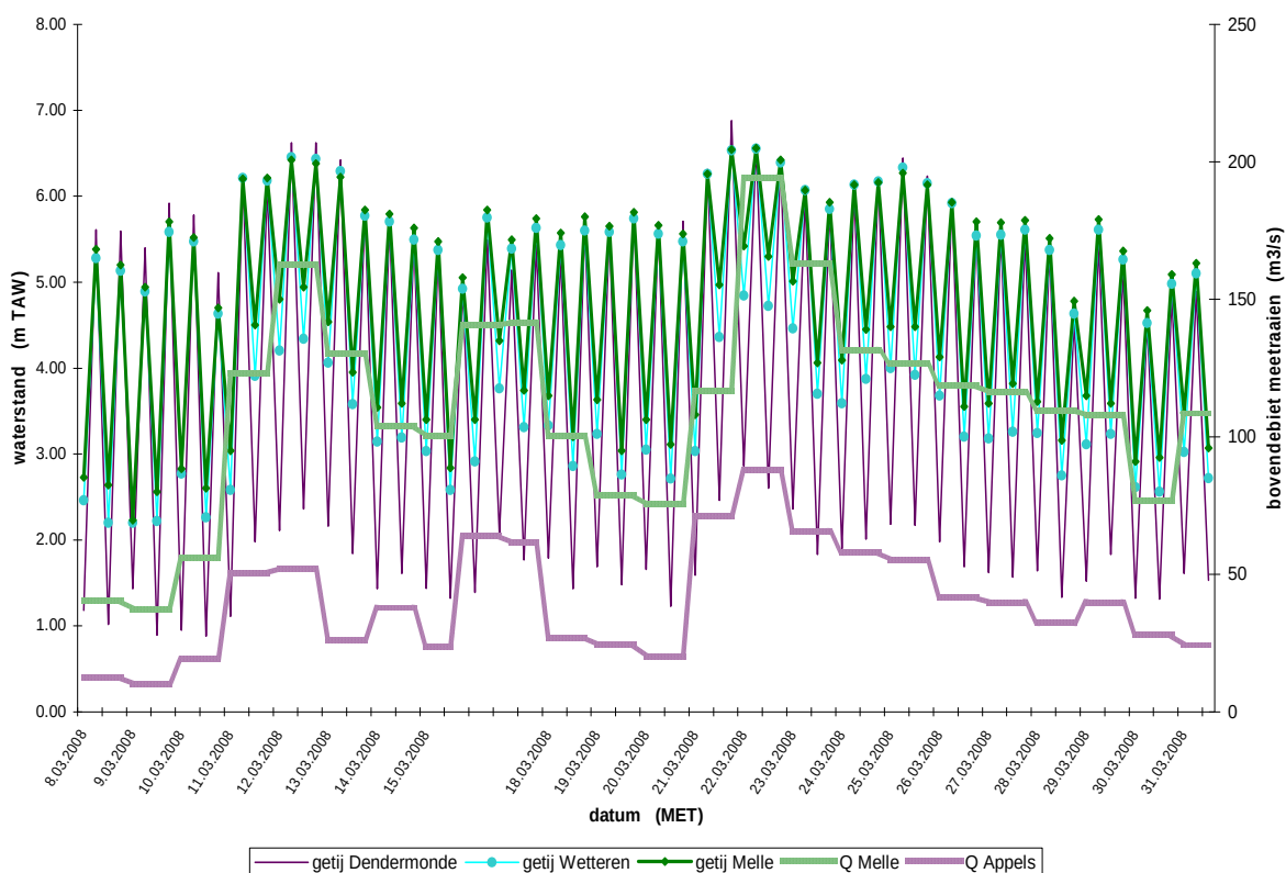
Figuur 33 - Zeeschelde en Dender: verloop van tij en bovendeibiet gedurende de was-periode van 11 à 31 maart 2008 (het tij is in meter T.A.W., de bovendeibieten zijn in m³/s)
