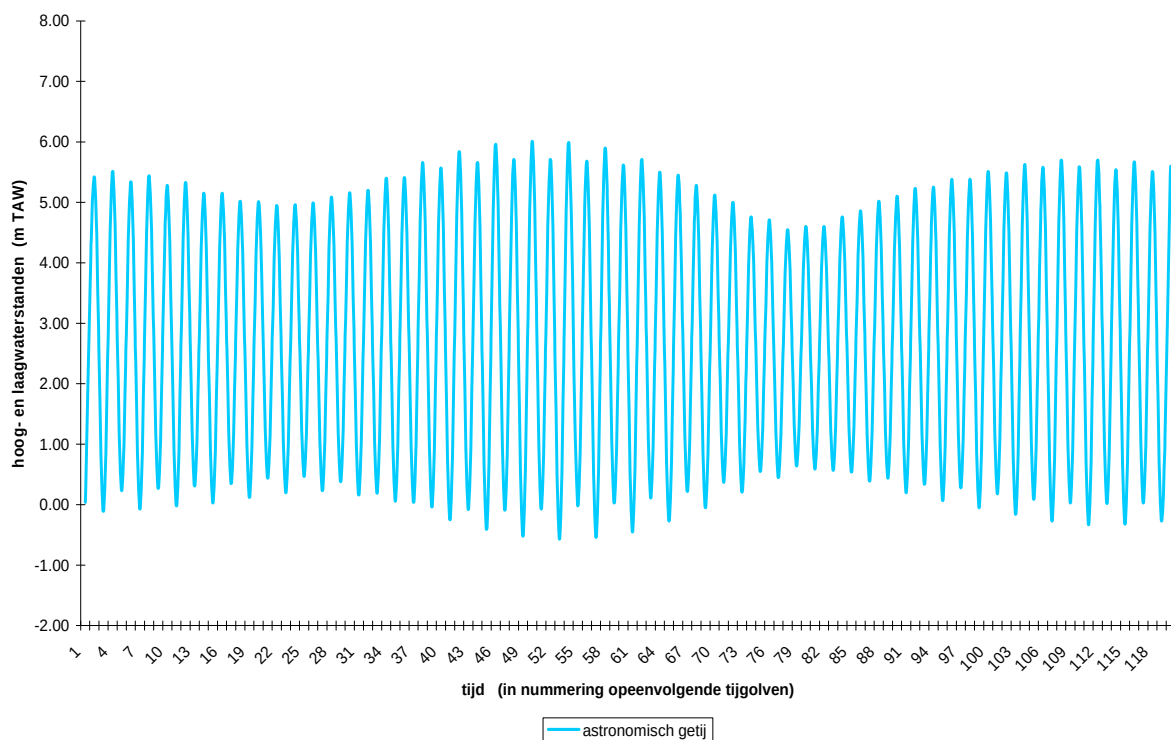
Beneden-Zeeschelde te Antwerpen-Loodsgebouw : vergelijking astronomisch voospeld en reëel waargenomen tij maand januari 2009
