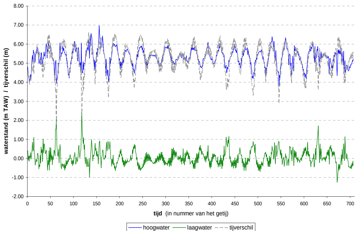
Figuur 13 - Beneden-Zeeschelde te Antwerpen-Loodsgebouw: jaarverloop van het tij gedurende het jaar 2008 door aanduiding van de afzonderlijke verlopen van hoogwater, laagwater en tijverschil
