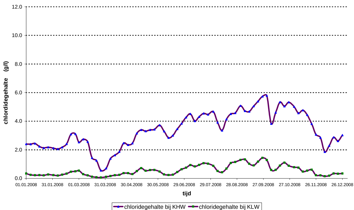
Figuur 69 - Beneden-Zeeschelde te Oosterweel: jaarverloop 2008 van het chloridegehalte per vijfdaagse periode, met onderscheid naar het chloridegehalte bij KHW en bij KWL
