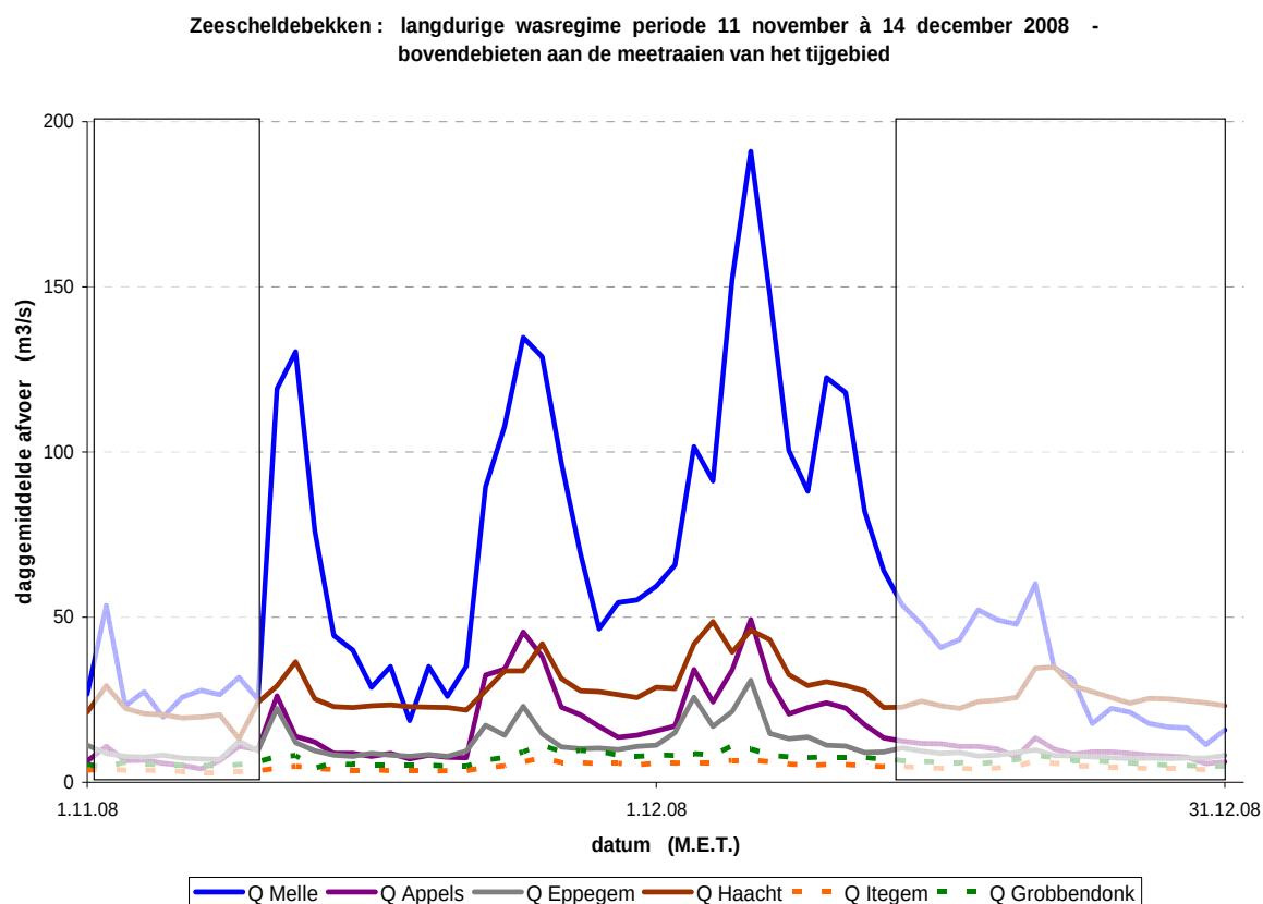
Figuur 37 - Zeescheldebekken: algemeen verloop van de bovendebieten aan de meetraaien gedurende de was-periode van 11 november à 14 december 2008 (alle bovendebieten zijn in m 3 /s)
