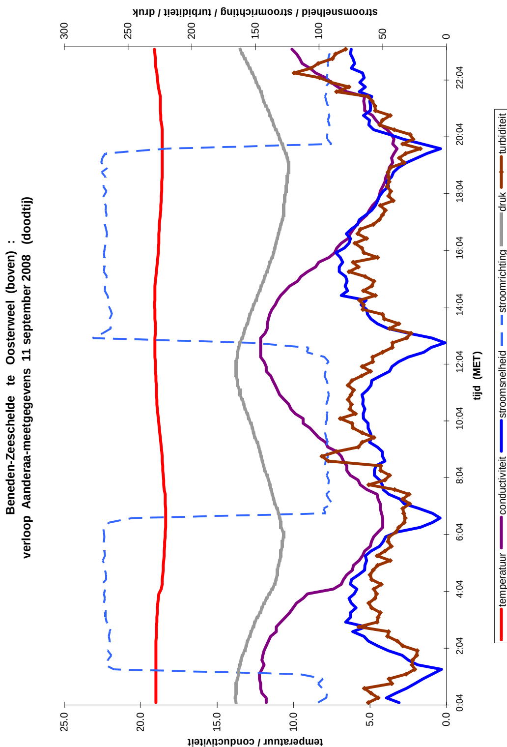
Figuur 59 - typisch verloop van de tienminuut-meetresultaten van Aanderaa-meettoestellen met name temperatuur, conductiviteit (bij heersende temperatuur), stroomsnelheid, stroomrichting, druk (zowel lucht- als waterdruk) en turbiditeit en zulks bij een doodtij (gedurende één etmaal)
