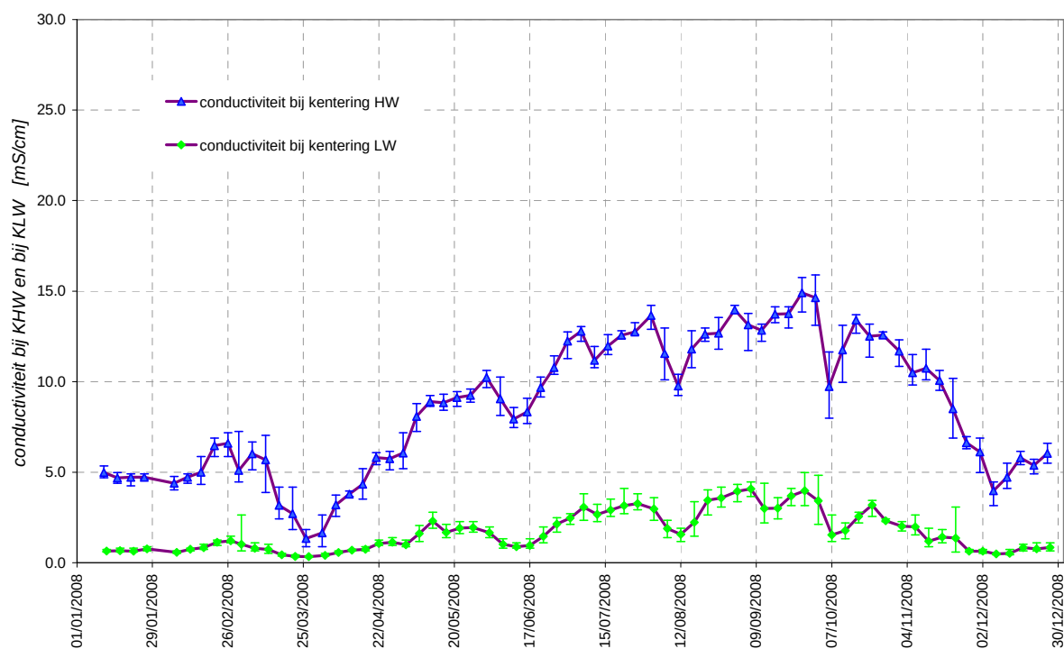
Figuur 84 - Beneden-Zeeschelde te Oosterweel: jaarverloop 2008 per vijfdaagse periode van de conductiviteit bij KHW en bij KLW (bovenste figuur gaat over het bovenste meettoestel, onderste figuur over het onderste)
