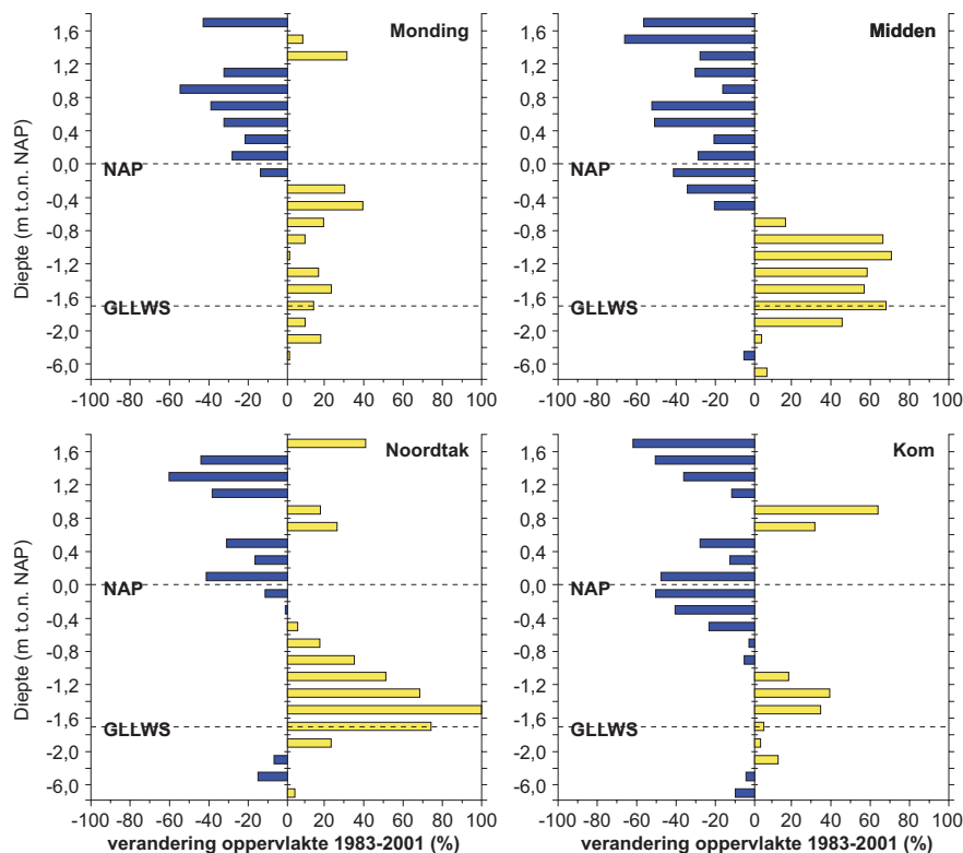
..... Figuur 6.5 Verandering van oppervlaktes intergetijdengebied en geulrand in dieptezones boven NAP –8 m voor de vier deelgebieden. Let op: tussen NAP –8 m en NAP –2 m de dieptezones 2 m diep zijn. Boven NAP –2 m zijn de dieptezones 0,2 m diep.
