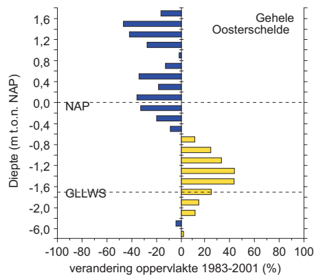
..... Figuur 6.4 Verandering van oppervlaktes intergetijdengebied en geulrand in dieptezones boven NAP –8 m in de Oosterschelde. Let op: tussen NAP –8 m en NAP –2 m de dieptezones 2 m diep zijn. Boven NAP –2 m zijn de dieptezones 0,2 m diep.
