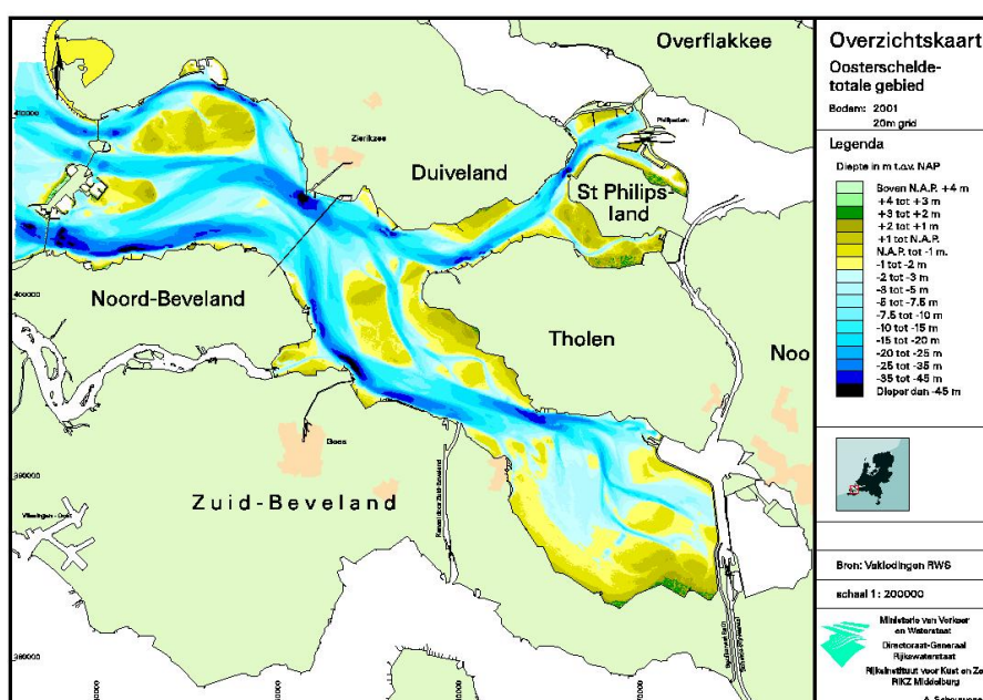
Figuur 6.1 Hoogte/ diepte kaart van de Oosterschelde in 2001.
