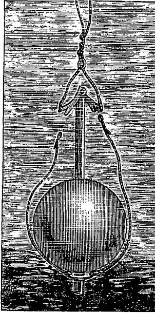
Fig. 5. — Sondeur de Brooke.
