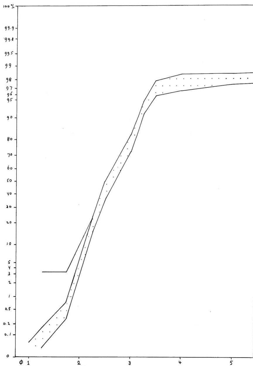
Fig. 6. Resultaat korrelgrootte-analyse P 77-3 zand.
