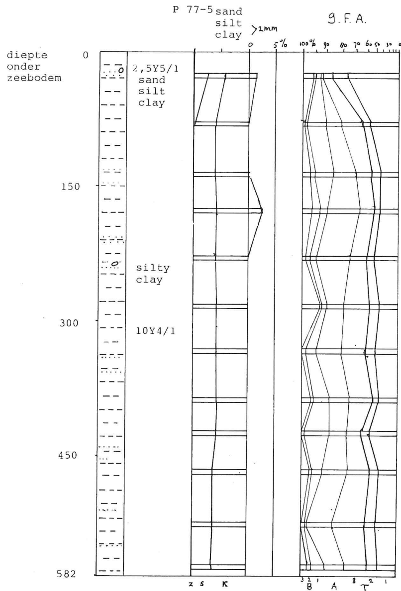
Fig. 8. Analyse kolom 4, P 77-5
