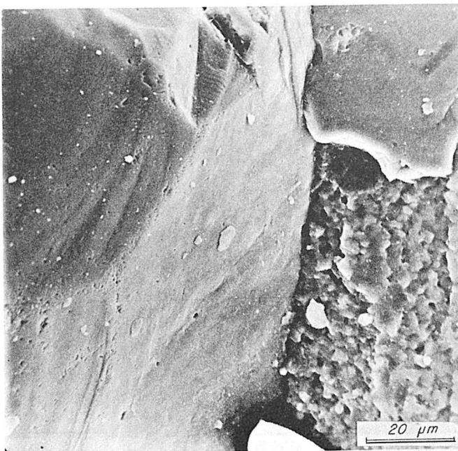
Plaat 3..Nieuwvorming van silikaatkristallen.
