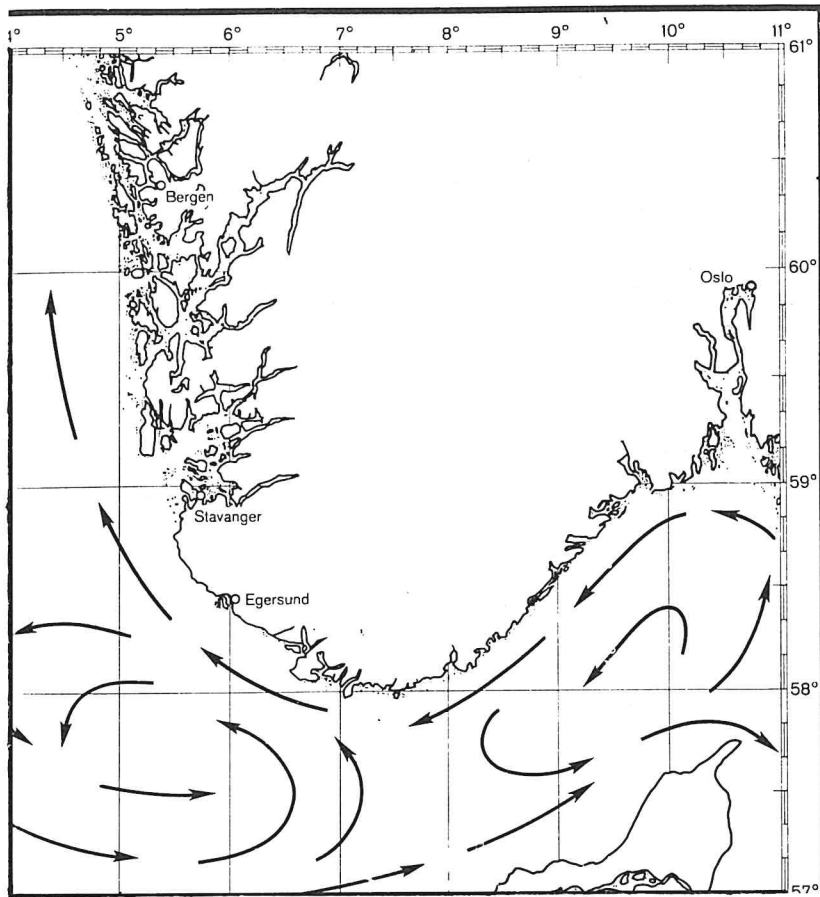
Fig. 2. Oppervlaktestrømmingen in het onderzochte gebied.
