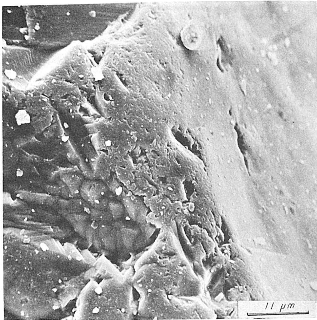
Plaat 2. V-vormige etsfiguren en nieuwvorming van silikaatkristallen.
