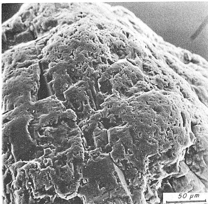
Plaat 5. Sterke chemische verwerking.
