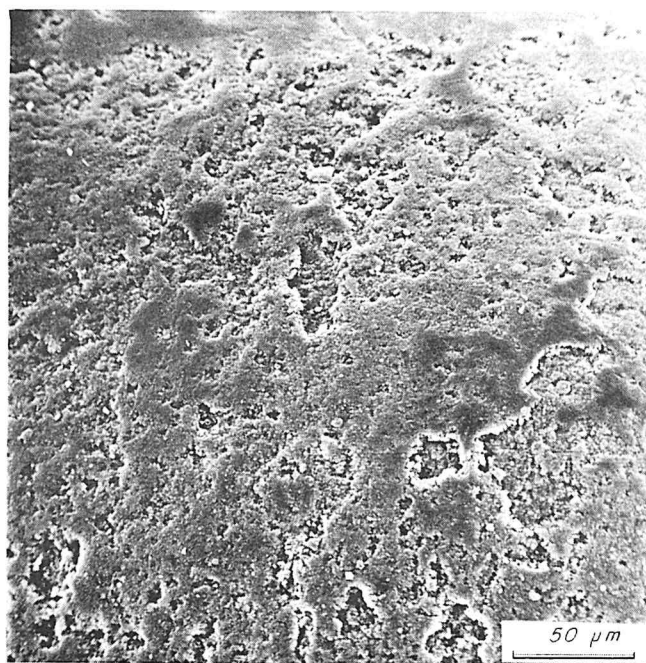
Plaat 1 (a en b). Kwartskorrel met ijzerhuidje.
