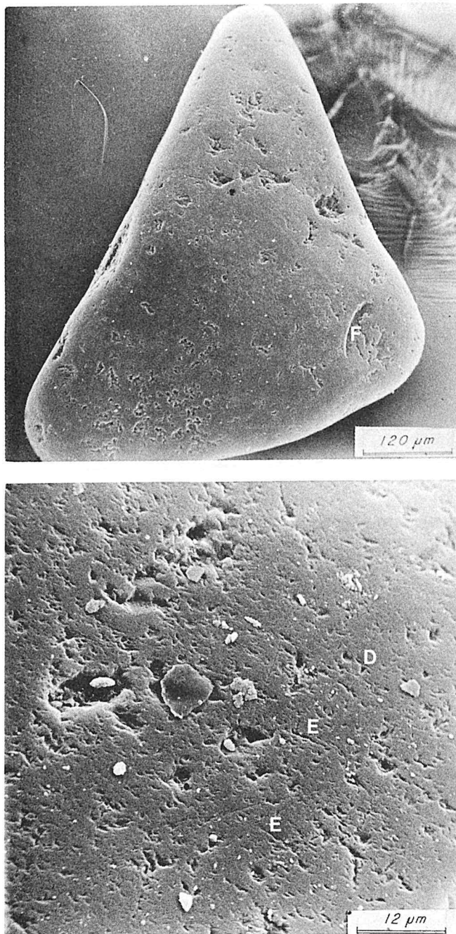
Plaat 9 (a en b). Ingespoeld kwartskorrel met glad korreloppervlak, afgeronde Korrelranden, V-vormige inkepingen (D), rechte of gebogen groeven (E) en boogvormige barsten (F). Op het korreloppervlak zijn verweerde striaties zichtbaar uit een eerder, vermoedelijk glaciaal stadium.
