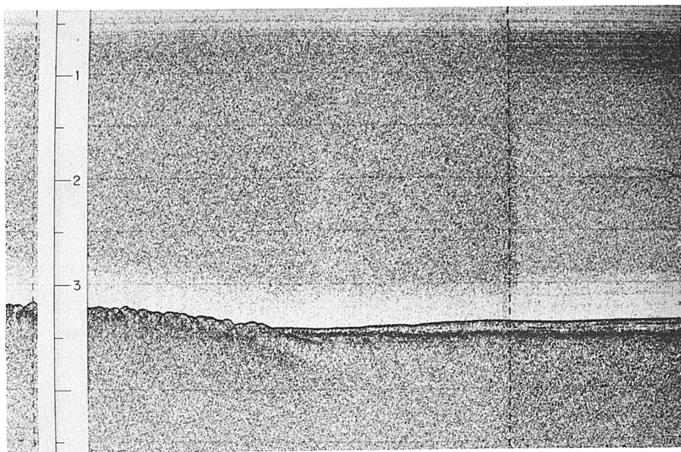
Fig. 3. Akoestisch profiel door de Noorse Geul.
