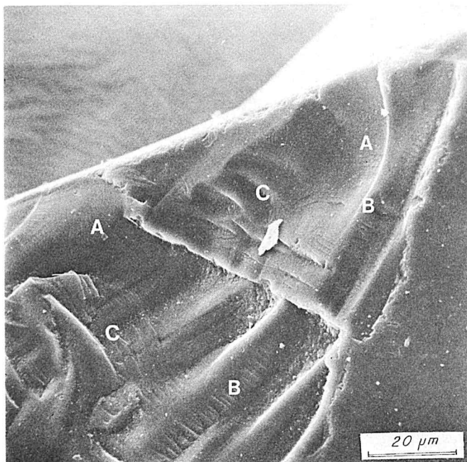
Plaat 7a. Als Plaat 6a, maar korrelranden enigszins afgerond door littorale abrasie. b. Detail.
