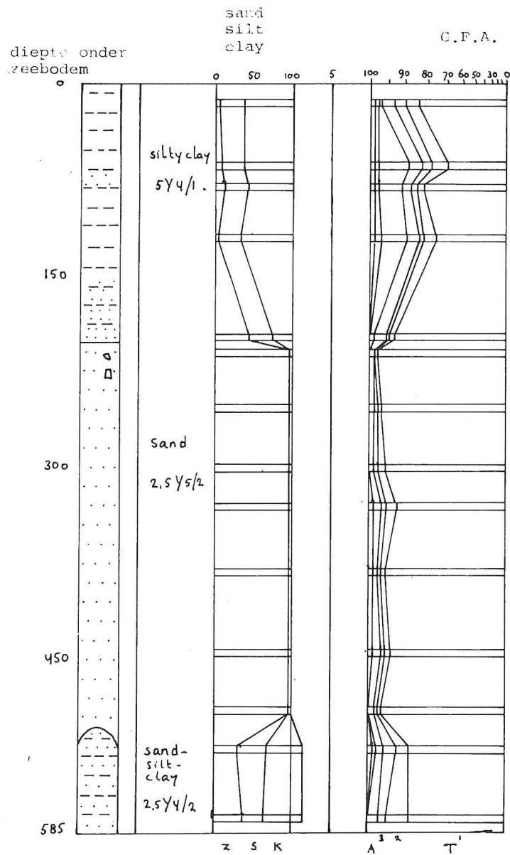
Fig. 5. Analyse kolom 2, P 77-3.
