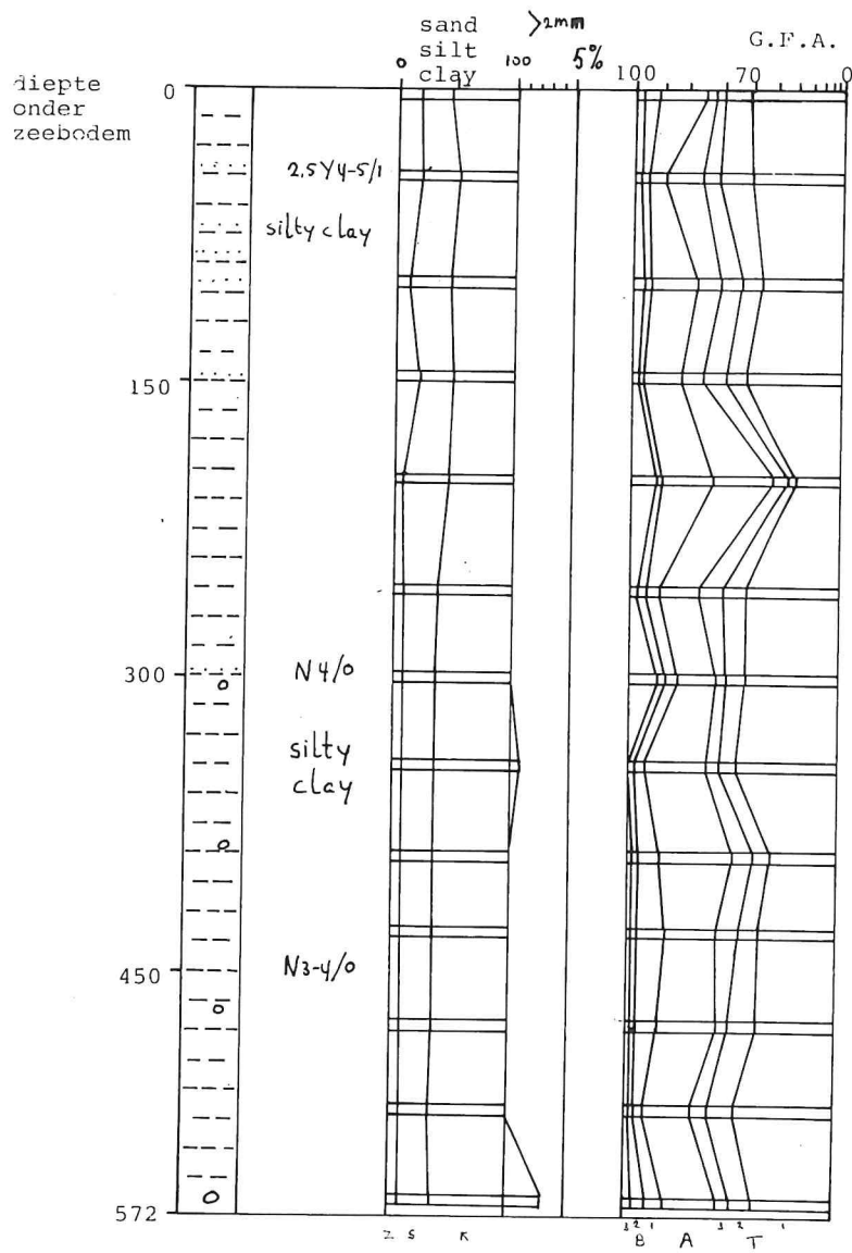
Fig. 4. Analyse kolom 1, P 77-1.
