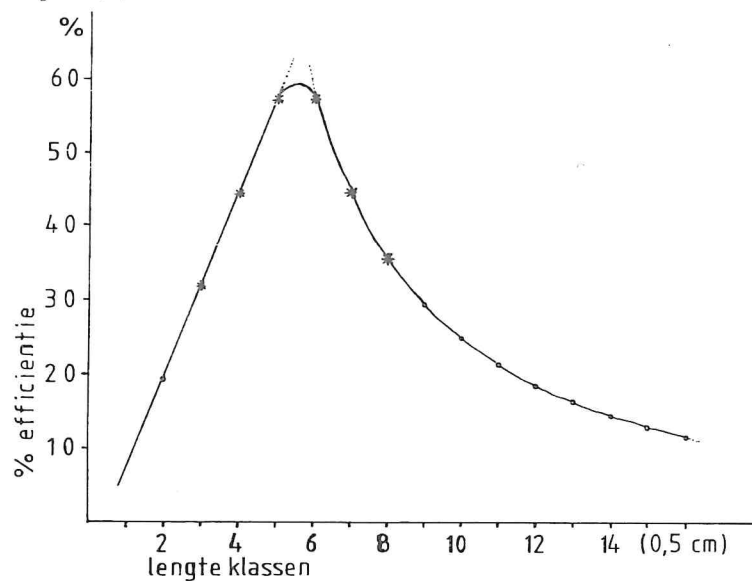
Fig. 2. De berekende % efficiëntie van het standaard boomkornet voor 5 mm lengteklassen van grondels. De gemiddelde lengte van de grondels in iedere klasse is (5 \times LK) + 2,5 mm.
