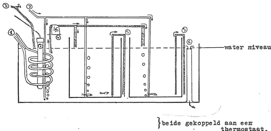
Fig. 25. P. microps . Opstelling voor de bepaling van de dagelijkse voedselopname van grondels in het laboratorium: 1. koelsysteem gevuld met methanol, 2. verwarmingselement, 3. zeewatertoevoer, 4. hevelpomp voor de watertoevoer naar de proefbakken, 5. afvoerhevel, 6. afvoer waarmee de waterhoogte ingesteld kan worden, 7. beluchting.
