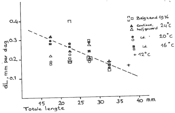
Fig. 29. P. microps . De lineaire relatie tussen de lengtegroei (mm/dag) en de lengte (5 mm klassen) van de grondels tijdens de groeiproeven.
