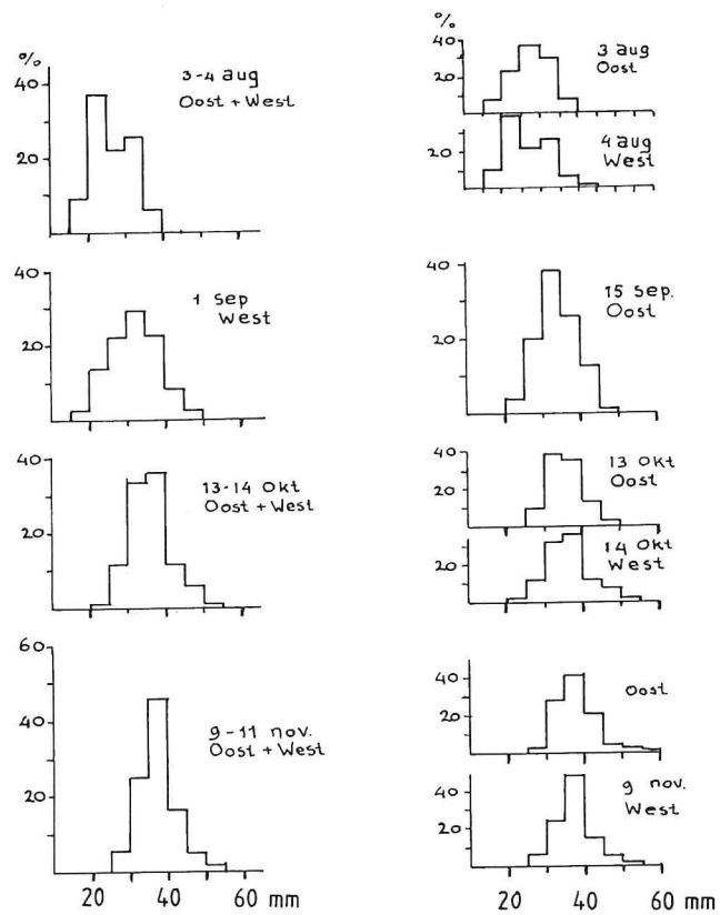
Fig. 6. P. microps . De lengteverdeling van de grondels op het Balgzand in 5 mm lengteklassen in 1976.
