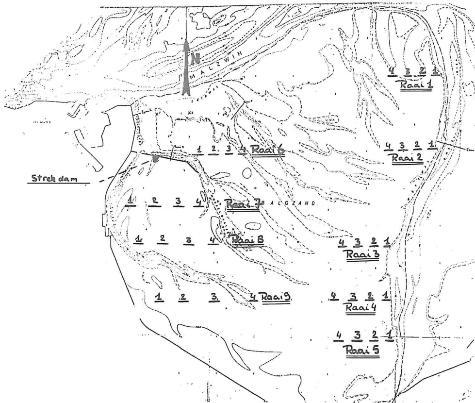
Fig. 3. Balgzand. Situering van de raaien en de stations waar gevist werd.
