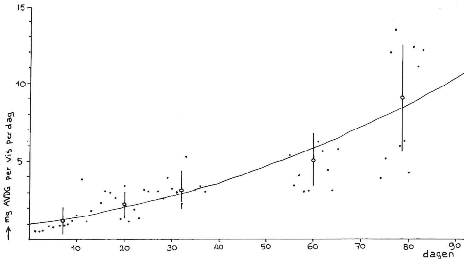
Fig. 31. P. microps . De dagelijkse voedselopname van de grondels (mg AVDG per vis, per dag) gemeten in het laboratorium bij 20°C. V_{20} = 0,00133 \cdot L^{2,474} ; n = 5 ; r = 0,991 .
