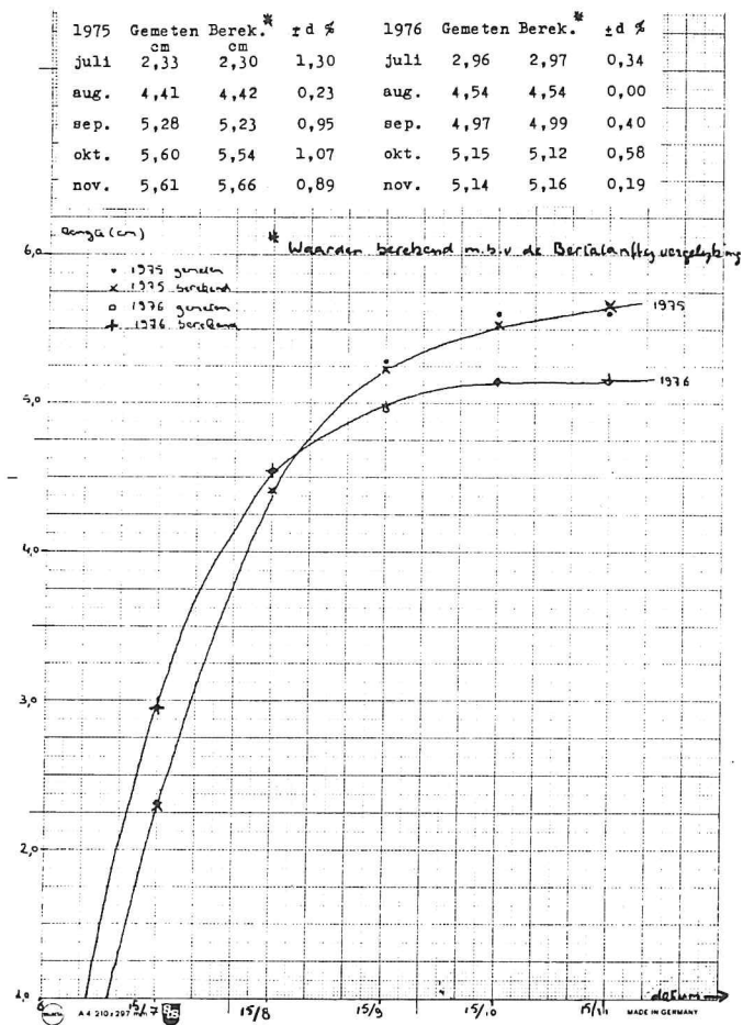
Fig. 15. P. minutus . Groei op het Balgzand. De maandelijkse gemeten gemiddelde lengte in cm voor 1975 (●●) en 1976 (oo), en de lengten berekend m.b.v. de Bertalanffy vergelijking voor 1975 (x) en 1976 (+).
