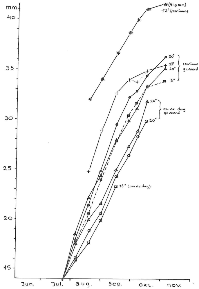
Fig. 28. P. microps . De lengtegroei (mm) in het laboratorium bij verschillende constante temperaturen en twee voedselregimes.
