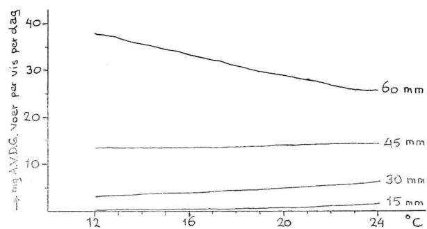
Fig. 34. P. microps . De invloed van de temperatuur op de dagelijkse voedselopname (V, mg AVDG/vis) berekend volgens de formule:
