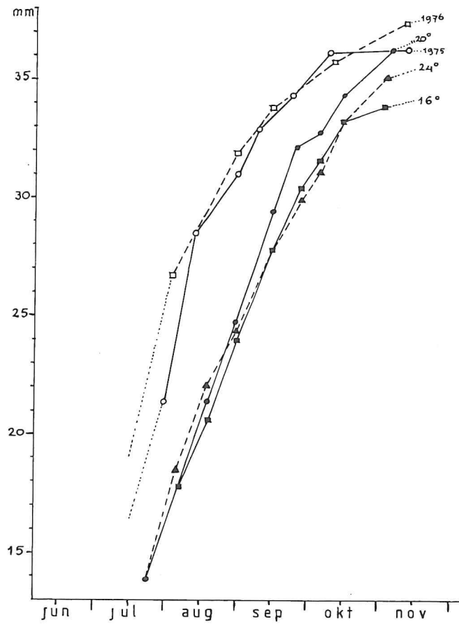
Fig. 10. P. microps . De groei in lengte (mm) van grondels op het Balgzand in 1975 (—) en 1976 (---) en in het laboratorium bij constante temperaturen van 16° (□), 20° (oo) en 24° (ΔΔ).
