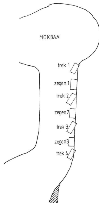
Fig. 1. Bepaling van de efficiency van het standaard boomkornet. De situering in de Mokbaai (Texel) van de trekken met het kornet (Tr) en met de zegen (Z).
