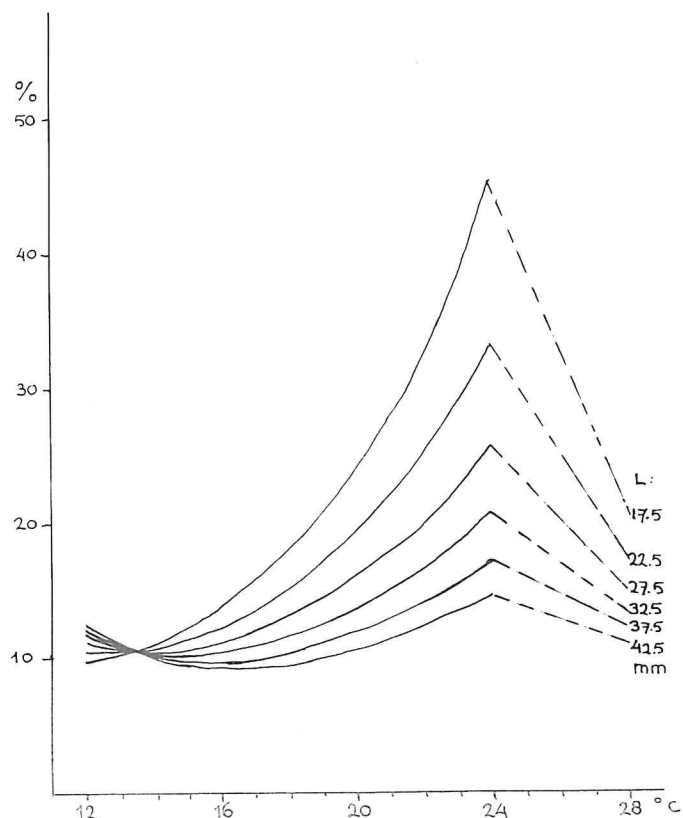
Fig. 33. P. microps . De invloed van de temperatuur op de dagelijkse voedselopname (AVDG) uitgedrukt als een percentage van het asvrij drooggewicht van de vis.
