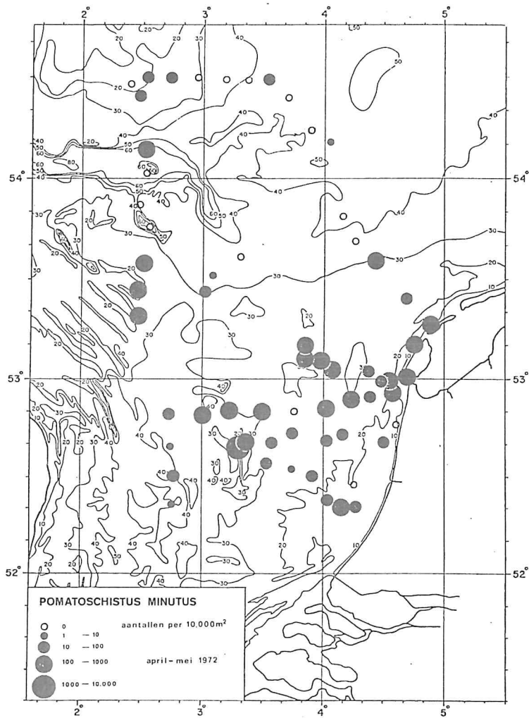
Fig. 20. P. minutus . De verspreiding van P. minutus in de Zuidelijke Noordzee. Gegevens van vaartochten met m.s. Aurelia in 1972.
