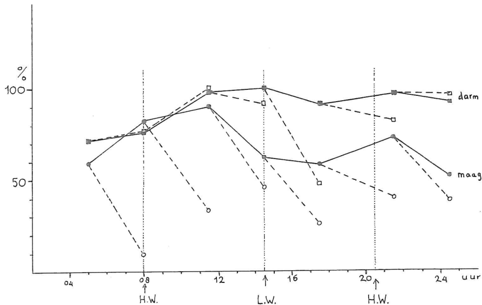
Fig. 22. P. microps . Resultaten van de Baikov serie op 25/9/76. Het percentage met gevulde magen (—●—) en met gevulde darmen (—■—) in relatie tot de tijd van monstername, direkt na vangst gemeten; tevens situatie 3 uur later (○ □). HW is hoogwater, LW is laagwater.
