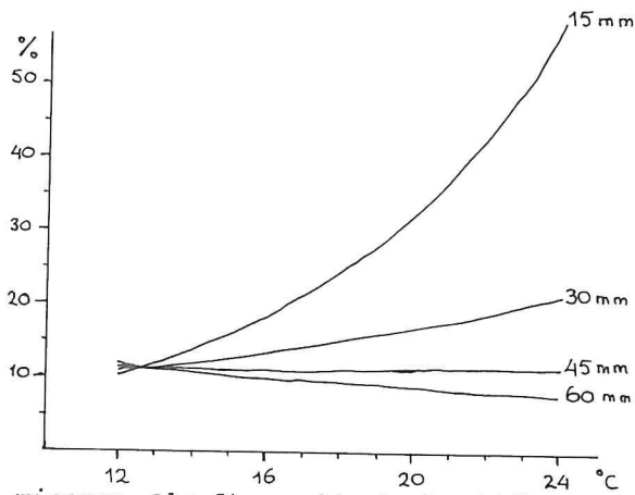
Fig. 35. P. microps . Als figuur 34, de dagelijkse voedselopname (AVDG) uitgedrukt als een percentage van het gewicht van de vis (AVDG).
