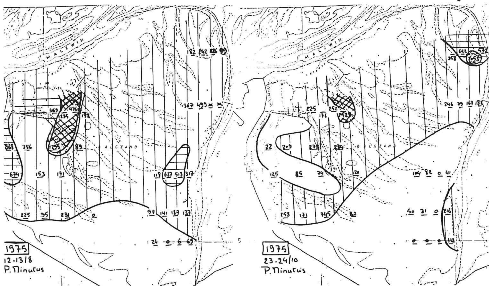
Fig. 13. P. minutus . Aantallen grondels per 1000 m 2 op het Balgzand in 1975.
