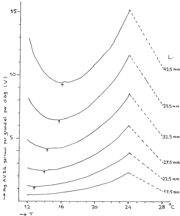
Fig. 32. P. microps . De invloed van de watertemperatuur ( T in °C) op de dagelijkse voedselopname ( V in AVDG) van de grondels in het laboratorium, in relatie tot hun lengte ( L in mm), voor de 5 mm klassen: V_{812-24^\circ\text{C}} = 7,2125 \times 10^{-5} \cdot T^{8,581} \cdot L^{25,806} T^{-0,7839} .
