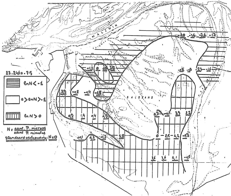
Fig. 18. Verspreiding van de verhouding (N) van de aantallen P. microps /aantallen P. minutus op het Balgzand in de periode 23/24-10-1975: \ln N < -1 (gearceerd); -1 < \ln N < 0 (wit) en 0 < \ln N (geblokt).
