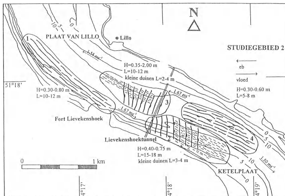
Figuur 5: Geomorfologische kaart van studiegebied 2, resulterend uit de side-scan sonarregistraties van 13/12/1995. De volle en onderbroken pijlen geven respectievelijk de vloed- en eb-stroom weer met vermelding van de maximum snelheid ( \text{ms}^{-1} ) in de bovenlaag (R. Codde & L. De Keyser, 1967). - Geomorphological map of study area 2, resulting from the side-scan sonar registrations of 13/12/1995. The full and dotted arrows represent the flood and ebb current, respectively, with the maximum current speed ( \text{ms}^{-1} ) in the upper layer (R. Codde & L. De Keyser, 1967).
