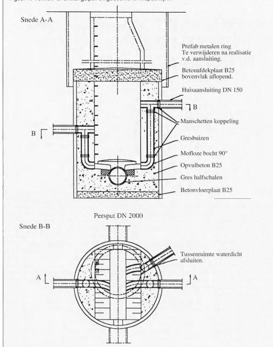
Figuur 1: Vertrek- of ontvangstput omgebouwd tot inspectieput.
