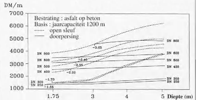
Grafiek 4: Kostenvergelijking, open sleuf - doorpersing, boven het grondwater met gresbuizen.
