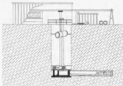
Figuur 5: Schilddoorpersing met hydraulisch transport.
