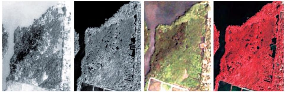
Door de beelden van 4 spectrale vensters te combineren komt men in de multispectrale remote sensing tot nauwkeurige waarnemingen van het bestudeerde oppervlak. Hier zien we eenzelfde stuk mangrovewoud in Pambala-Kakkapalliya (Sri Lanka) v.l.n.r. op een luchtfoto, op een panchromatisch beeld, op een ware kleurencompositie (blauw-groen-rood) en een valse kleurencompositie (blauw-groen-nabij-infrarood) met de IKONOS sensor (FDG)
