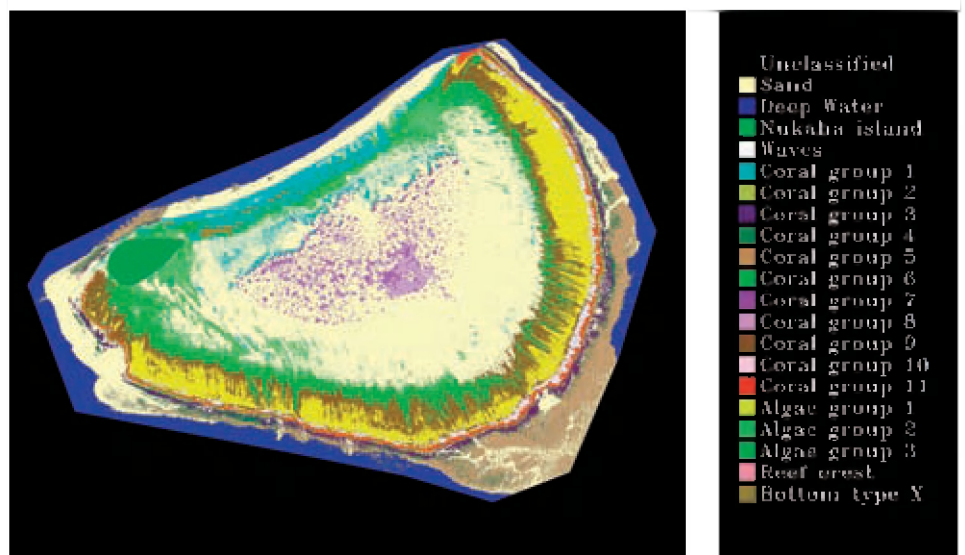
Classificatieresultaat (onder) van een hyperspectrale vliegtuigopname (boven rechts) van een atol (boven links) in Indonesië (regio Tanimbar - Fordate). Het hyperspectrale beeld laat toe de voornaamste koralengemeenschappen en sedimenttypen te onderscheiden (VITO)
