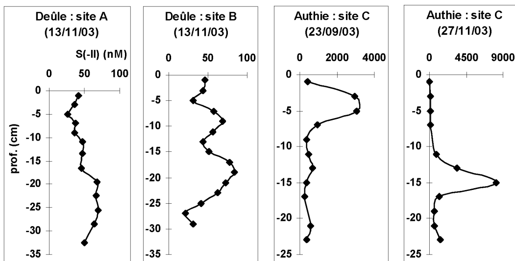
Figure/Figuur 3.5: Profils de concentration (nM) du soufre réduit dans les eaux interstitielles des carottes sédimentaires prélevées dans l'estuaire de l'Authie et le canal de la Deûle. (site A) : point de prélèvement situé en face du hangar de l'usine Métaleurop ; Deûle (site B) : point de prélèvement situé en amont (environ 300 m) de l'usine Métaleurop ; Authie (site C) : point de prélèvement situé sur la vasière nord de l'estuaire de l'Authie (salinité : 20 psu).
