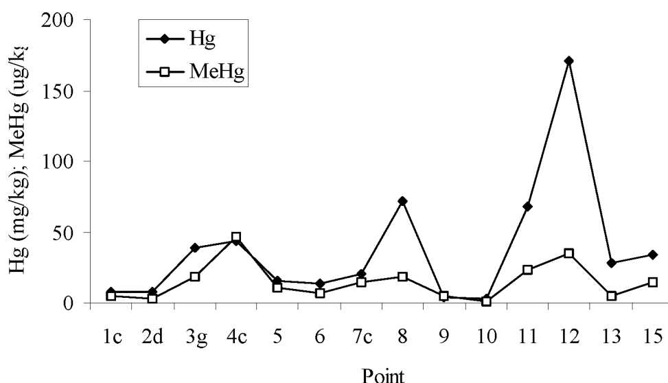
Figure/Figuur 8.3 : Concentration du mercure et du méthylmercure dans des sédiments de surface de la Deule Concentratie van kwik en methylmercure in de oppervlakesedimenten van de Deule
