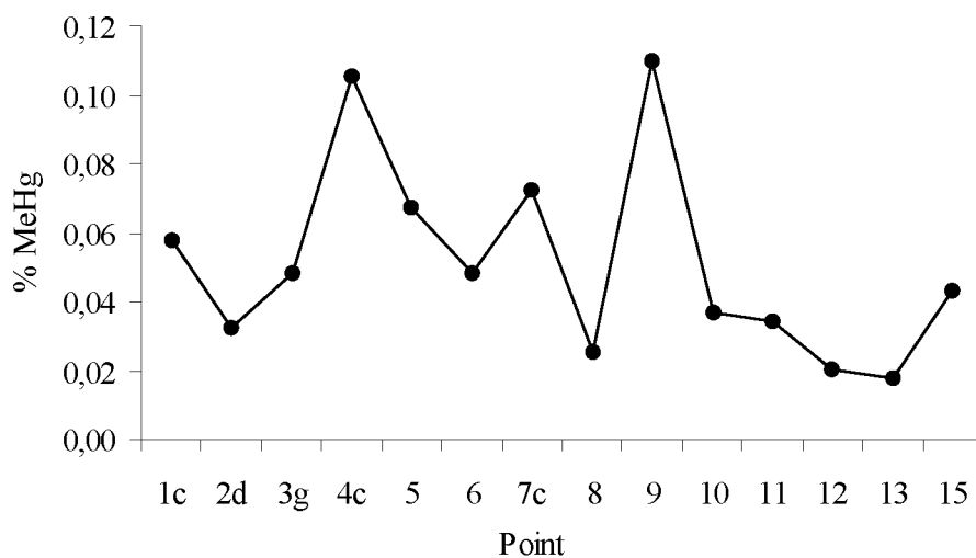
Figure/Figuur 8.4 : Percentage de methylmercure dans des sediments de surface de la Deule Percentage methylmercure in de oppervlaktesedimenten van de Deule
