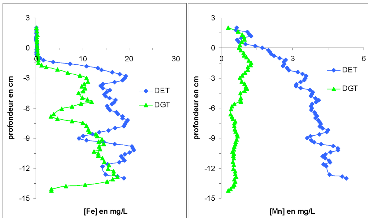
Figure / Figuur 3.2. Comparaison des teneurs en fer et manganèse dissous mesurées par les techniques DGT et DET en fonction de la profondeur d'un sédiment reconstitué.. Vergelijking van de gehalten aan opgelost ijzer en mangaan gemeten met de DGT en DET technieken in functie van de diepte van een hersamengesteld sediment.
