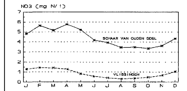
Afbeelding 14 Seizoenvariatie nitraat 1985-1992.
