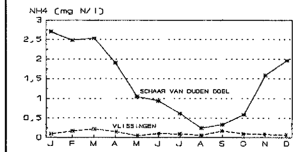
Afbeelding 15 Seizoenvariatie ammonium 1985-1992.
