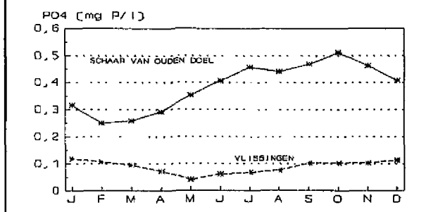
Afbeelding 16 Seizoenvariatie ortho-fosfaat 1985-1992.
