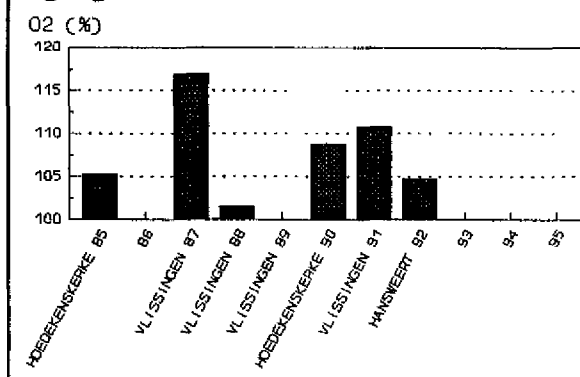
Afbeelding 12 Maximale zuurstofverzadiging.
