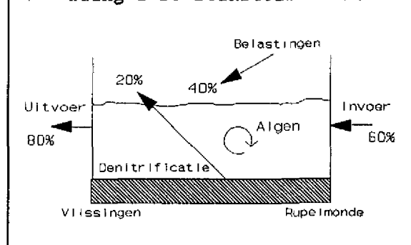
Afbeelding 2 De stikstofbalans.
