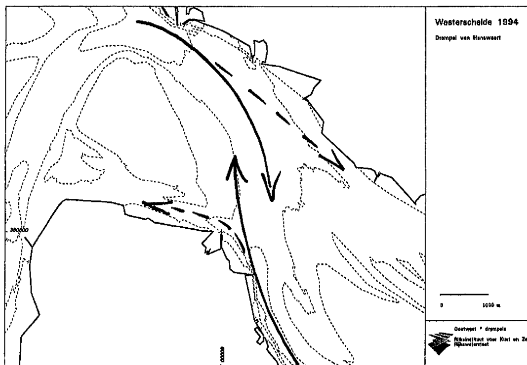
Figuur 3.3 Overgang van een 'botsende ebgeul'-type drempel (1931) naar een 'ontwikkende geulen'-type drempel (1994). Drempel van Hansweert
