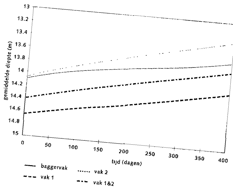
Figuur 4.10 Bodemontwikkeling in baggervak en drempelvak (vak 1 en 2) na correctie voor baggerwerk
