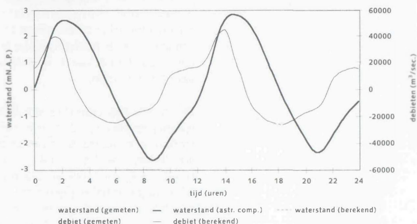
Figuur 4.2 Gemeten en berekende waterstand en debiet bij de Drempel van Hansweert.
