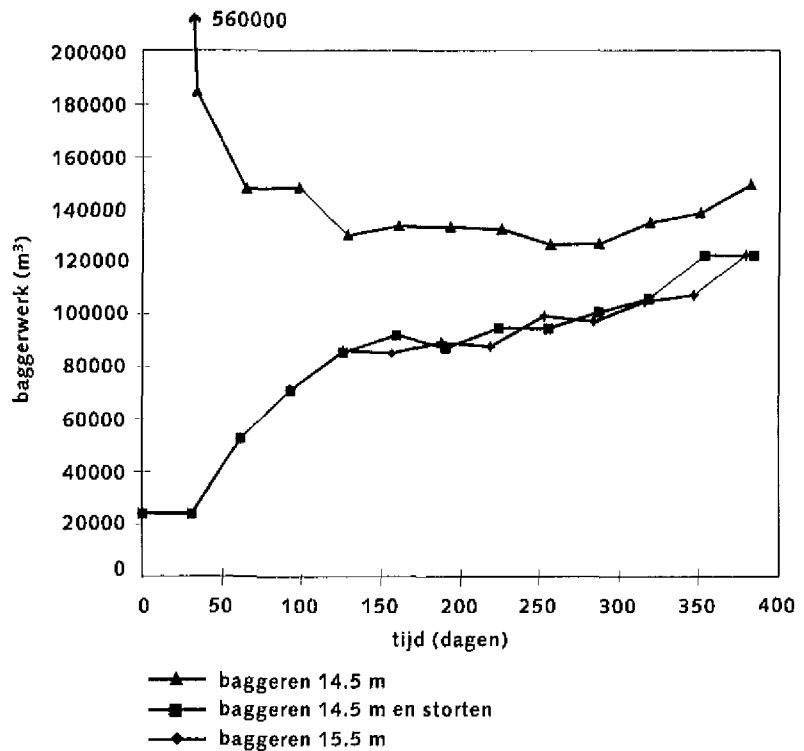
Figuur 5.4 Omvang van het baggerwerk als enkel de vaargeul gebaggerd wordt.
