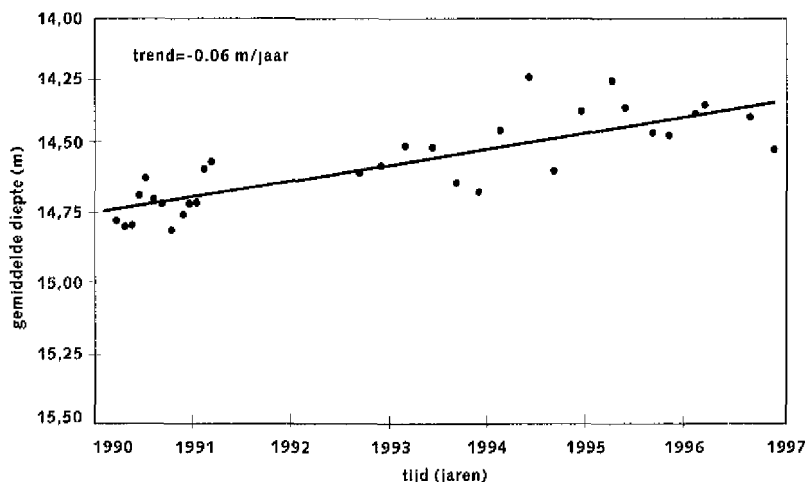
Figuur 4.5 Bodemligging op basis van lodingen van het baggervak
