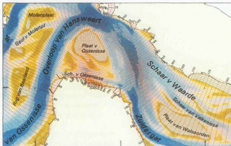
Figuur 4.1 Rooster van het DELFT2D-MOR model rond de Drempel van Hansweert.
