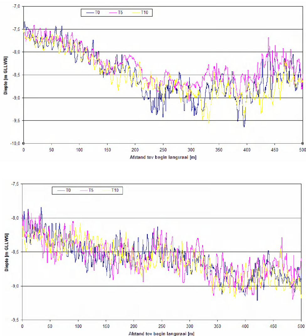
Figuur 13 - Evolutie profiel langsraai 1 (boven) en langsraai 2 (onder)
