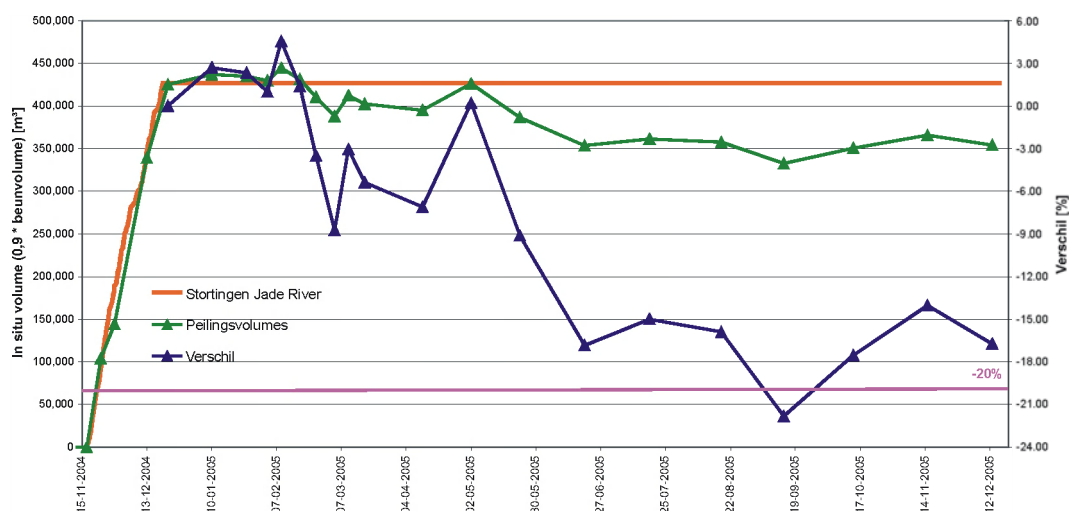
Figuur 10 - Volumeberekening op basis van multibeam peilingen
