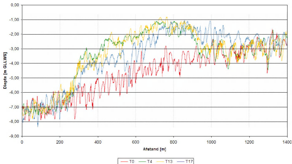
Figuur 11 - Evolutie profiel langsraai door de stortzone
