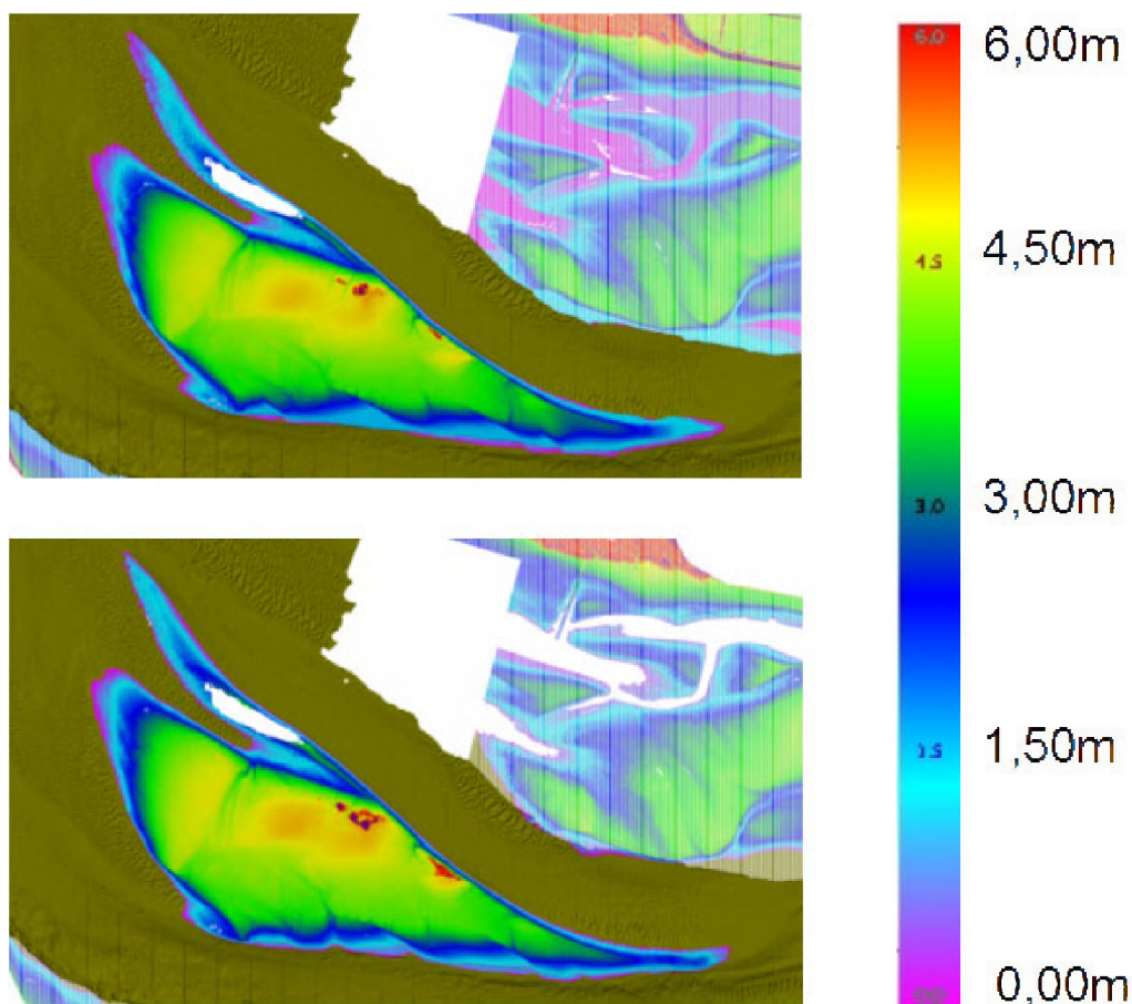
Figuur 14 - LIDAR opname plaat van Walsoorden (boven: november '04, onder: oktober '05). Verticale schaal: m boven GLLWS
