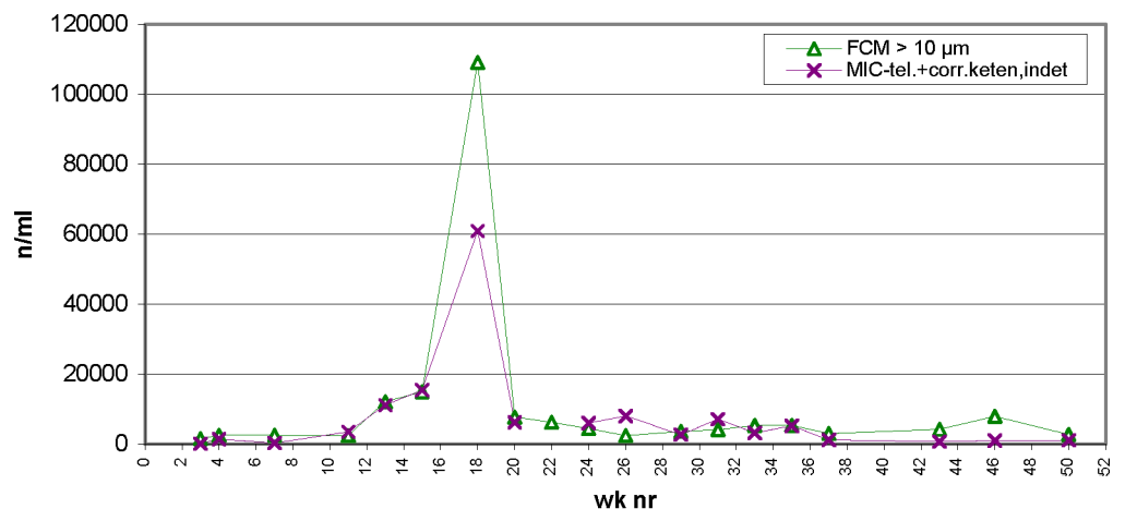
Figuur 4.3.3 Noordwijk 2: 2001 Microscooptellingen op lugol-gefixeerde monsters gecorrigeerd voor ketens en onbepaalde algen(paars) versus flowcytometertellingen van autotrofe deeltjes van 10 µm en hoger (groen)
