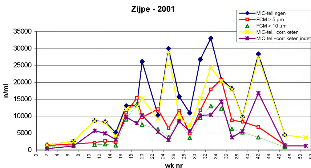
Figuur 4.3.4 Zijpe: 2001 Microscopietellingen op lugol-gefixeerde monsters gecorrigeerd voor ketens en onbepaalde algen (paars) versus flowcytometertellingen van autotrofe deeltjes van 10 µm en hoger (groen)
